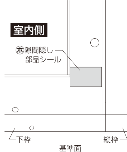
〔下部詳細図〕
