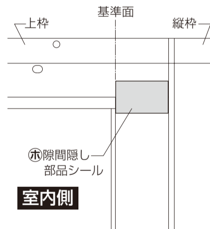
〔上部詳細図〕
