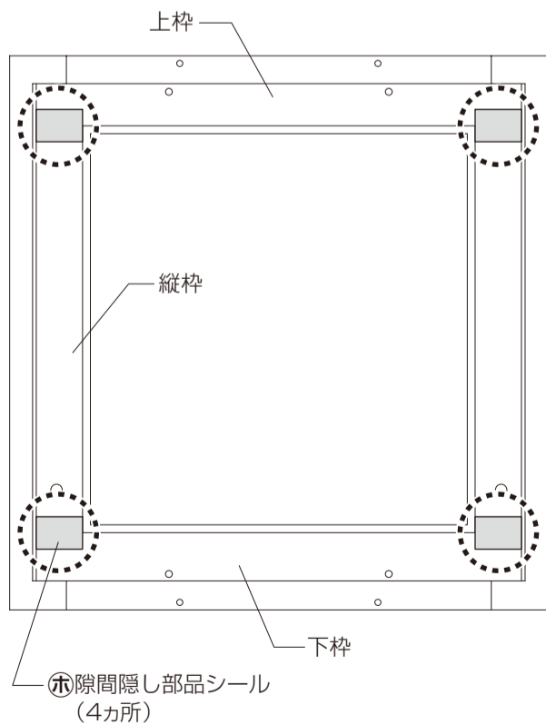
〔下部詳細図〕
