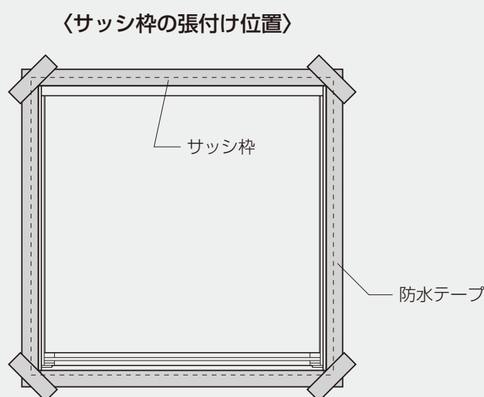
〔防水テープ張付け位置〕
