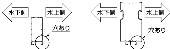
図5-1 W30・W52・W57
