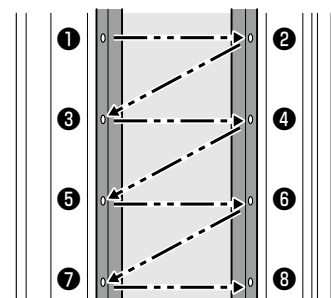
図7-2 ネジ固定順序
