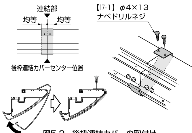
図5-2 後枠連結カバーの取付け
