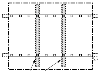
図3-1 前後枠ひっかけ用の中間アーチ取付位置
