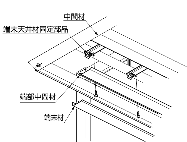
図1-2 天井材を側枠まで取付けない場合
