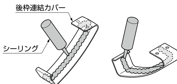
図5-1 後枠連結カバーのシーリング
