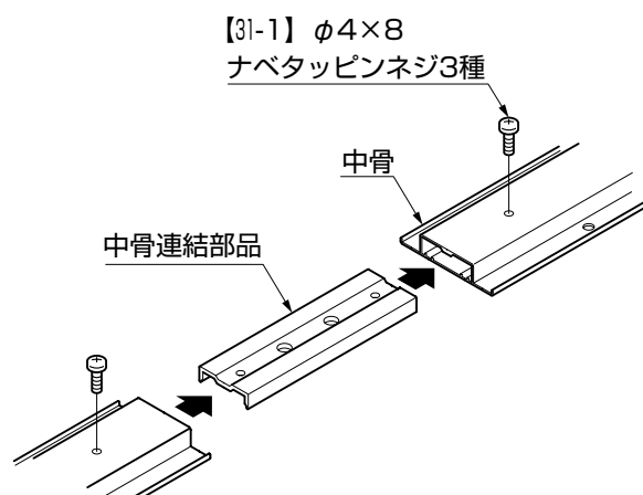
図1-3 A部詳細図 中骨を連結する場合 (2スパン、4スパン、5スパンの場合)
