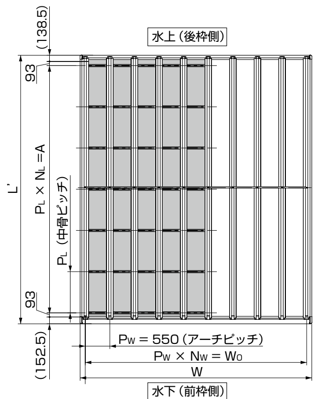
図2-3 5スパン
