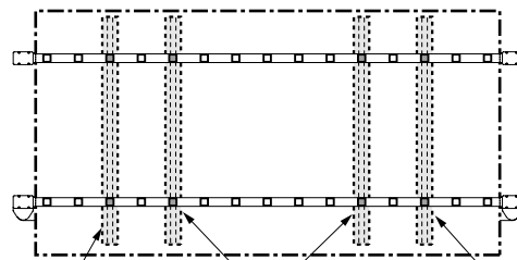
図3-1 前後枠ひっかけ用の中間アーチ取付位置
