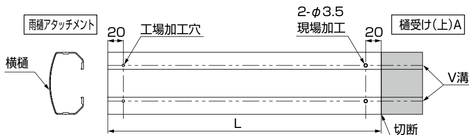
図1-3 加工図
