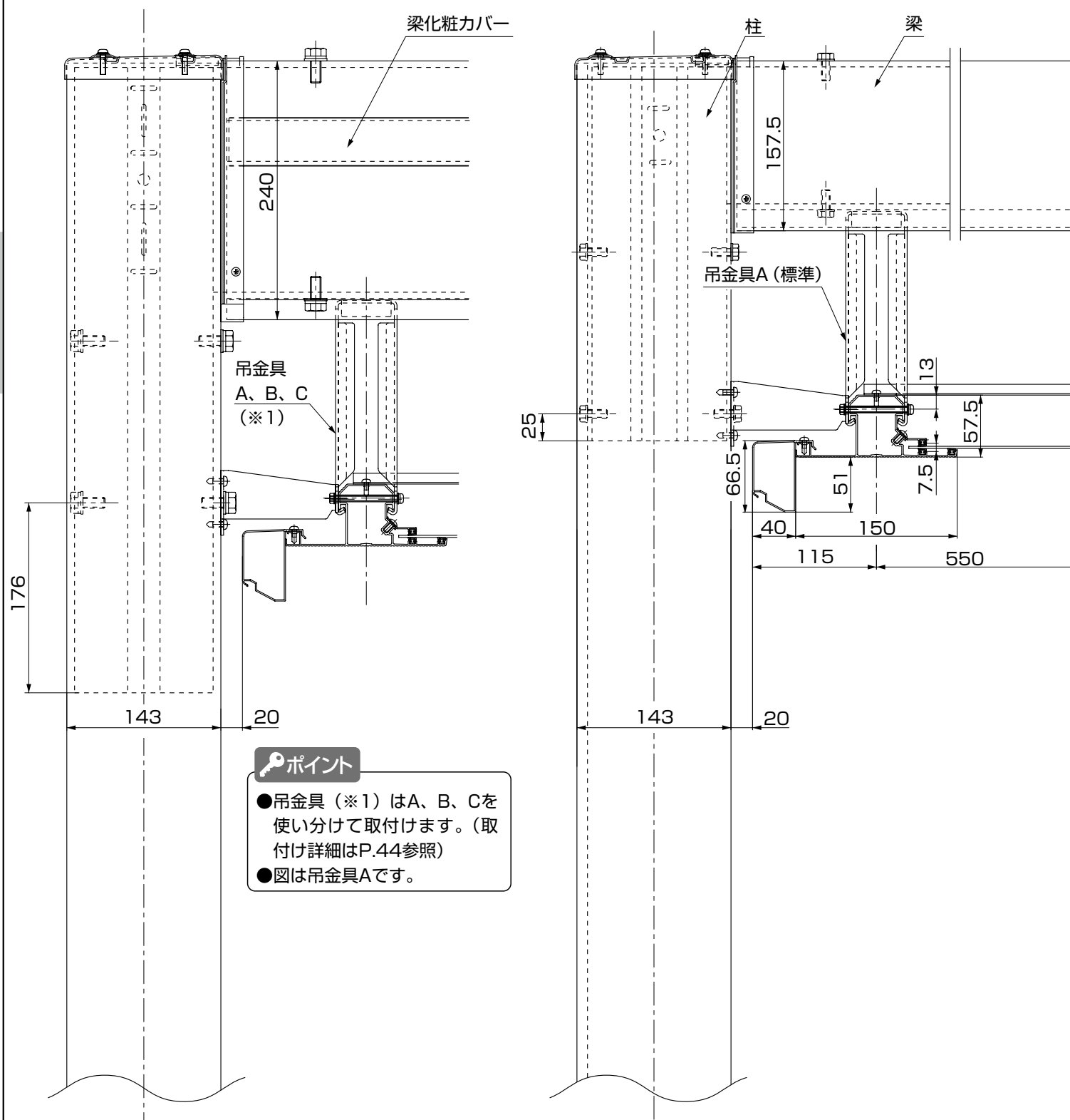
図2-1 W79・W90
