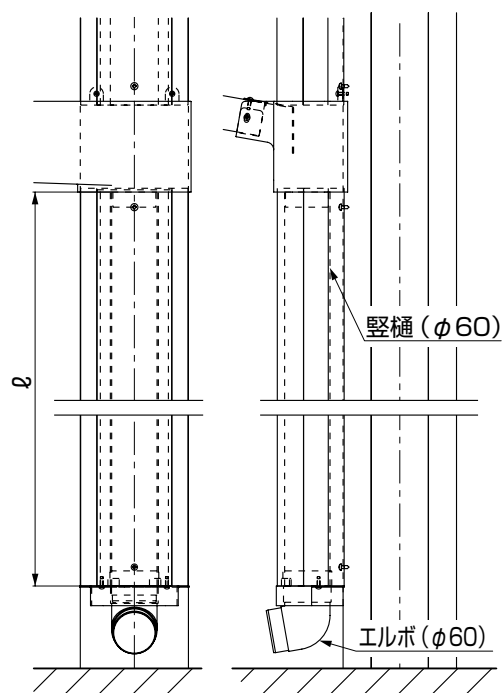
図3-3 W79・W90
