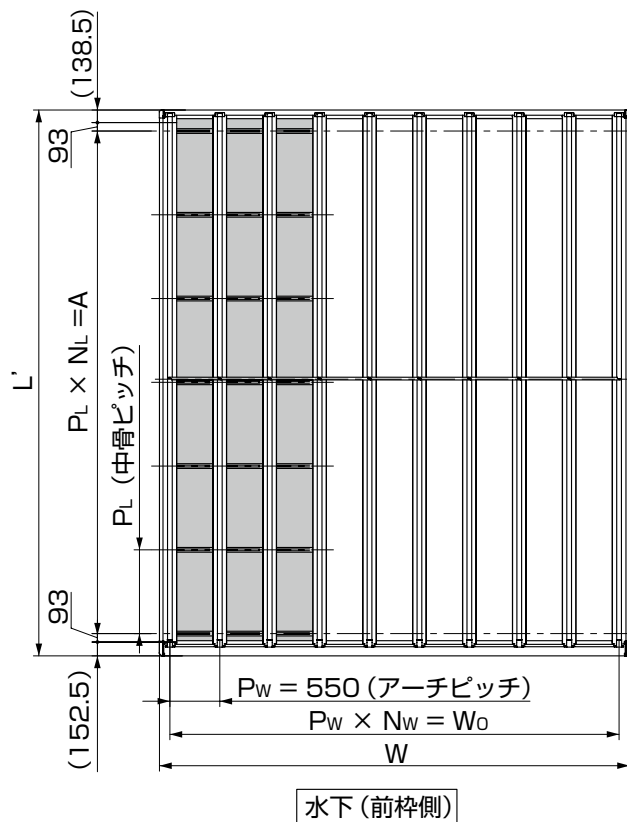
図2-2 3スパン
