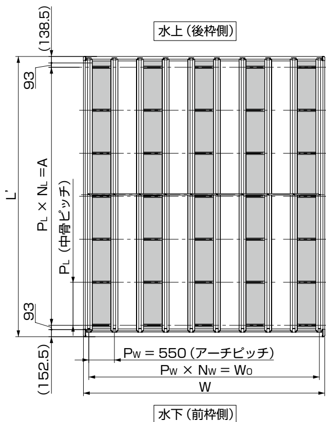
図2-1 1スパン (ゼブラ)
