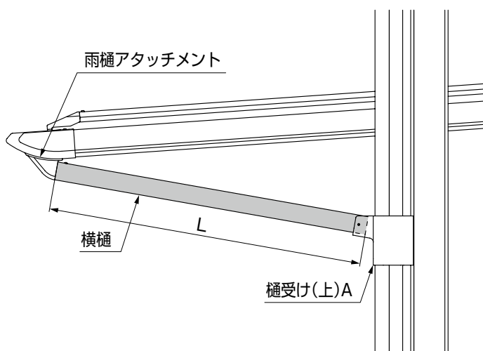
図1-3 加工図
