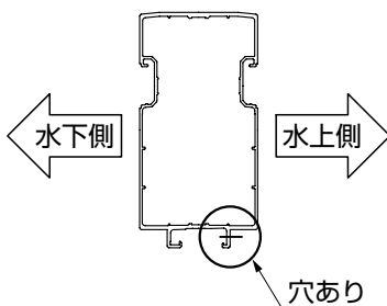
図4-2 W79・W90
