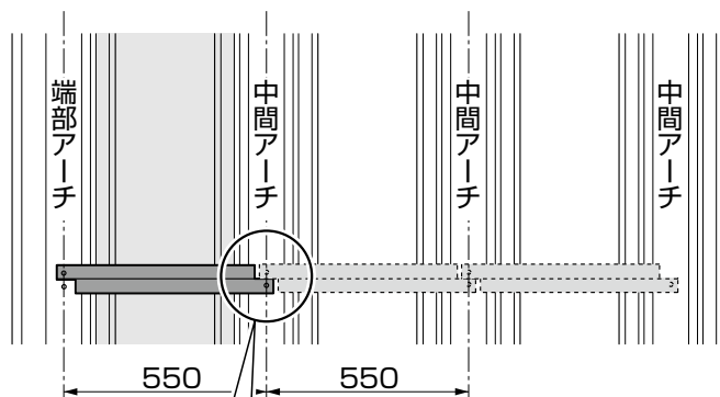
図7-1 上面図
