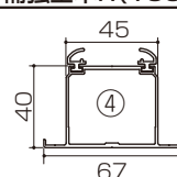
補強垂木R(1500)
