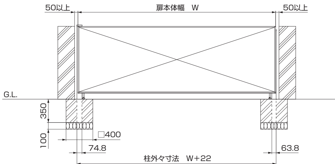
図2-2 正面図
