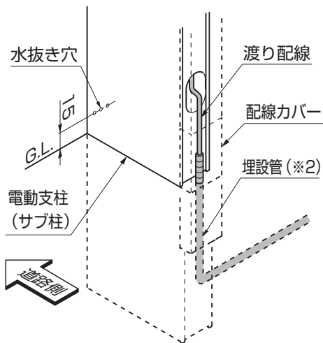
電動支柱の場合
