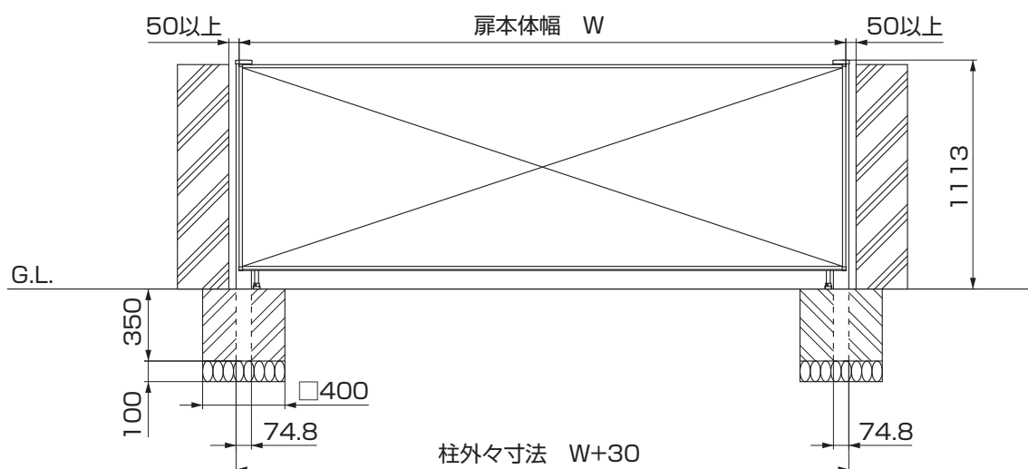
図2-10 正面図
