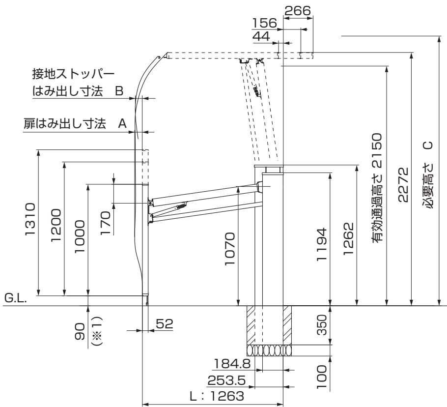
図2-4 側面図（ハイルーフの場合）
