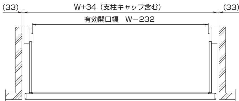
図2-9 平面図
