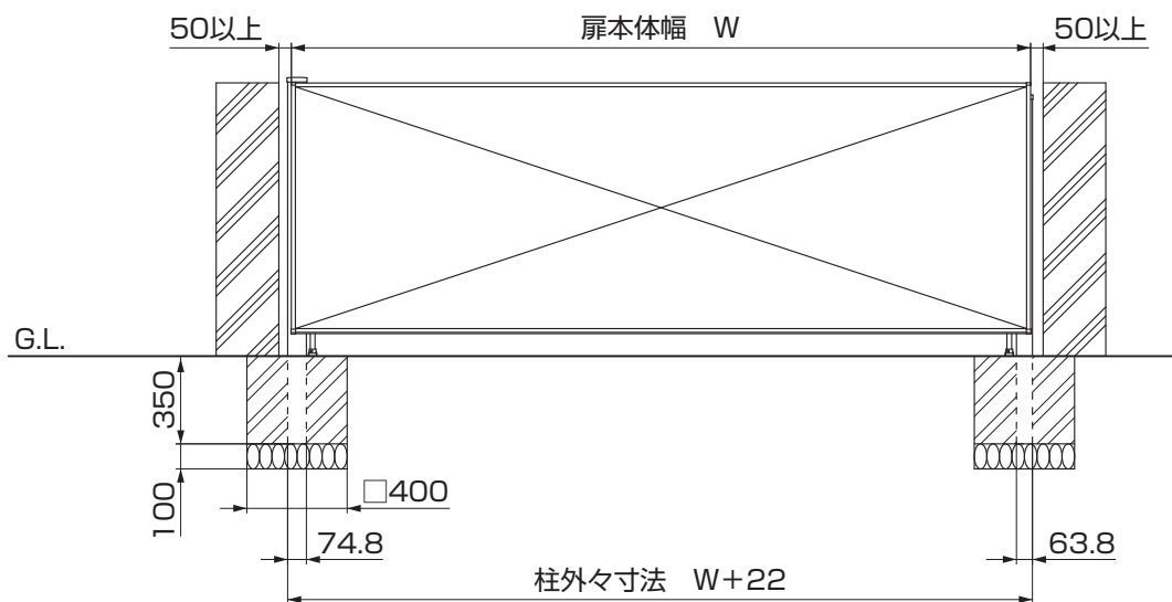
図2-6 正面図
