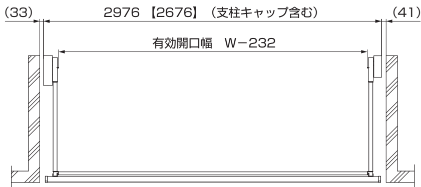
図2-1 平面図
