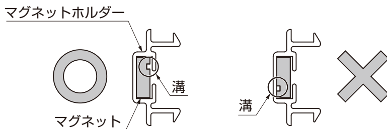
図3-3 片引きの場合
