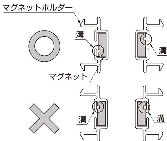
図3-4 引き分けの場合
