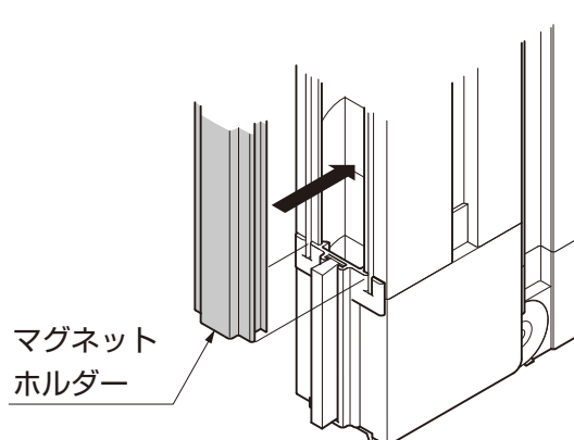
図3-5 マグネットホルダーの取付け
