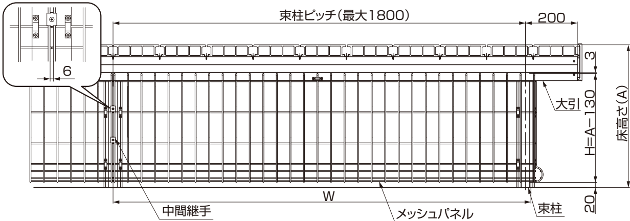
図1-1 正面図
