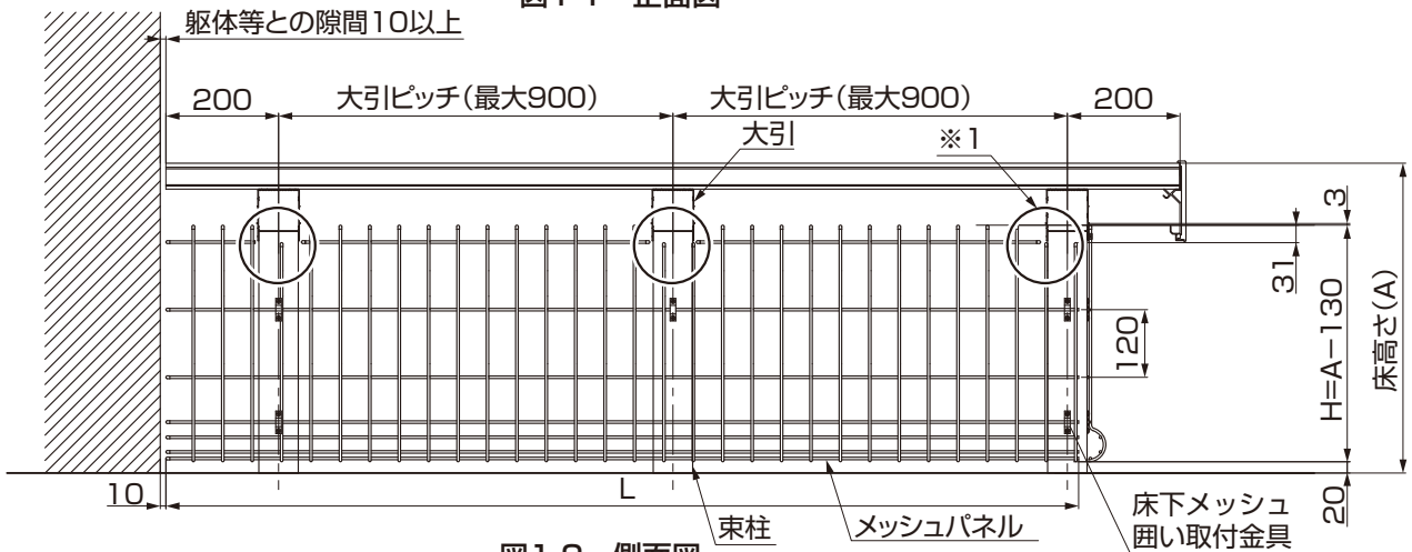
図1-2 側面図
