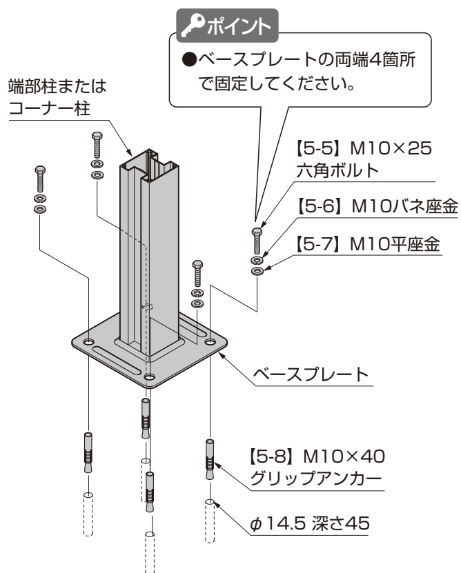
【5-8】 M10×40 グリップアンカー
