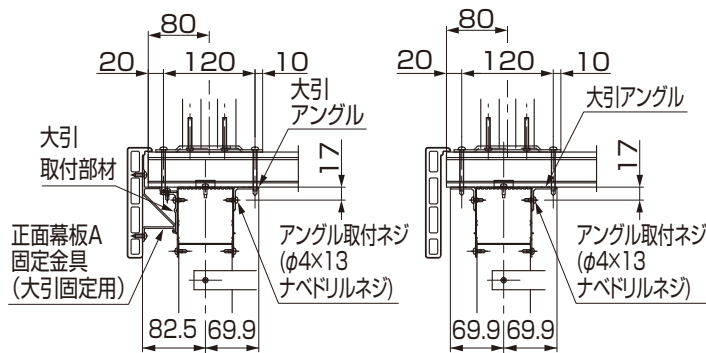
A-A矢視図
