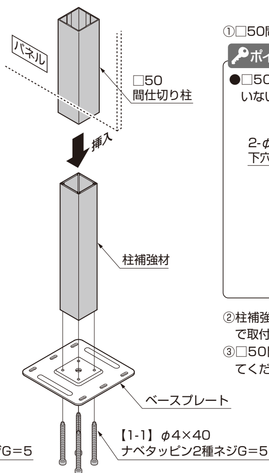
図4-2 側面固定の場合
