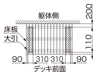
柱設置可能範囲(柱芯寸法)
