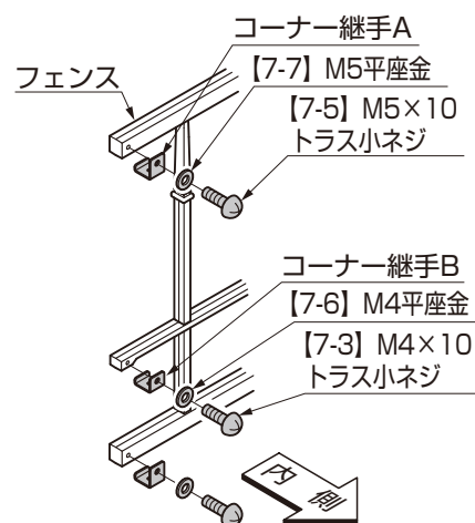
図7-3 コーナー部
