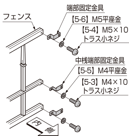
図7-1 端部
