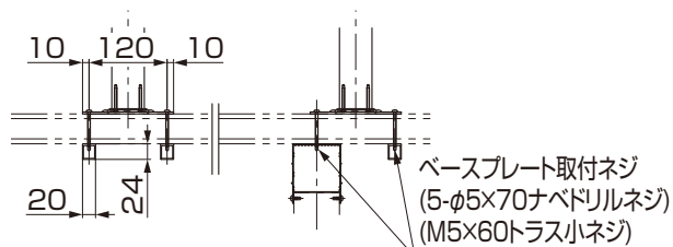
柱設置可能範囲(柱芯寸法)
