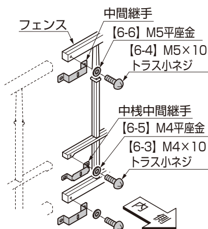
図7-2 中間部
