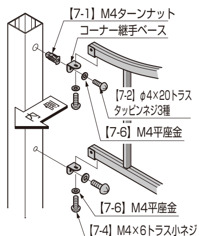
図6-6 コーナー部
