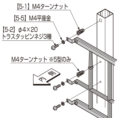
図7-4 端部
