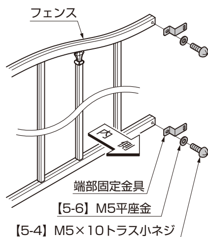
図6-1 端部
