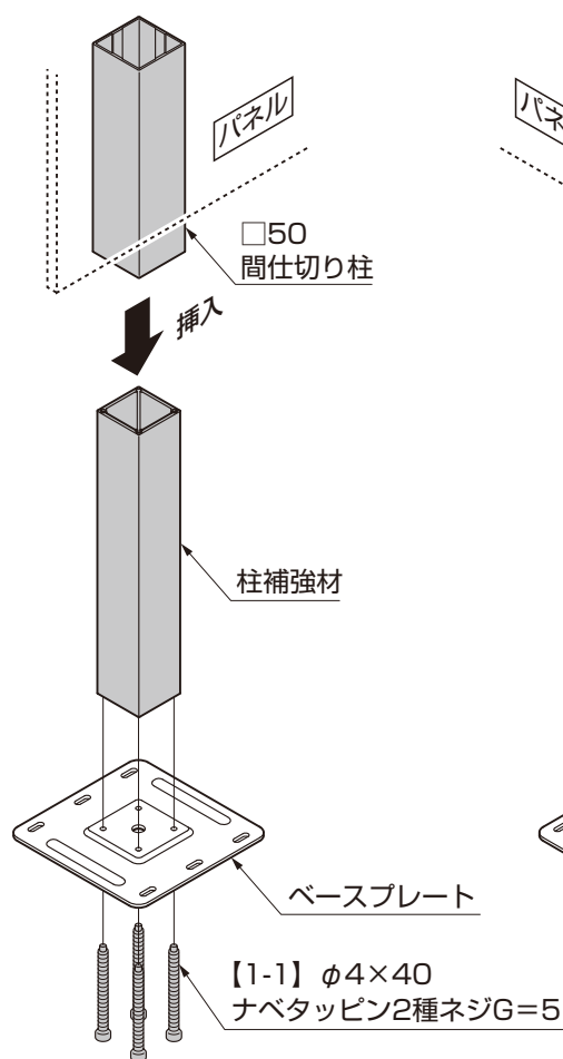
図4-1 正面固定の場合
