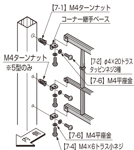
図7-6 コーナー部
