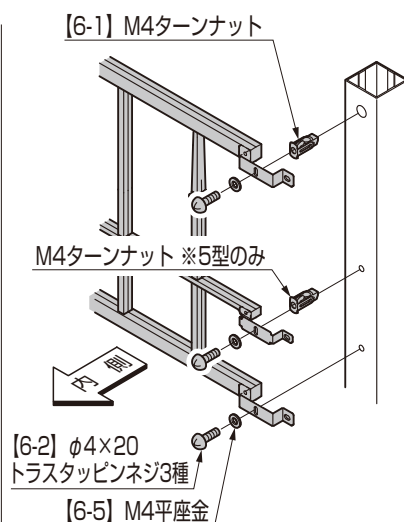
図7-5 中間部
