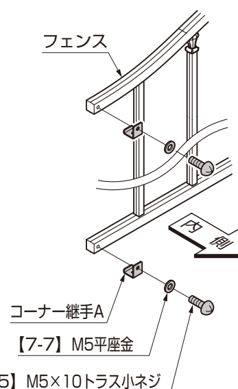
図6-3 コーナー部
