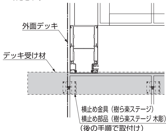
【外面デッキを切欠かない場合】
