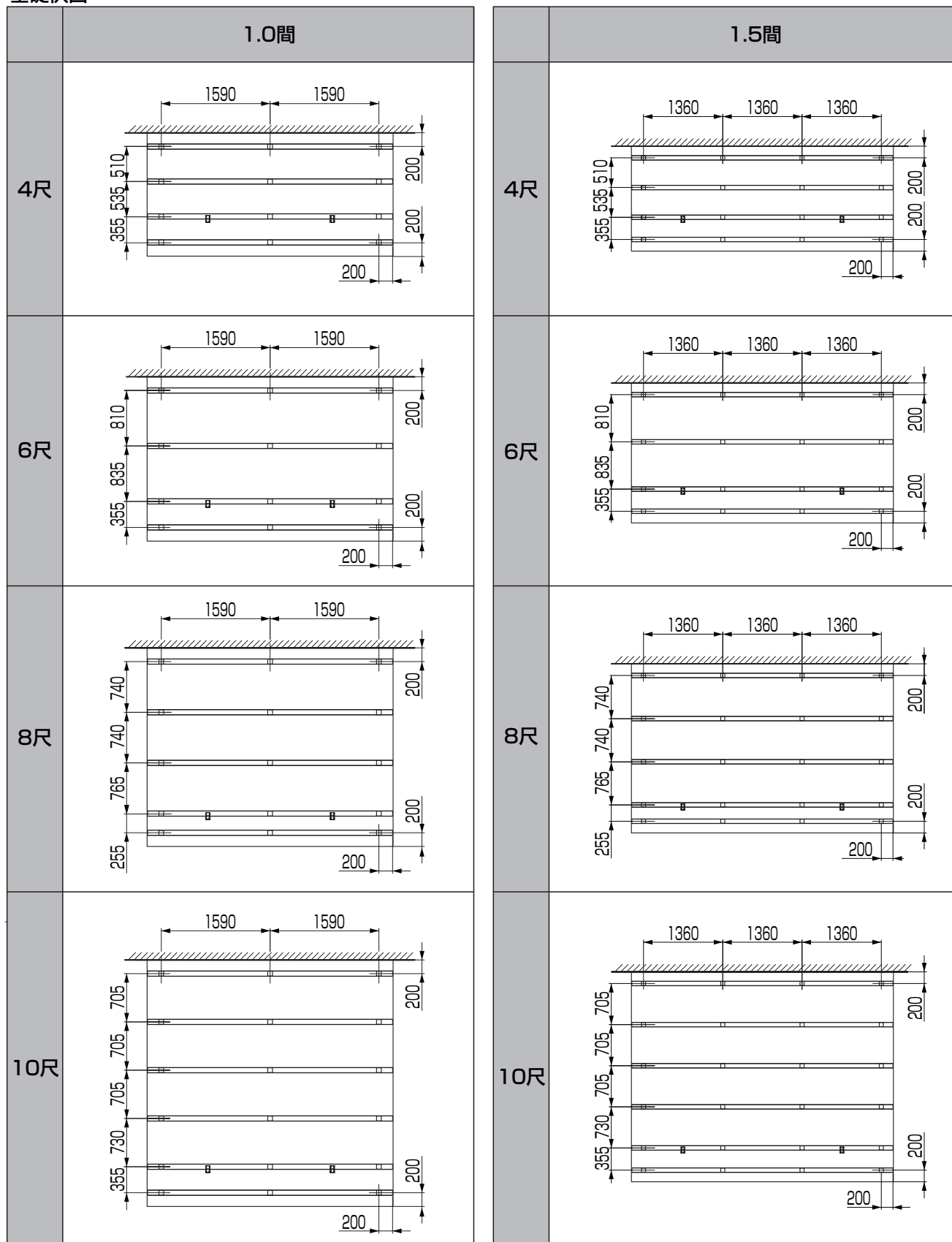
基礎伏図
