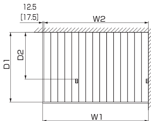
デッキ割付図
