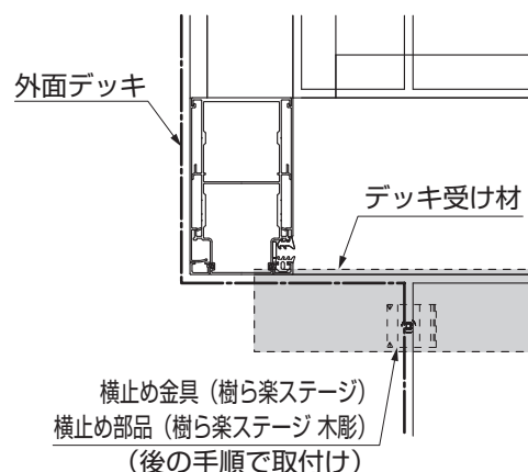
【外面デッキを切欠く場合】
