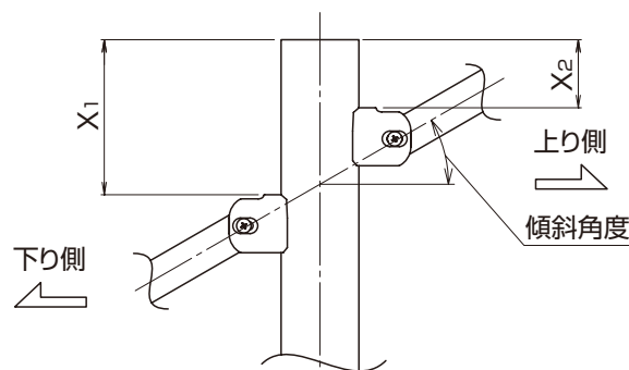
傾斜支柱フタ
