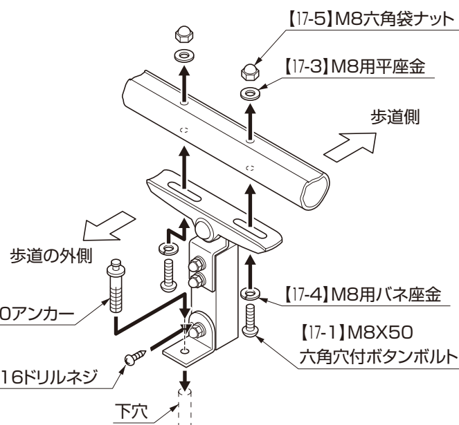
補助柱アンカー固定タイプ
