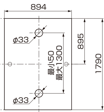
【中間】
