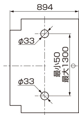
【端部(外観右)】※左は対称
