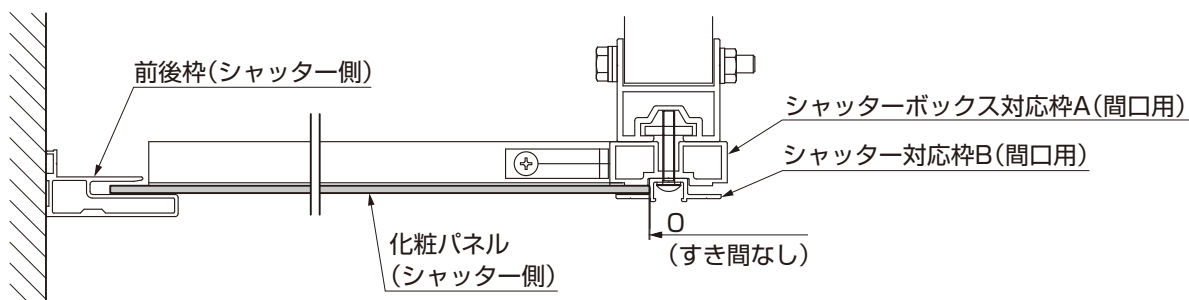
【間口方向断面図】
