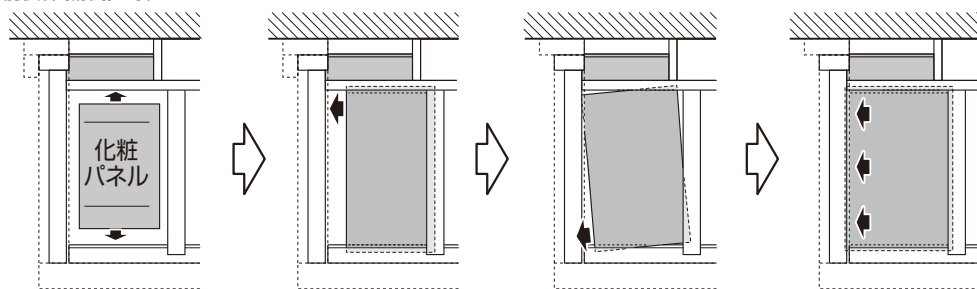
化粧パネル取付け方法概略図
