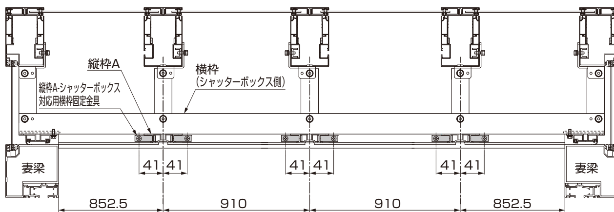
【縦枠A取付けピッチ】
