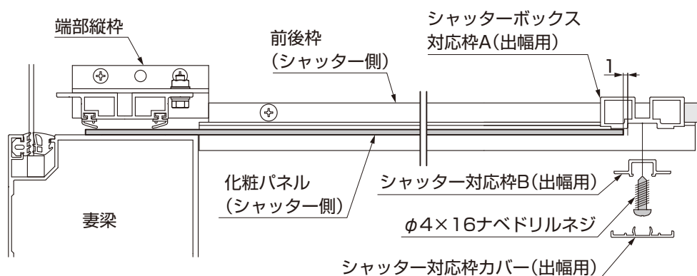
【間口方向断面図】
