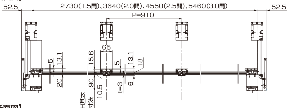
【A-A断面図】
