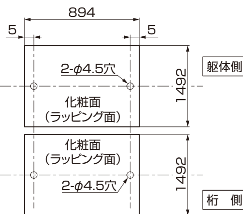
【中間】
