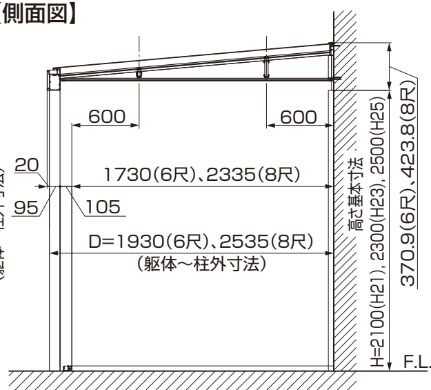
【側面図】
