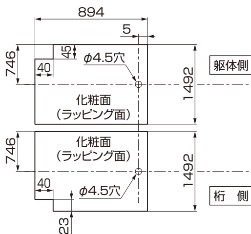
【端部(外観右)】※左は対称
