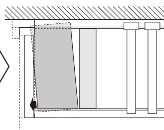
0.5間化粧パネル取付け方法概略図
