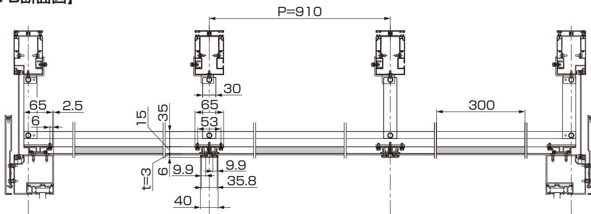
【B-B断面図】
