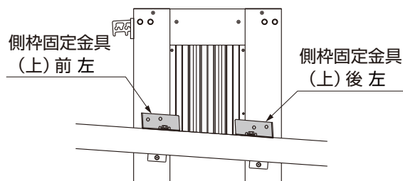
図8-3 右側面
