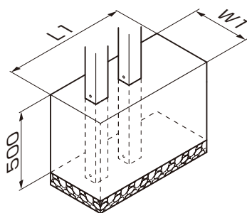
図5-2 土間コンなしの場合
