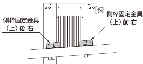
図8-2 左側面
