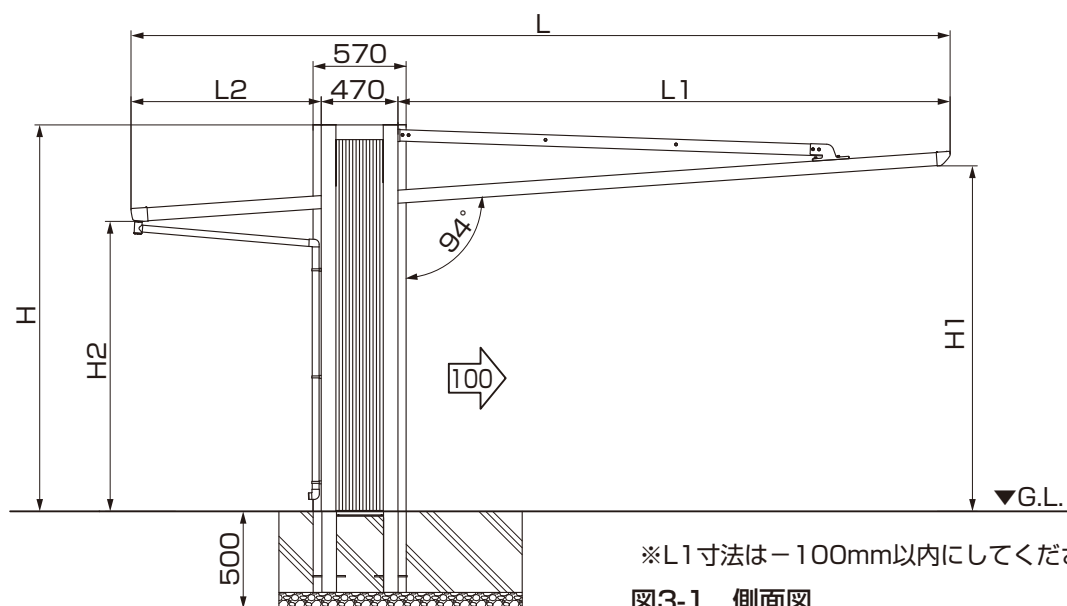
図3-1 側面図
