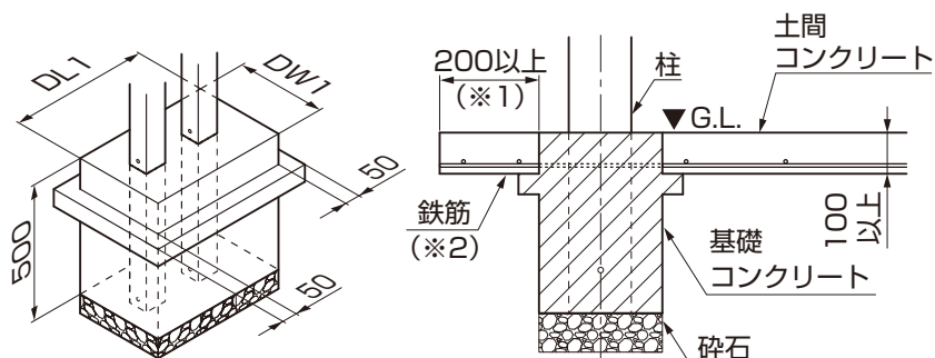
図5-3 土間コンクリート併用基礎の場合
