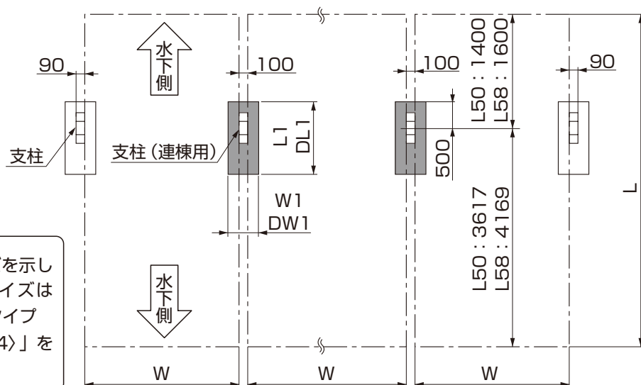
図5-1 基礎位置
