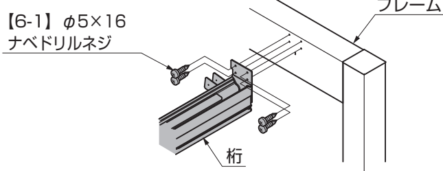
図2-9 フレームへ取付ける場合
