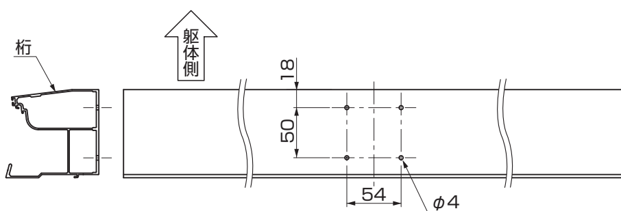
図2-20 桁の加工
