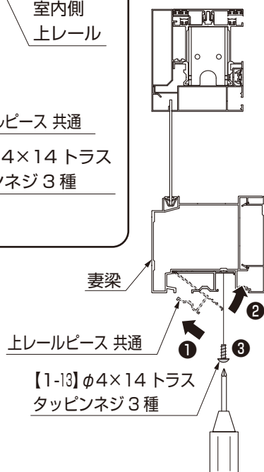
図 1-19 側面図 (妻梁側)
