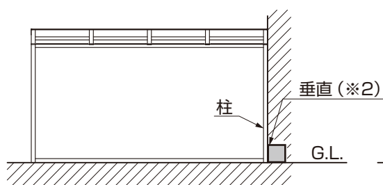
図6-14 正面図
