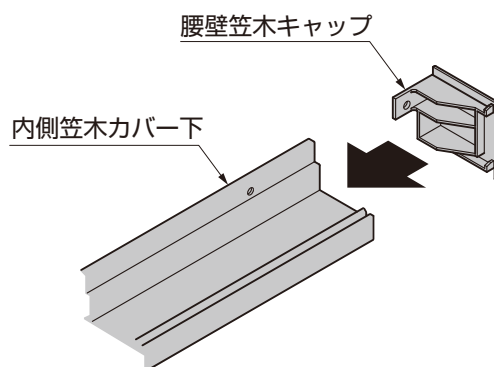
図12-10 腰壁笠木キャップの取付け
