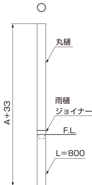
図17-4 加工寸法 (連結時)
