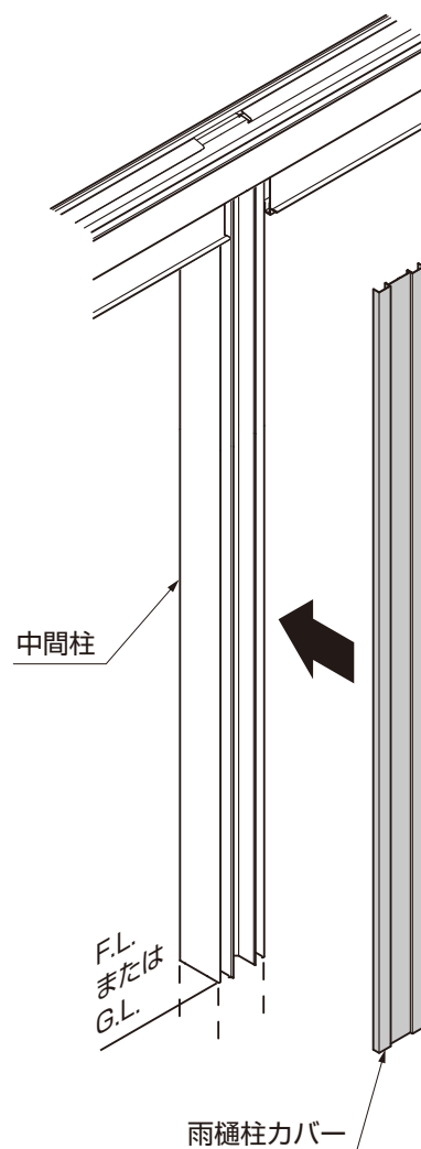
図17-9 中間柱の場合
