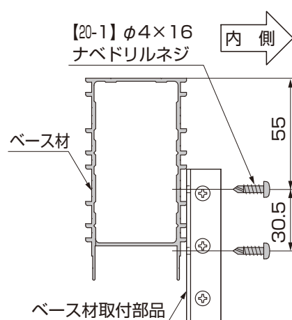
図10-10 出幅側 躯体
