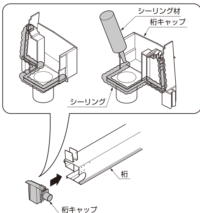
図1-10 桁キャップ
