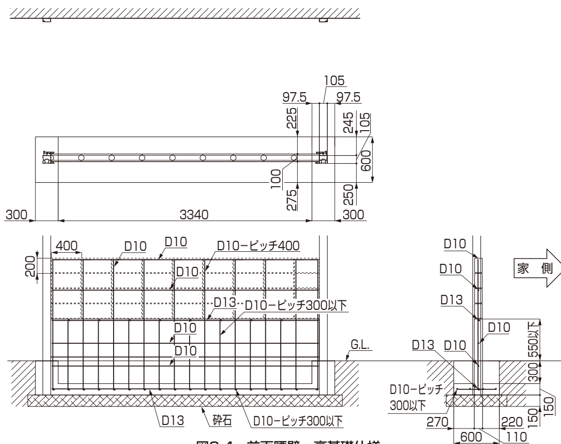
図8-4 前面腰壁 高基礎仕様
