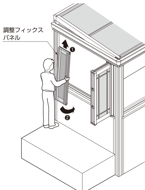
図2-9 調整フィックスパネル 腰壁
