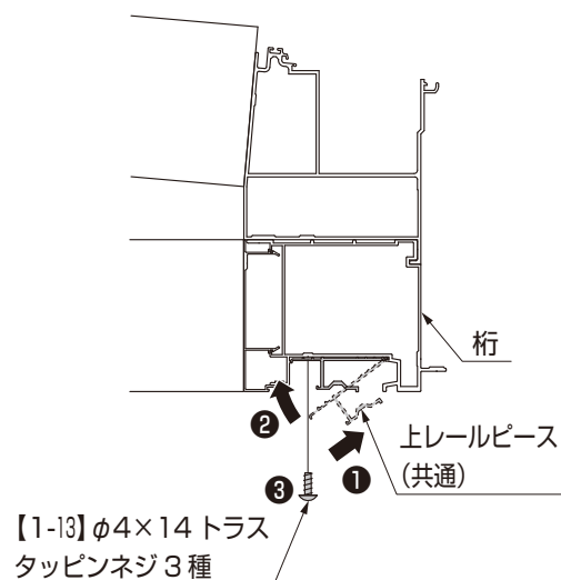
図 1-20 正面図 (桁側)
