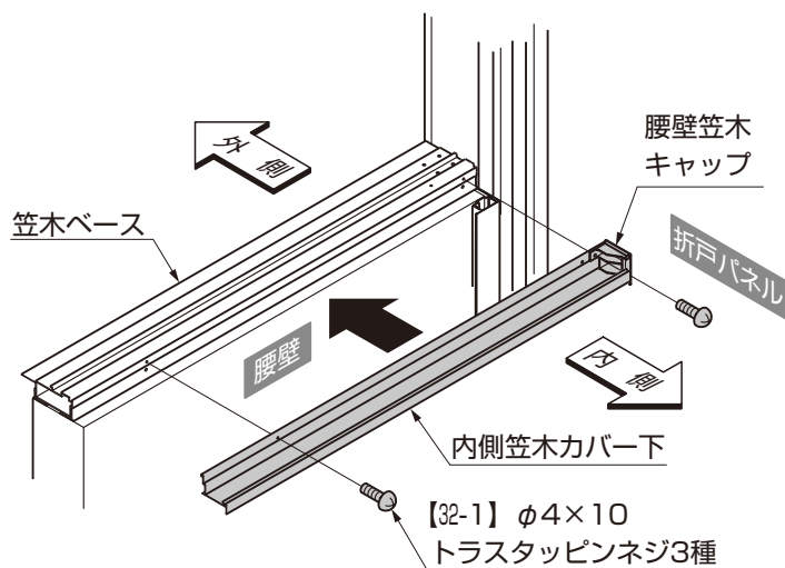
図12-11 内観図
