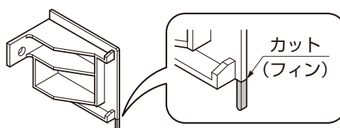
図12-9 腰壁笠木キャップ（間口側）
