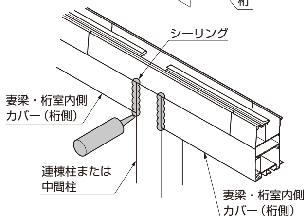
図12-8 連棟仕様・中間柱仕様
