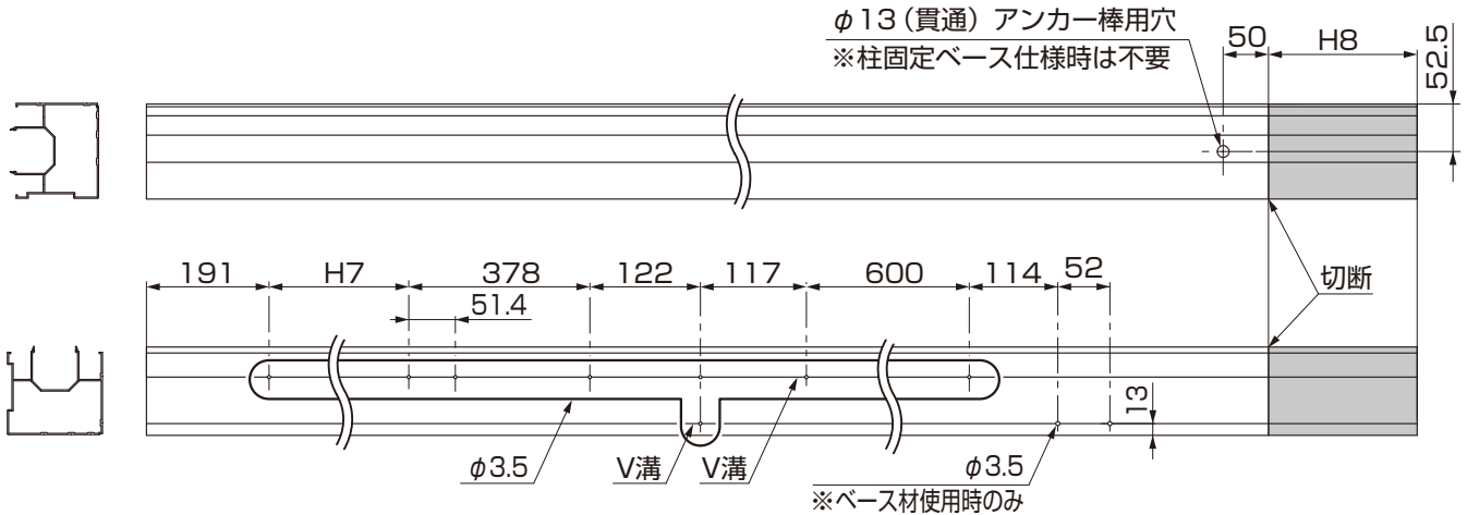
図3-6 主柱
