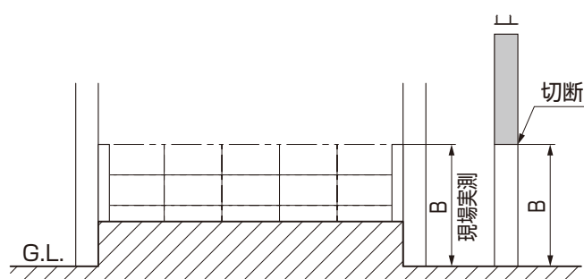
図11-2 内側
