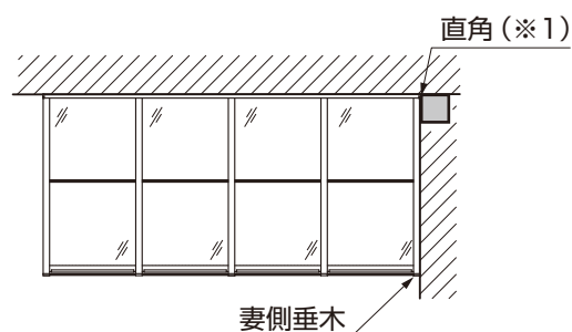
図6-13 上面図
