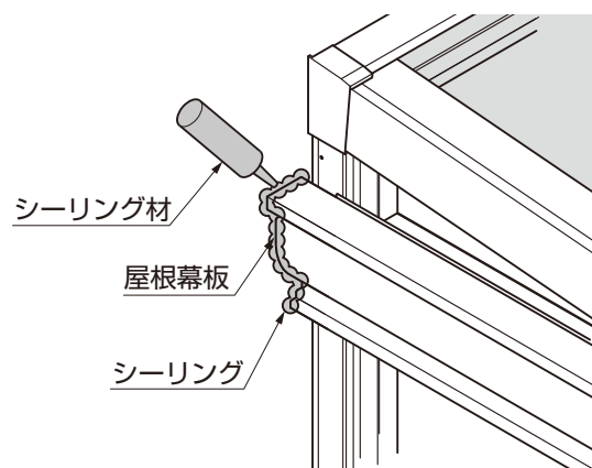
図1-19 屋根幕板
