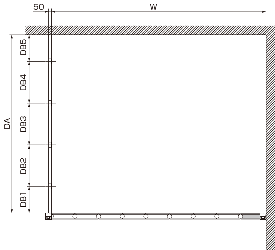
図3-2 基礎伏図
