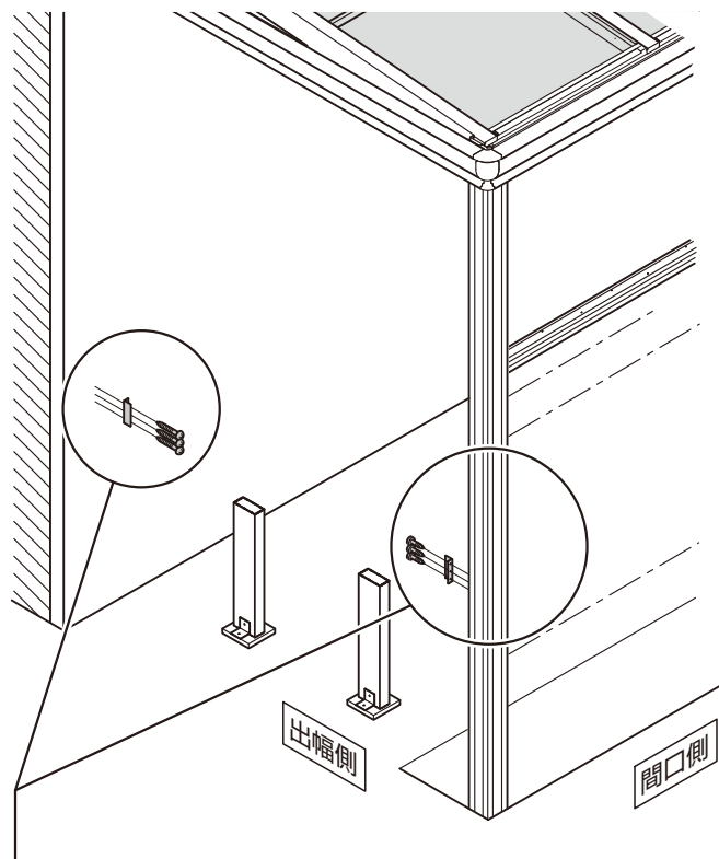
図10-5 ベース材取付部品躯体側の加工 ※柱側および間口側の現場加工はありません。
