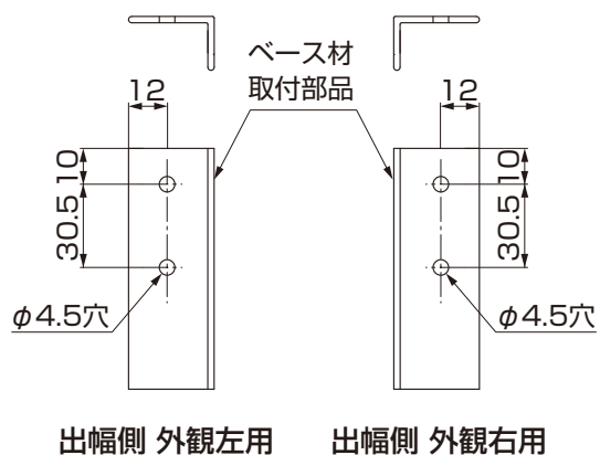
図10-5 ベース材取付部品躯体側の加工 ※柱側および間口側の現場加工はありません。
