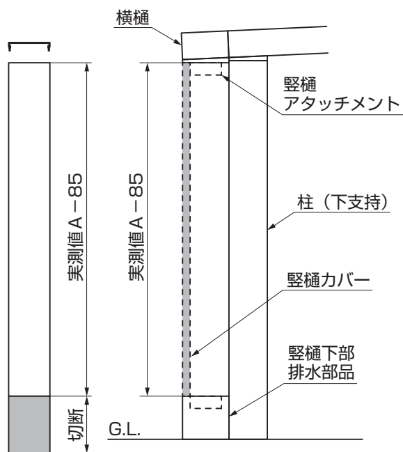
図2-2 竖樋カバーの加工
