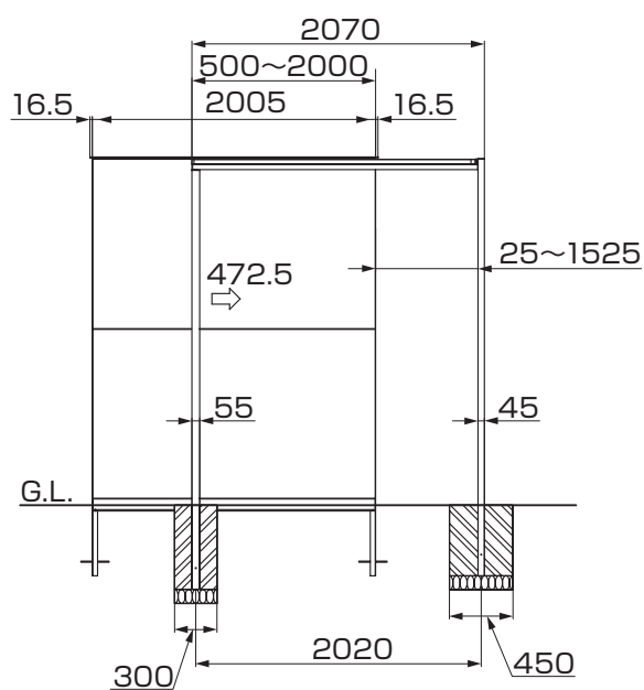
図1-4 背面図
