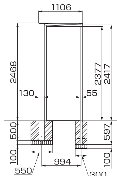
図1-3 右側面図
