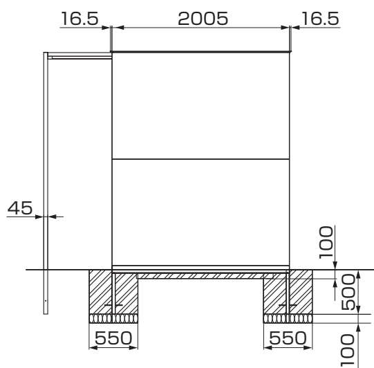
図1-2 正面図
