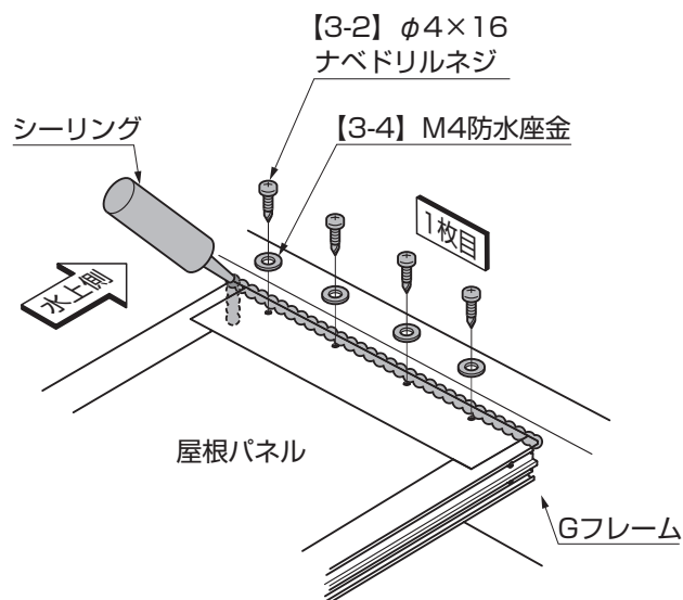
図7-3 B部 中間部水上側
