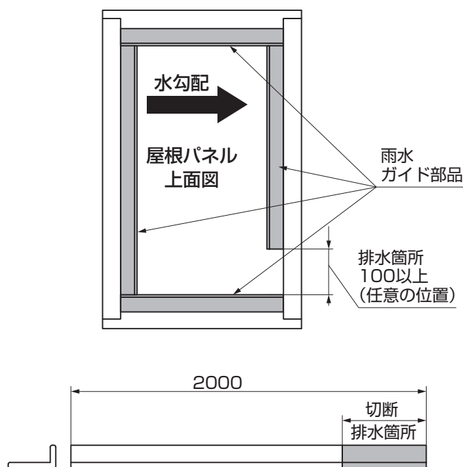
図2-1 排水箇所の切断（雨水ガイド部品）
