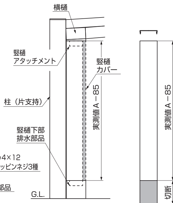
図2-4 縦樋カバーの加工
