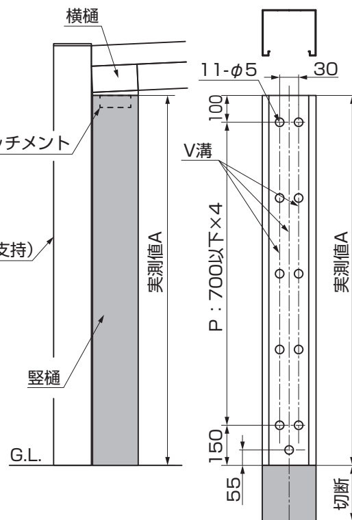
図2-3 縦樋の加工
