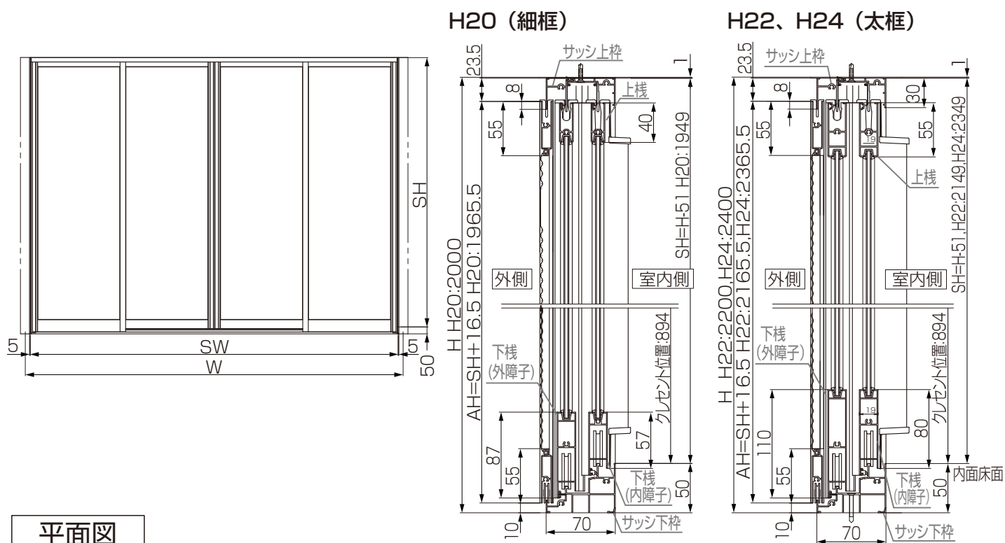
縦断面図
