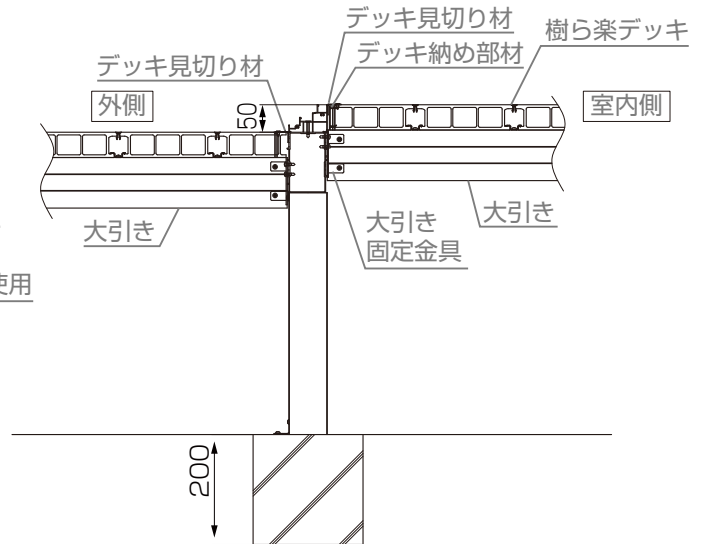
デッキ仕様間口断面
