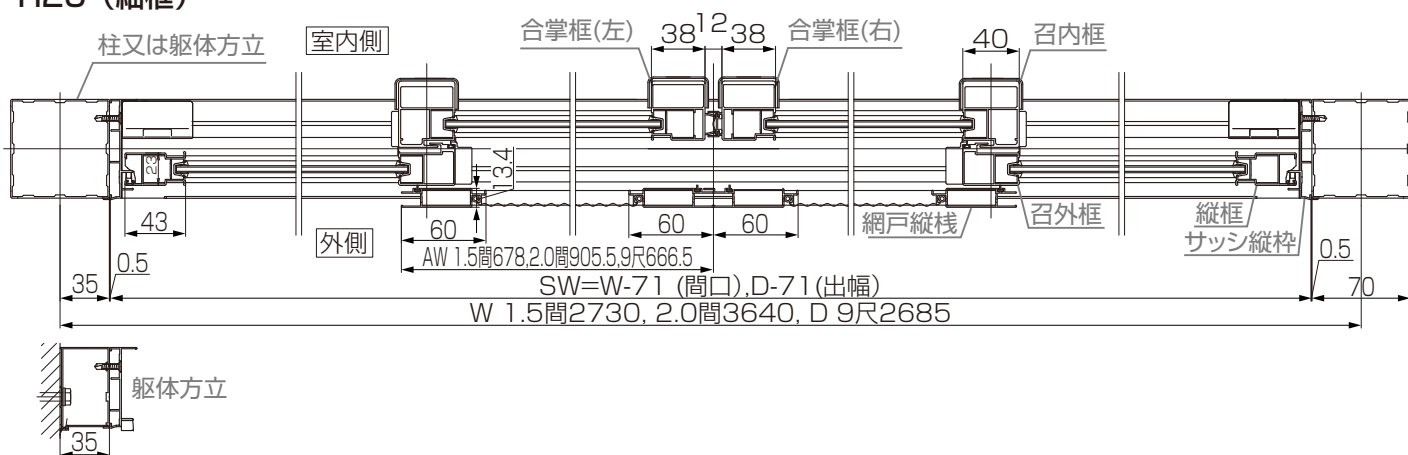
平面図
