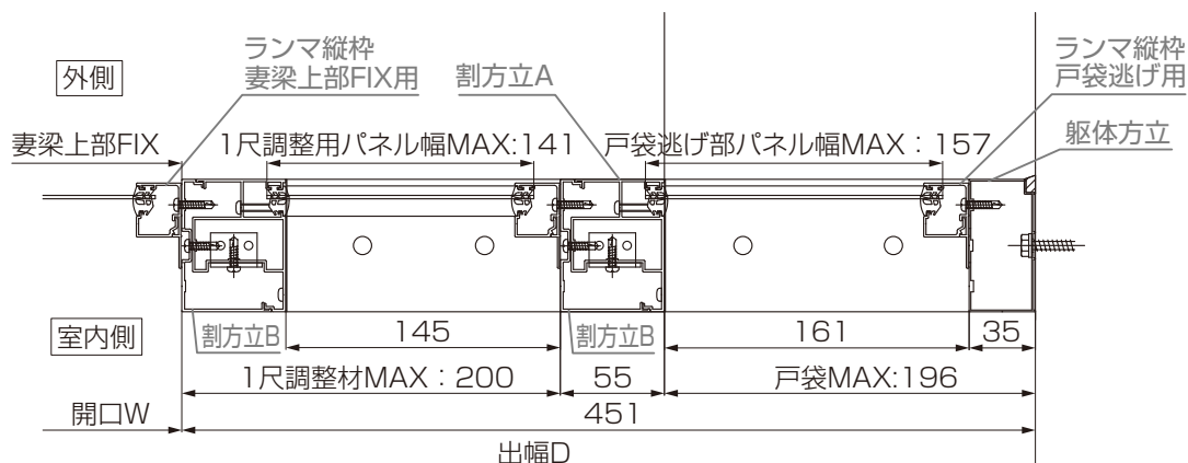
A-A断面
