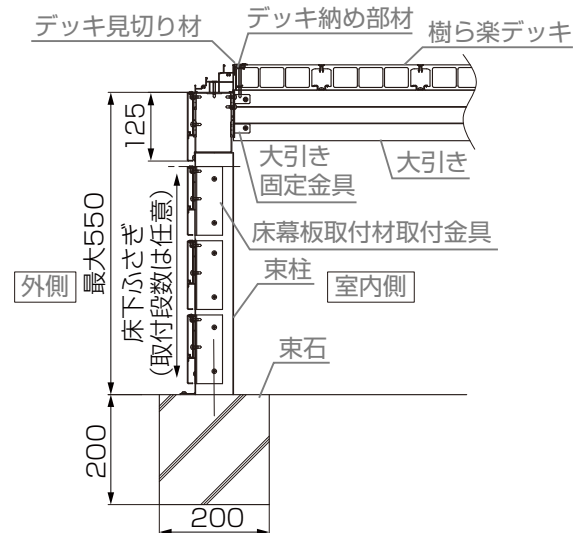
インナーデッキ仕様間口断面
