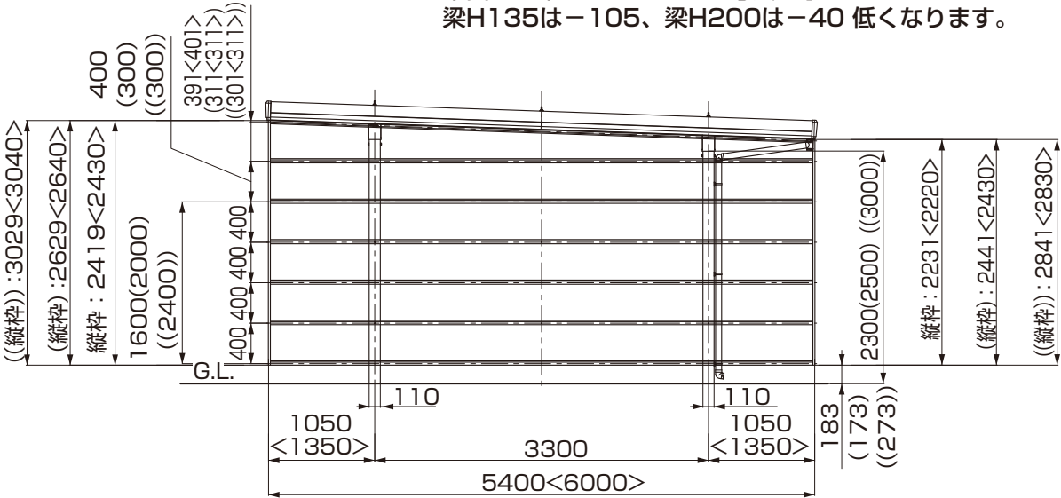
図2-7 4本柱
