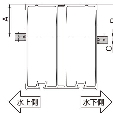
図4-6 梁240W
