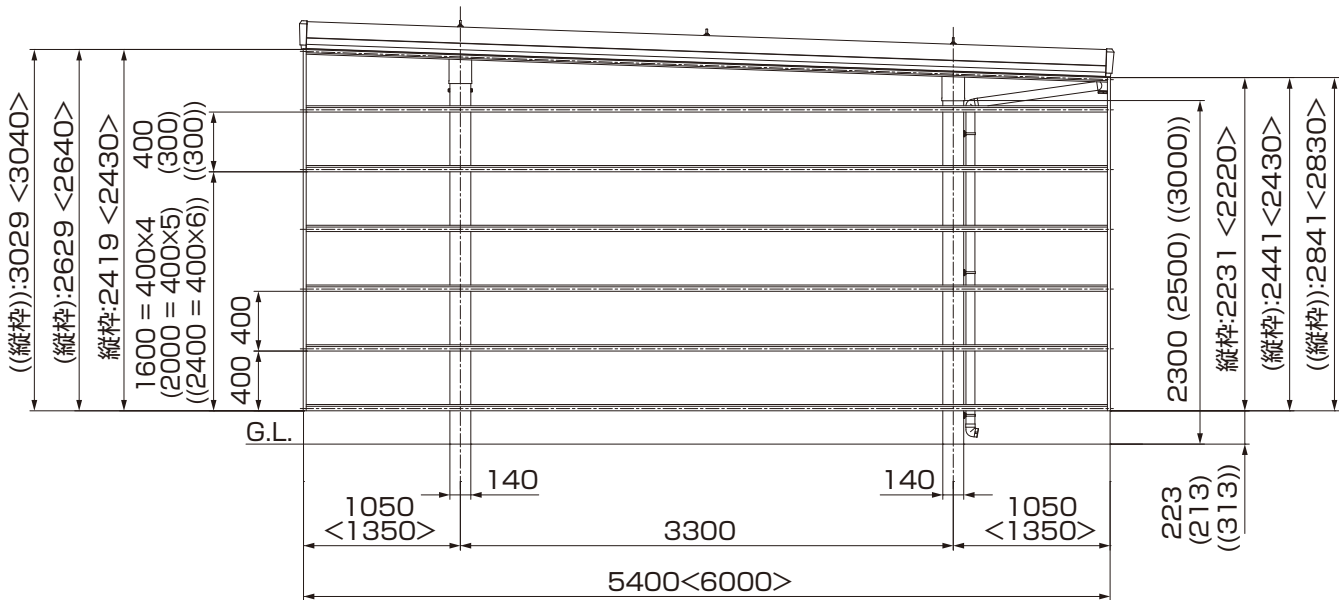
図2-10 4本柱(梁280)
