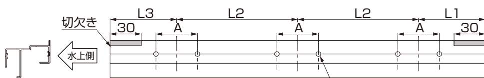
図3-8 6本柱
