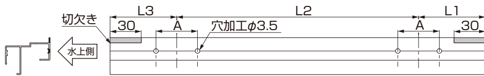
図3-7 4本柱
