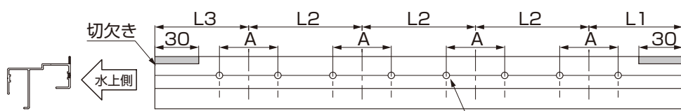
図3-9 8本柱
