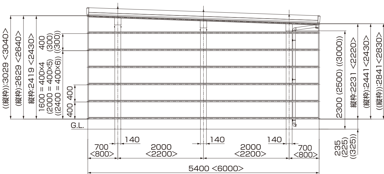
図2-11 6本柱(梁280)
