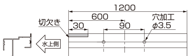
図3-10 12延長
