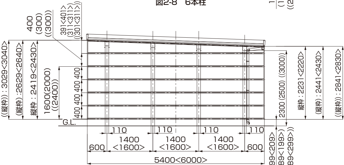
図2-9 8本柱
