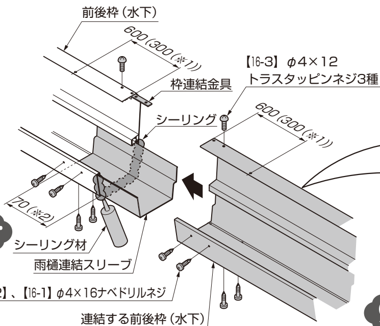
図5-6 前後枠 (水下)
