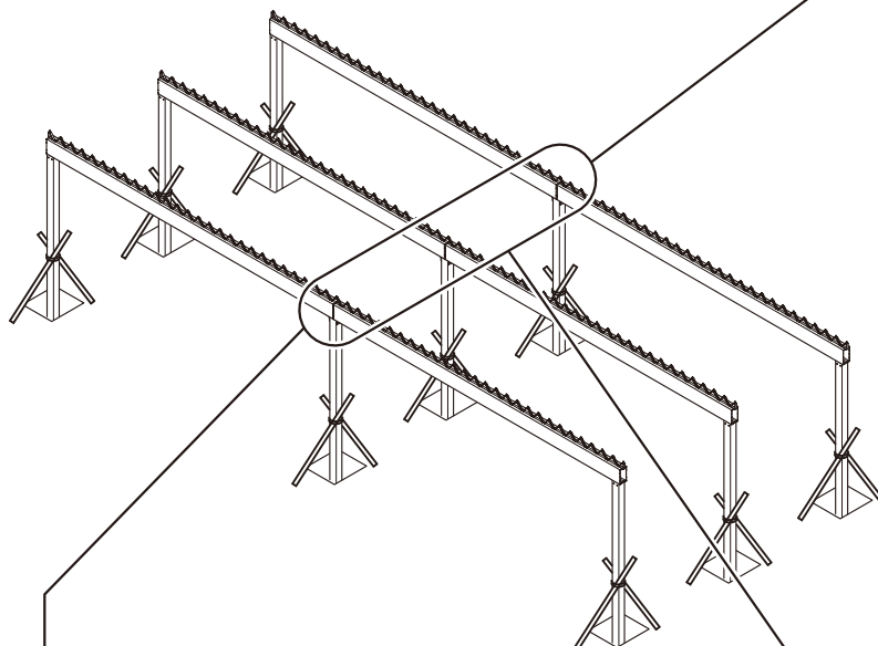
図2-6 横連棟仕様
