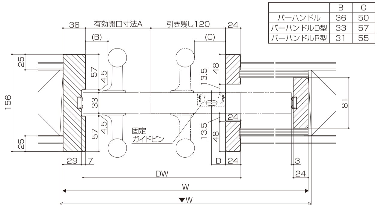
横断面図
