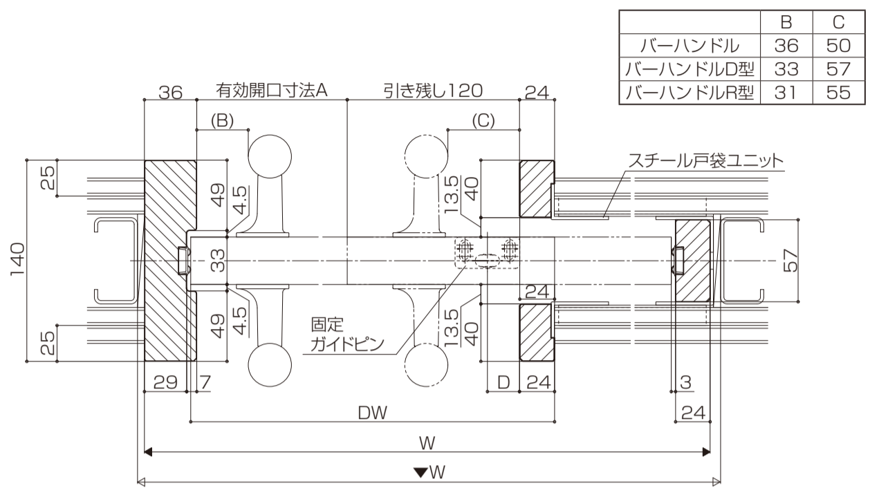
横断面図
