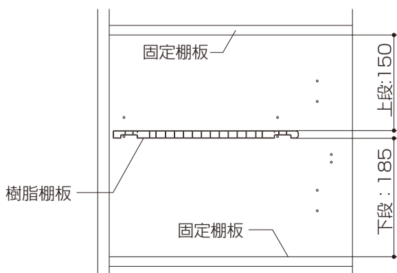
【樹脂棚板を下の穴に取付けた場合】
