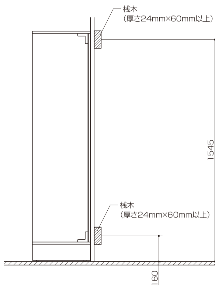
【棧木を設置する場合】
