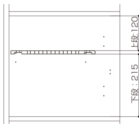
【樹脂棚板を上の方の穴に取付けた場合】
