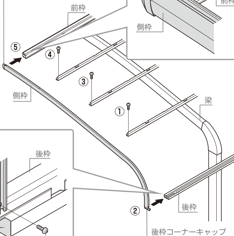
【1-3】φ5×12 トラスタッピンネジ3種
