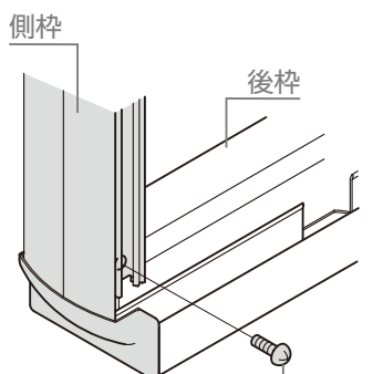
【1-3】φ5×12 トラスタッピンネジ3種
