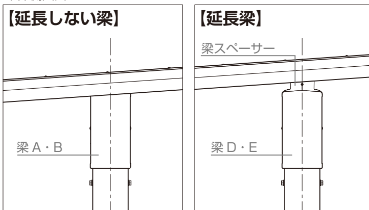
梁部側面図
