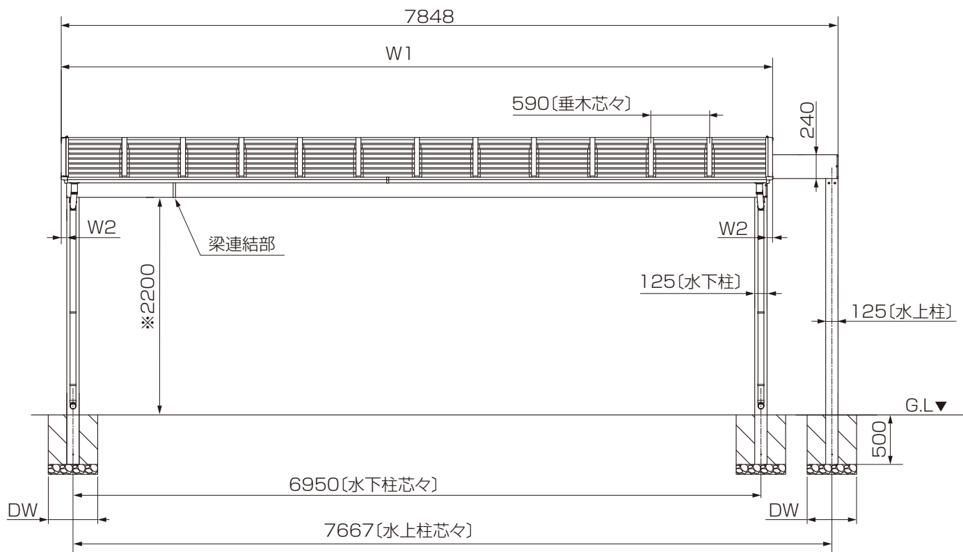
梁部側面図
