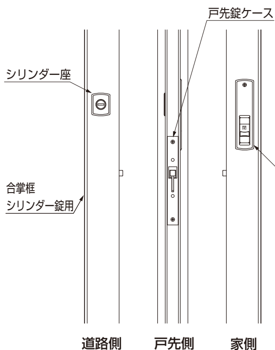
図3-3 シリンダー錠
