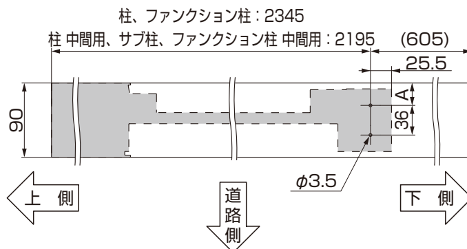
図1-2 柱側面図
