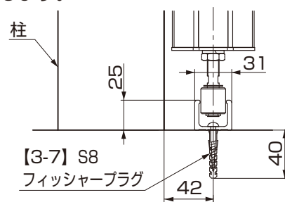
図4-2 ガイドレール詳細図
