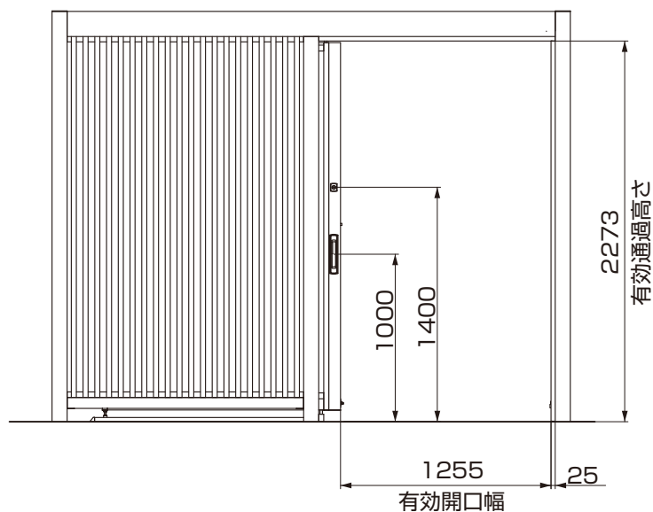
図3-2 吊引戸本体W15の場合
