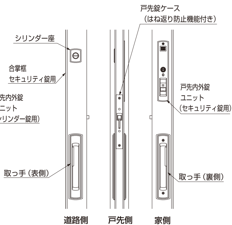
図3-4 セキュリティ錠
