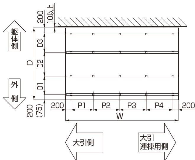
3-1 基本寸法
