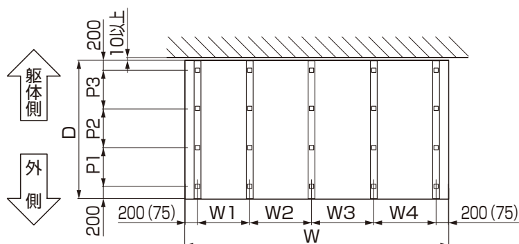
4-1 基本寸法
