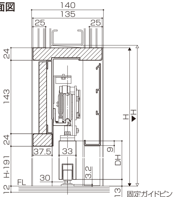
横断面図
