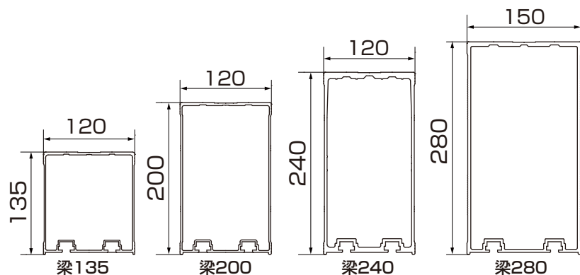
図1-5 梁断面図
