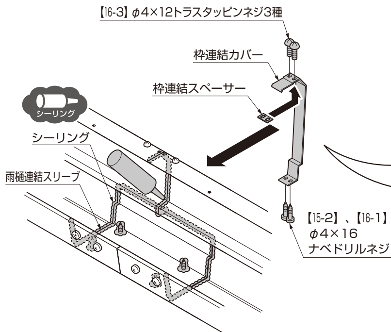
図5-10 前後枠（水下）
