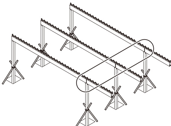
図2-5 幅18延長仕様
