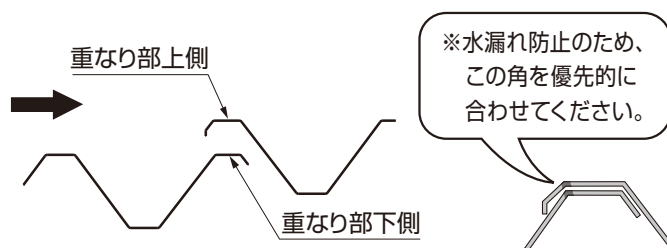
図4-6 折板重なり部詳細図
