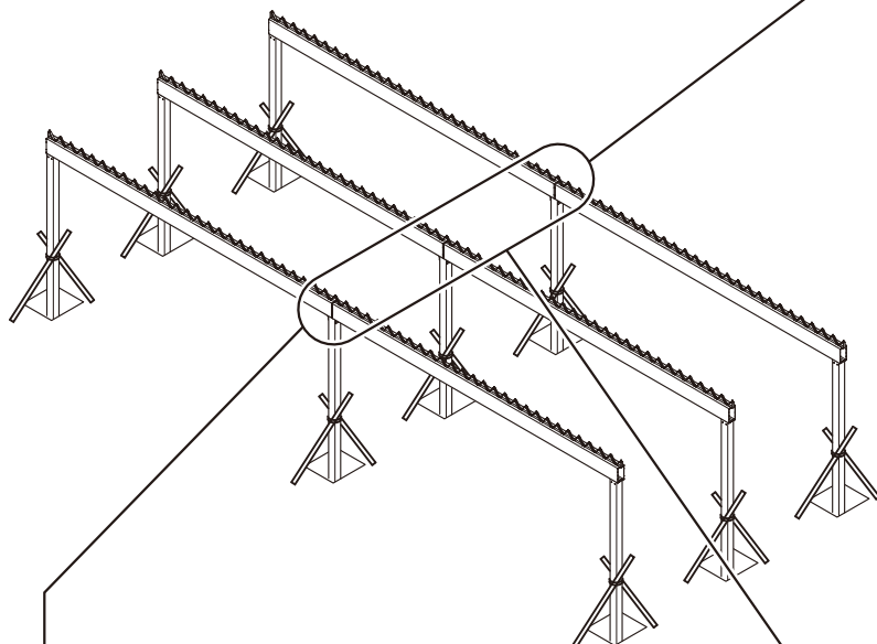
図2-6 横連棟仕様
