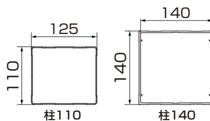
図1-6 柱断面図
