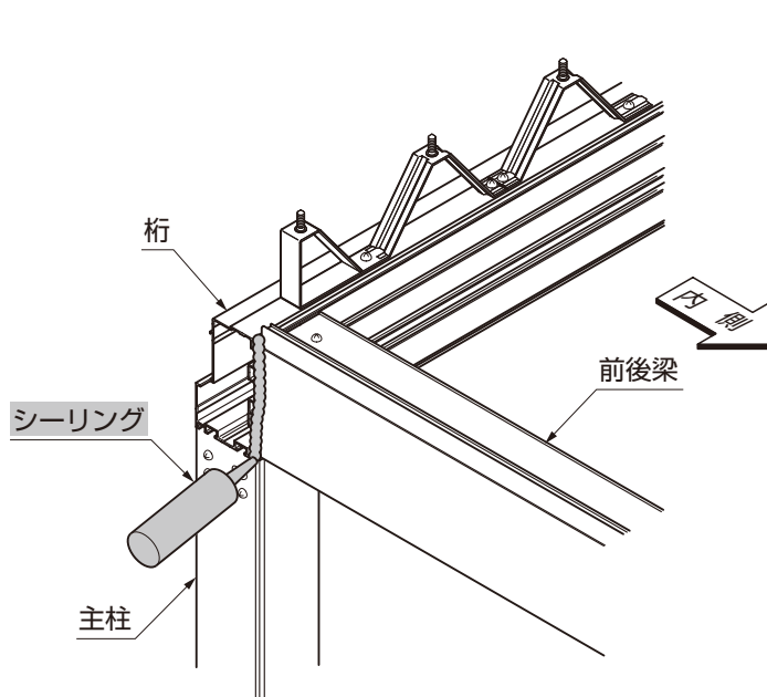
図1-1 桁・前後梁
