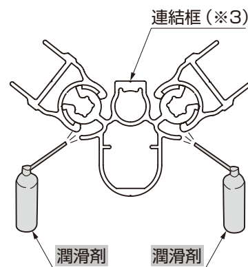
図1-16 B部パネル連結部
