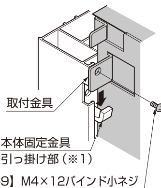
図5-2 A部詳細図
