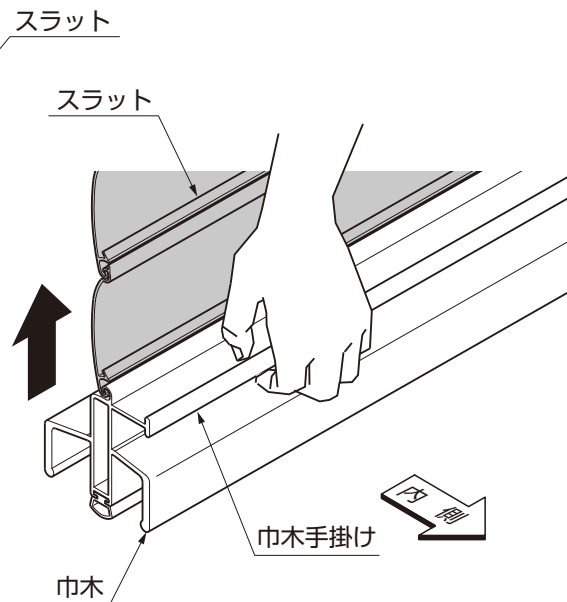
図14-2 手動におけるスラットの巻き上げ
