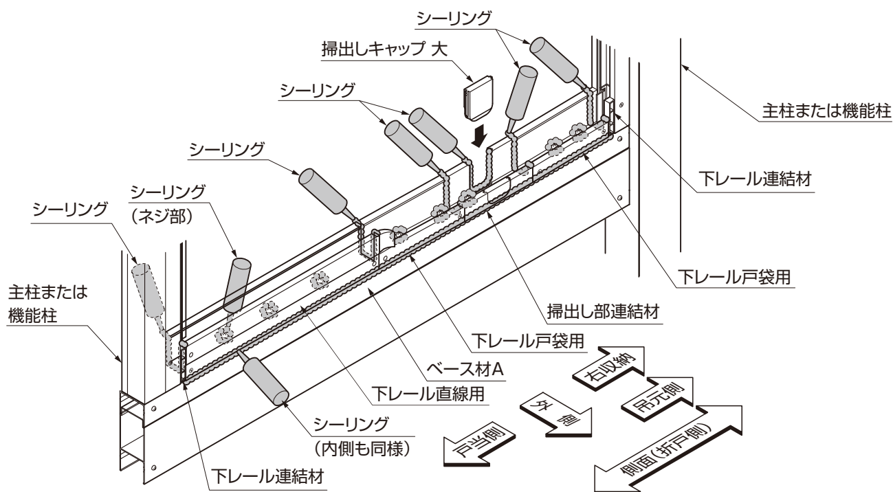
図1-5 下レール（下レールが土間仕上げ面より露出する場合）
