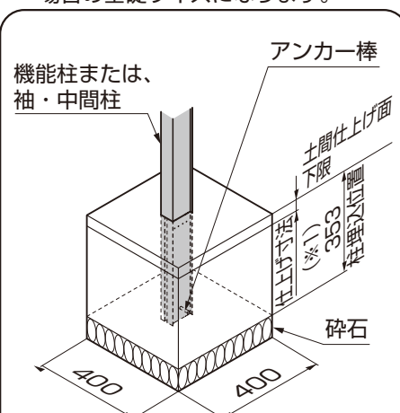
図2-22 機能柱または袖・中間柱の場合
