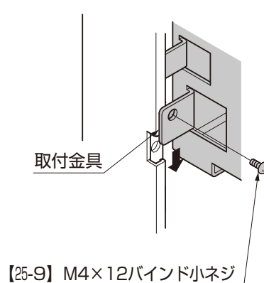
図5-3 B部詳細図
