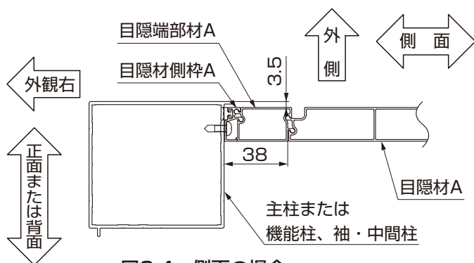
図2-4 側面の場合
