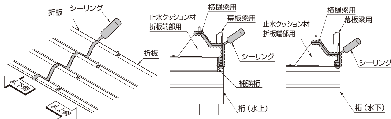
図1-8（横延長）折板屋根材重ね部分
