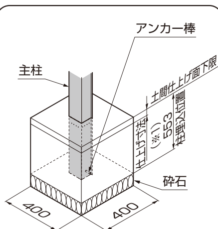
図2-21 主柱の場合
