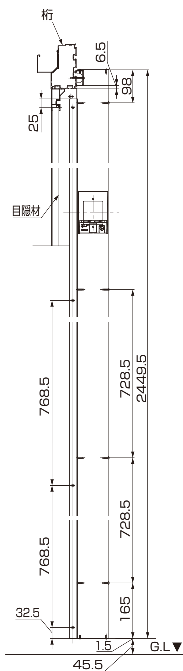
図2-3 C-C断面図 配線カバー支柱
