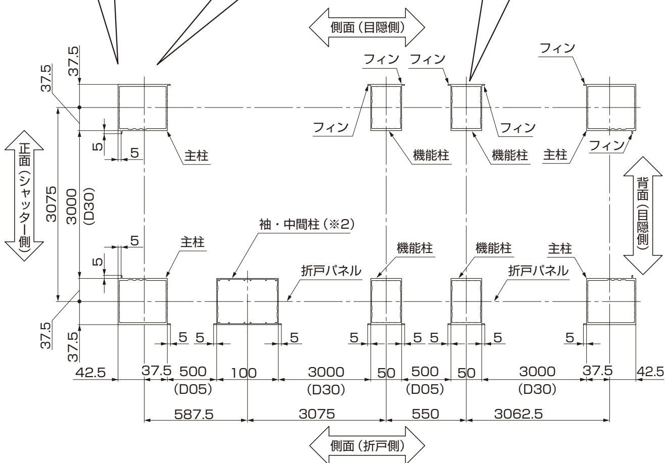
図2-22 機能柱または袖・中間柱の場合
