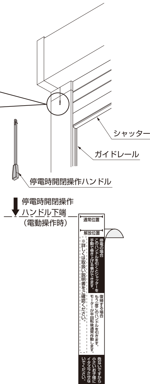
図7-3 停電開閉表示ラベル
