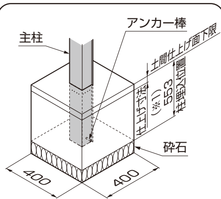
図2-16 主柱の場合
