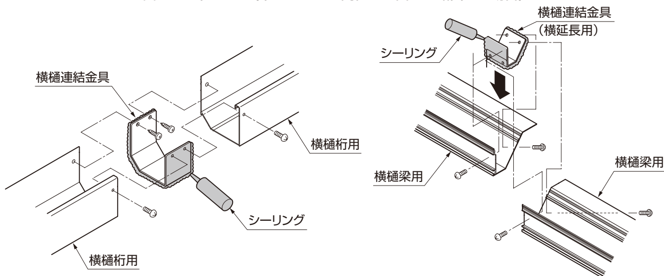
図1-6 横樋桁用（縦延長・縦横延長の場合）
