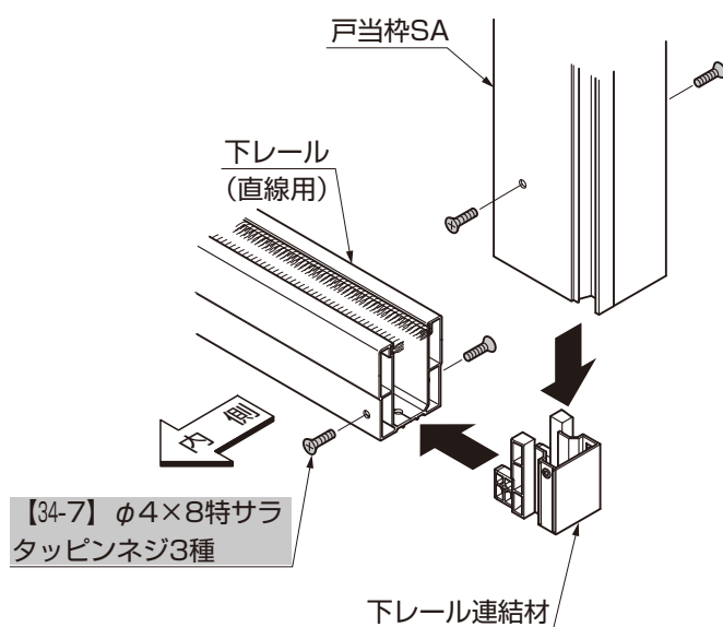
図1-13 戸当枠SAと下レール(直線用)の取付け
