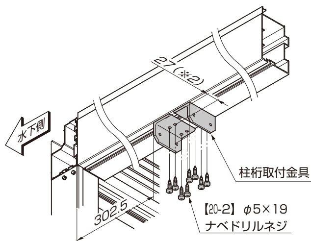
図11-1 柱桁取付金具の取付け（正面袖部分）
