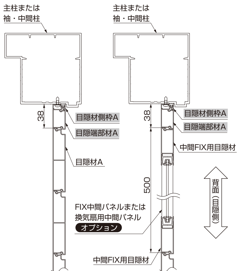
図2-4 目隠材の場合
