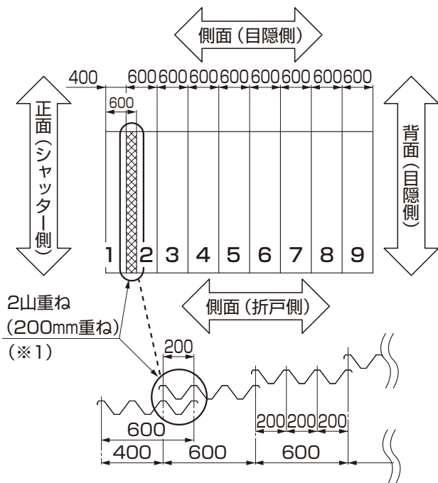
図16-1 L54の場合
