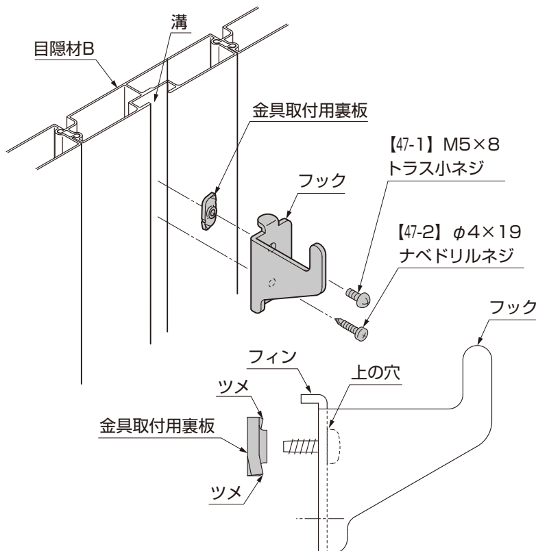
図9-2 フックの取付け
