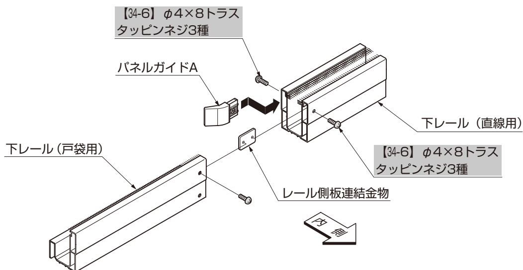
図1-14 下レール(戸袋用)と下レール(直線用)の取付け
