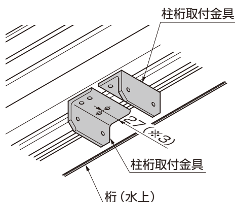
図6-5 B部詳細図 中央部の位置
