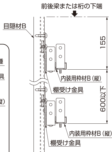
図4-3 内装用枠材Bの取付け高さ
