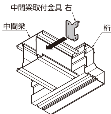
図12-3 中間梁の取付け
