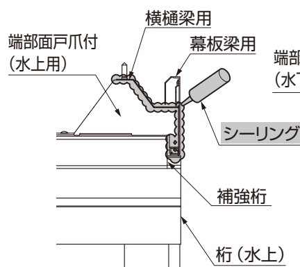
図1-10 (水上側) 端部面戸
