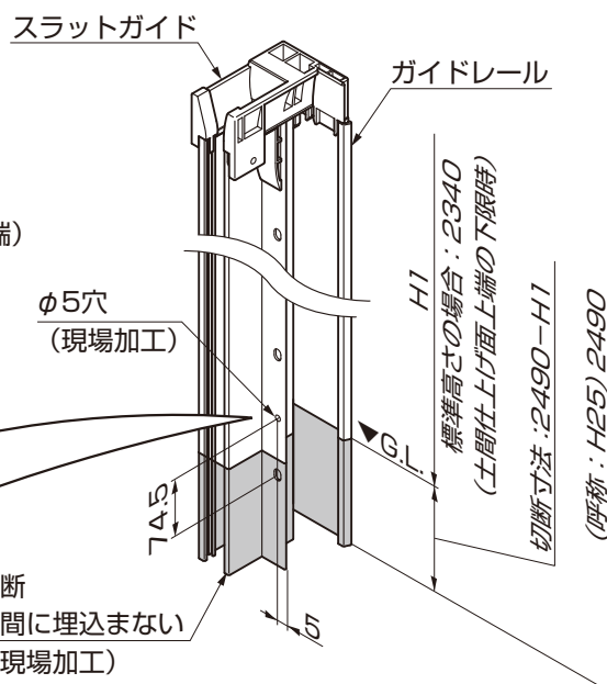
図3-2 ガイドレールの加工
