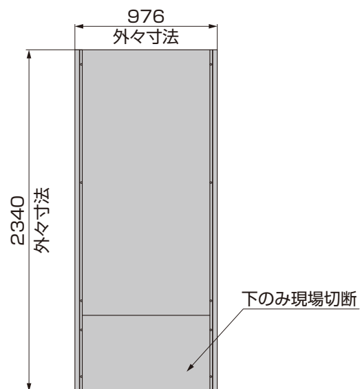
図2-2 内装パネル縦（壁付け）
