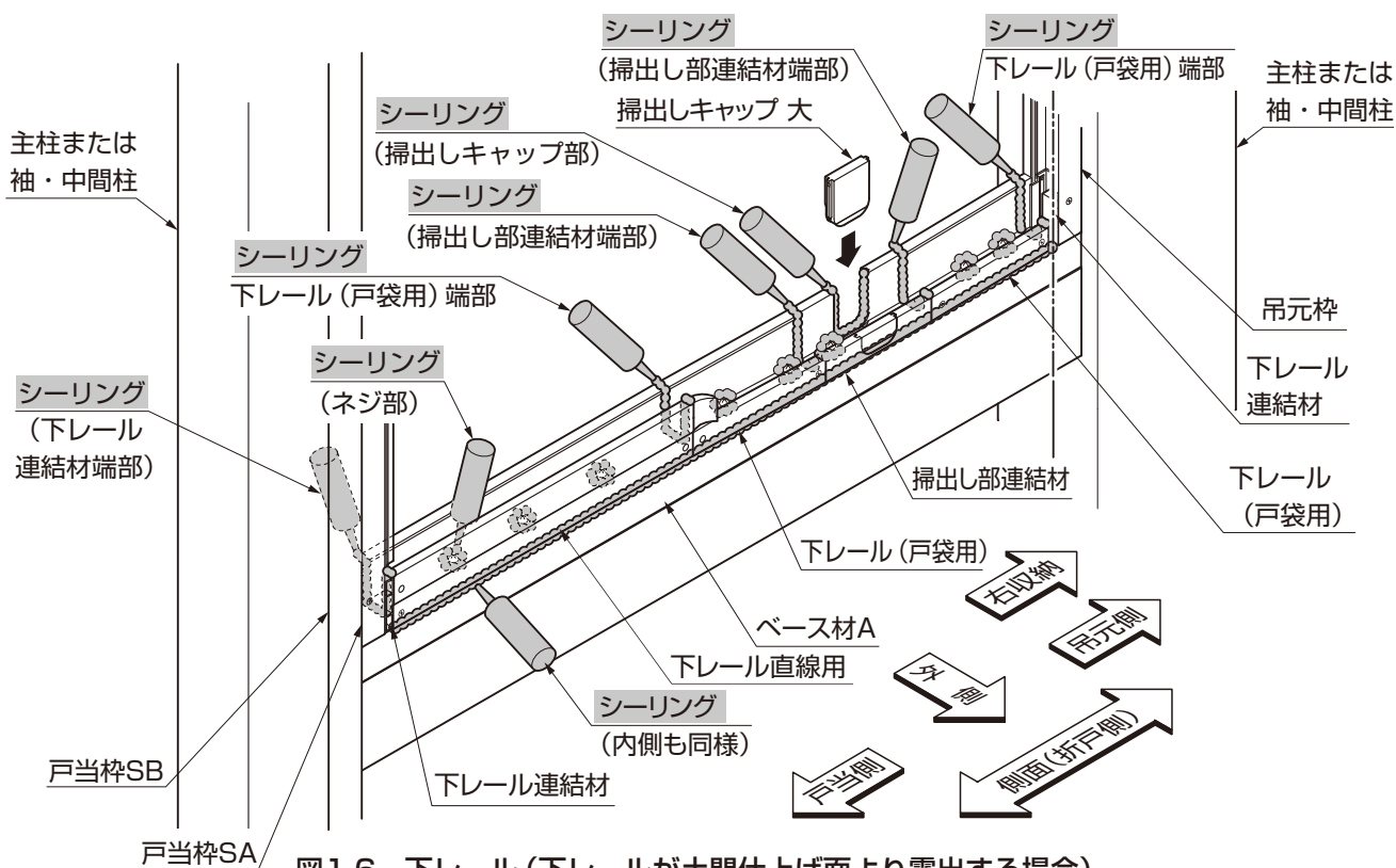
図1-6 下レール(下レールが土間仕上げ面より露出する場合)
