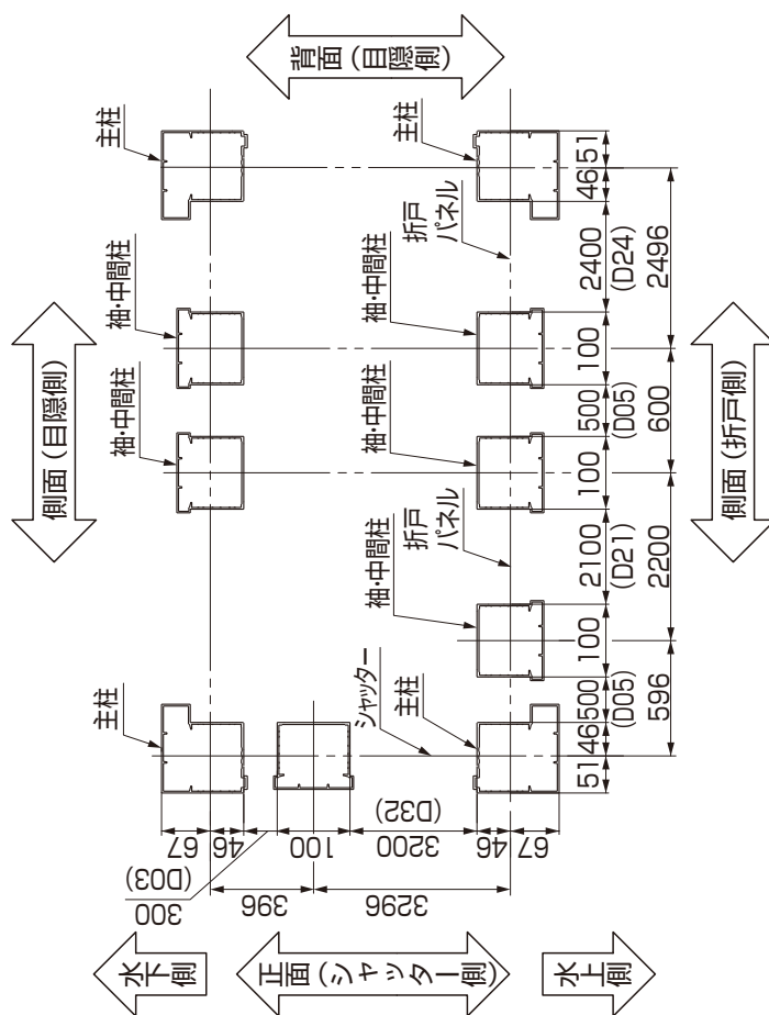
図2-28 柱の位置出し
