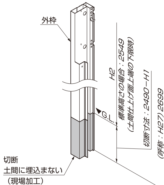
図3-1 外枠の加工
