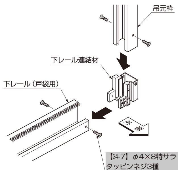
図1-12 吊元枠と下レール(戸袋用)の取付け
