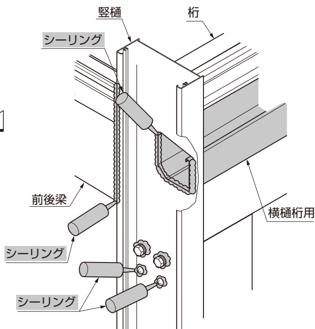
図1-3 縦樋
