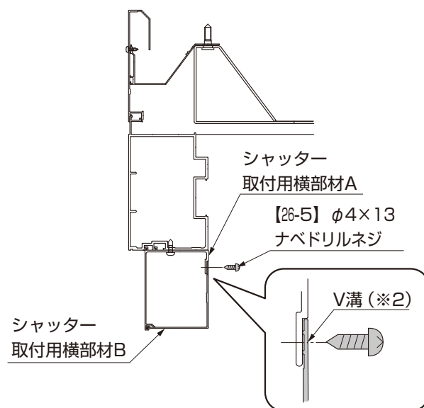
図2-4 シャッター取付用横部材Bの取付け
