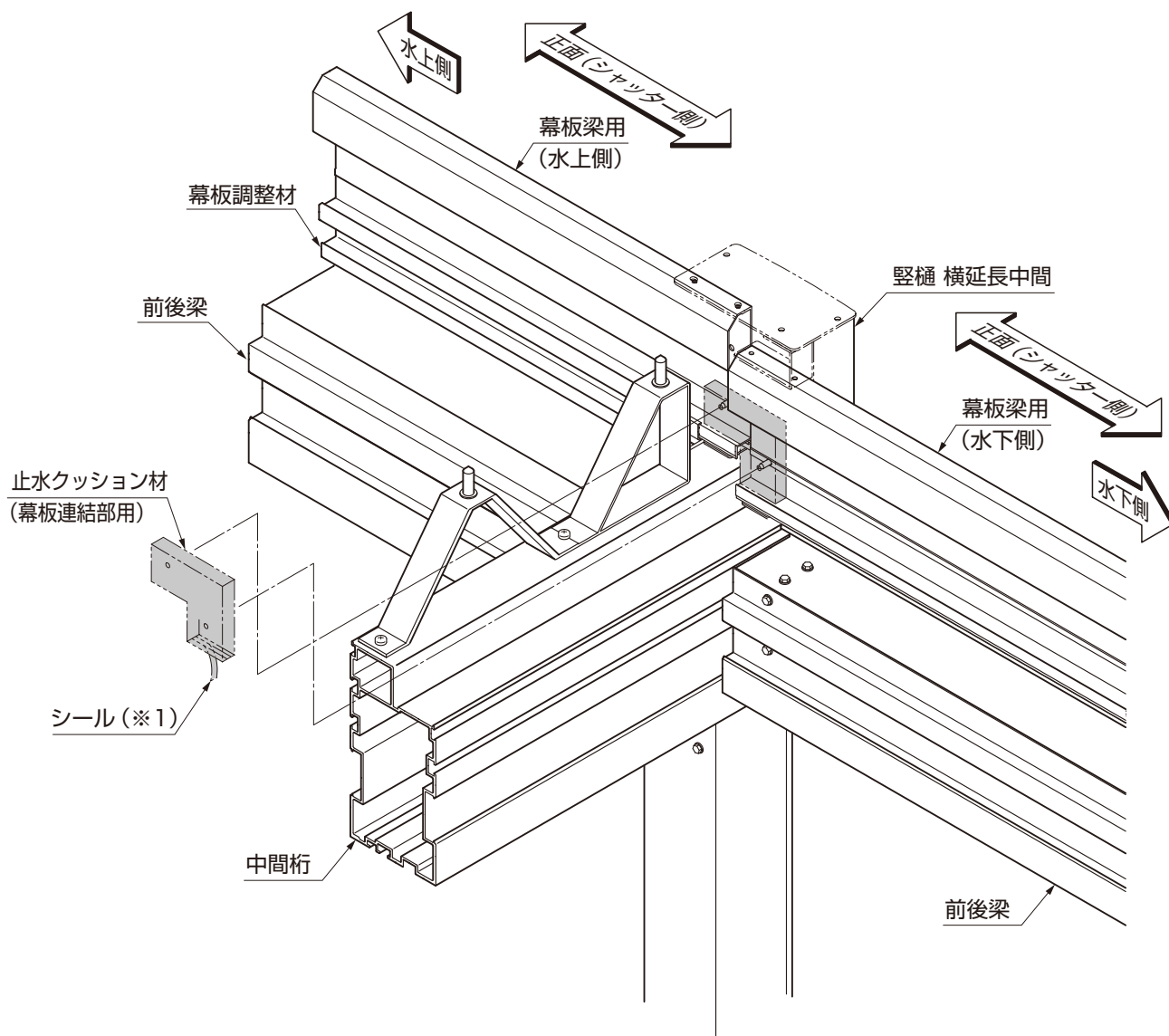
図14-12 止水クッション材(幕板連結部用)の取付け
