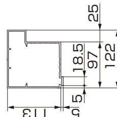
图2-79 主柱扩大图
