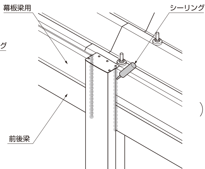
図18-21 中間部のシーリング
