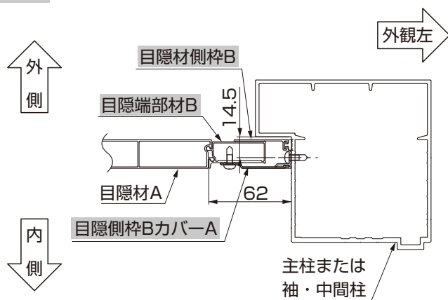
図2-6 部材断面図
