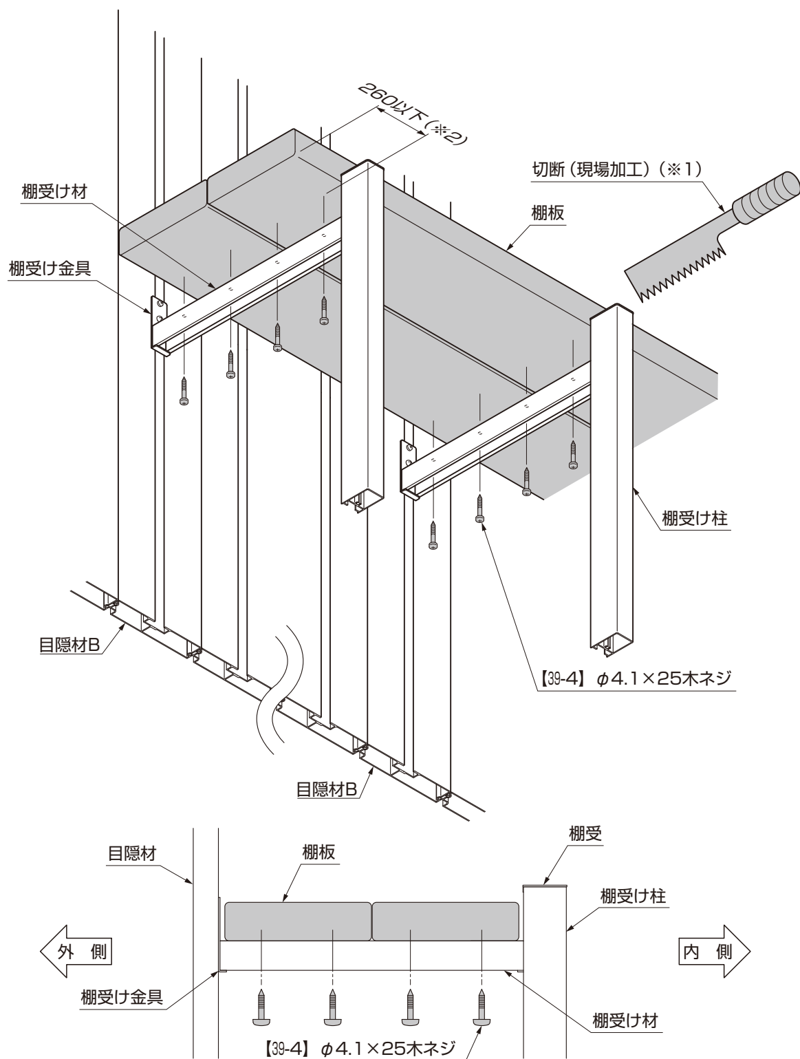
図6-1 棚板の固定
