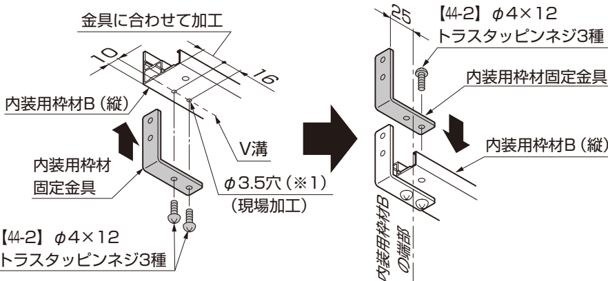
図4-2 内装用枠材固定金具の取付け
