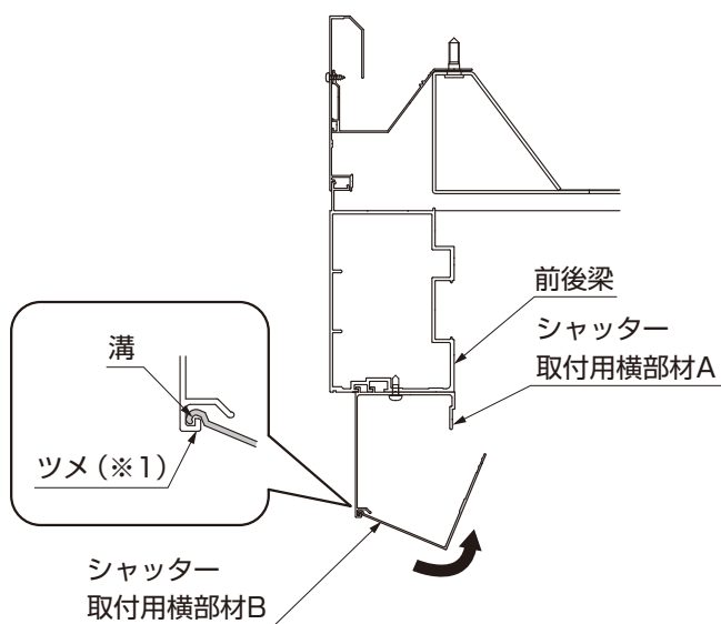
図2-3 シャッター取付用横部材Bの適合
