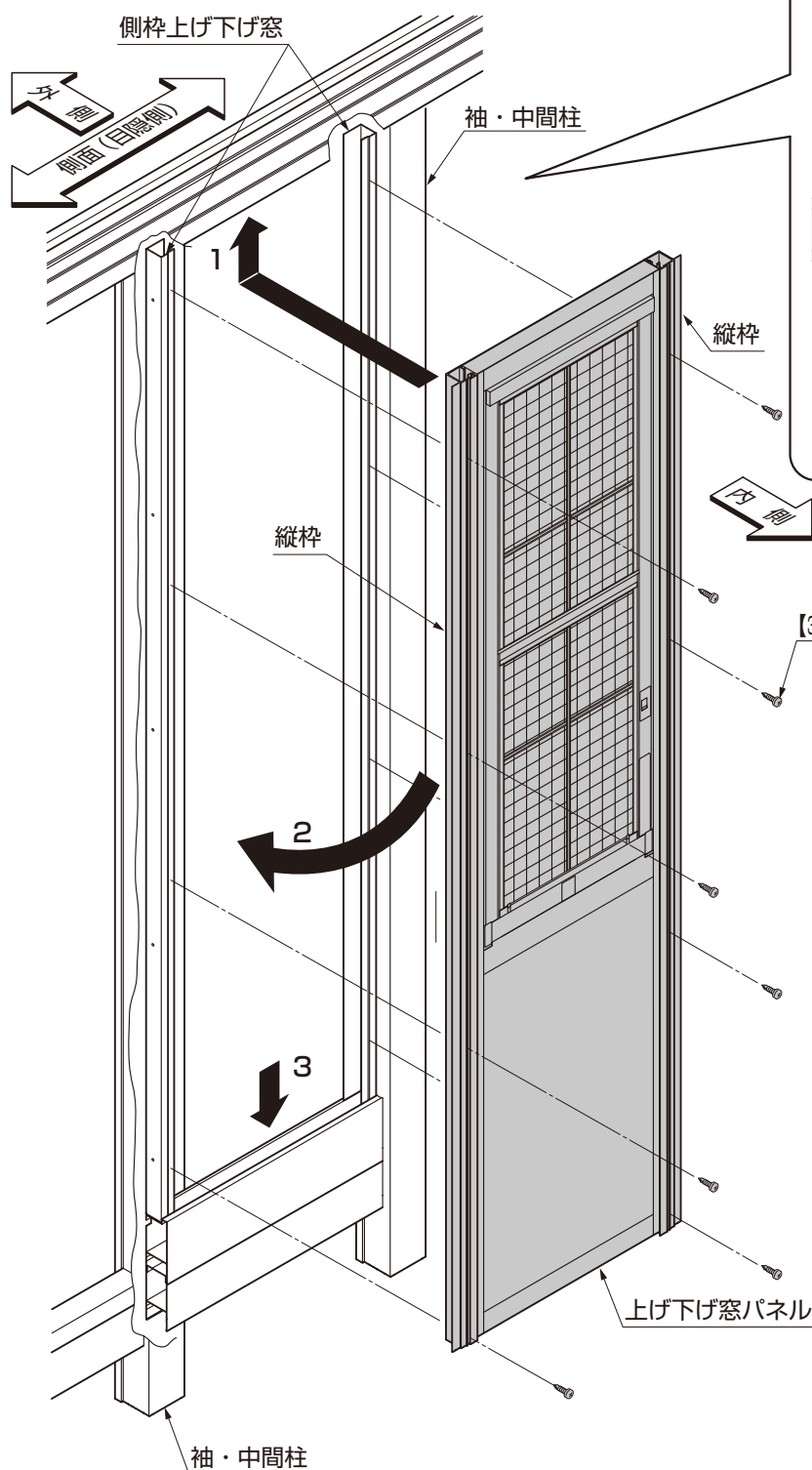
図4-1 上げ下げ窓パネル縦枠の取付け
