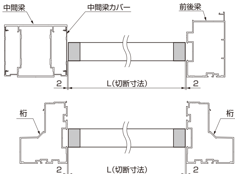
図1-1 桁配線カバーの切断
