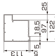
図2-62 主柱拡大図
