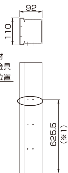
図10-14 袖・中間柱の場合
