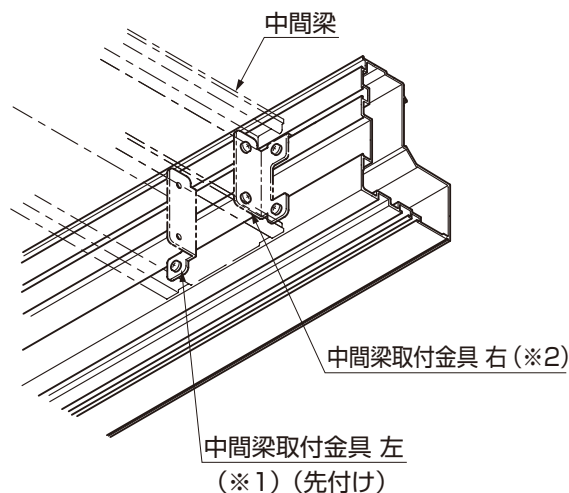
図6-2 中間梁取付金具の取付け位置
