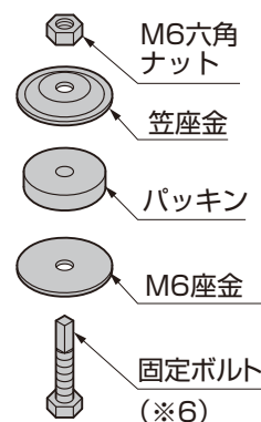
図16-14 中間用折板固定部品
