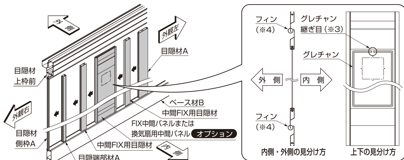
図6-1 目隠材の取付け (FIX中間パネルまたは換気扇用中間パネル オプション )
