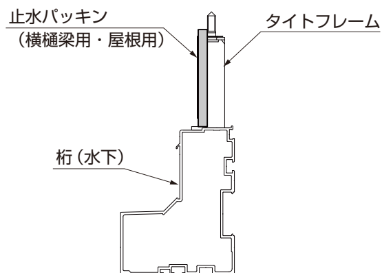
図15-4 桁（水下）の止水パッキンの貼付け位置
