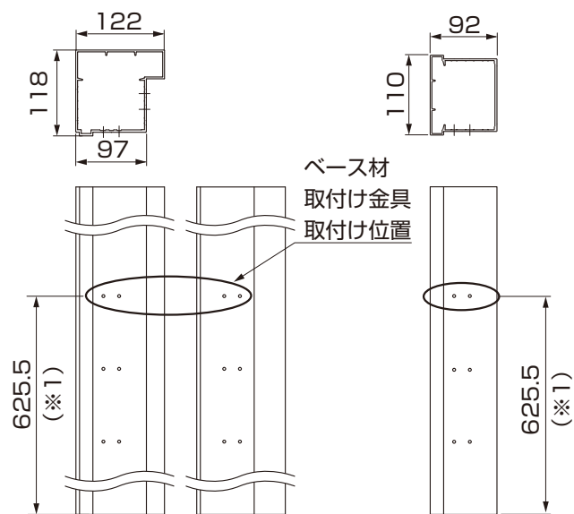
図10-8 主柱の場合
