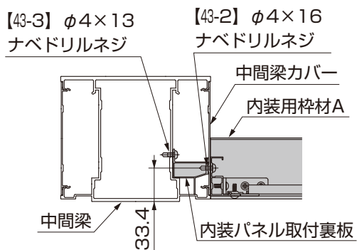
図3-3 中間梁との取合い
