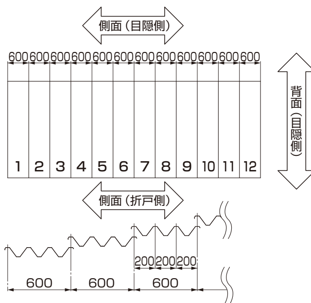
図16-4 L74の場合
