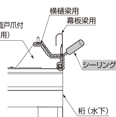
図1-11 (水下側) 端部面戸
