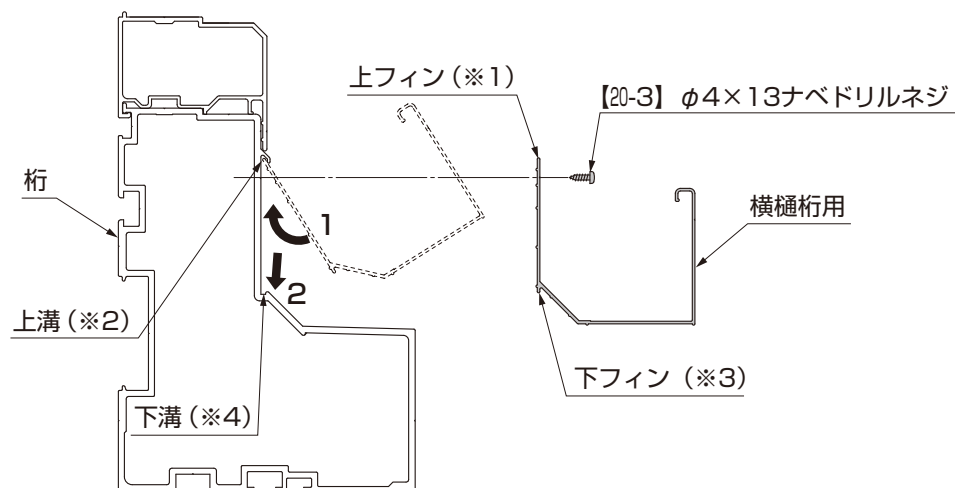
図8-1 横樋桁用の取付け
