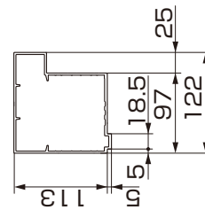
図2-7 主柱拡大図
