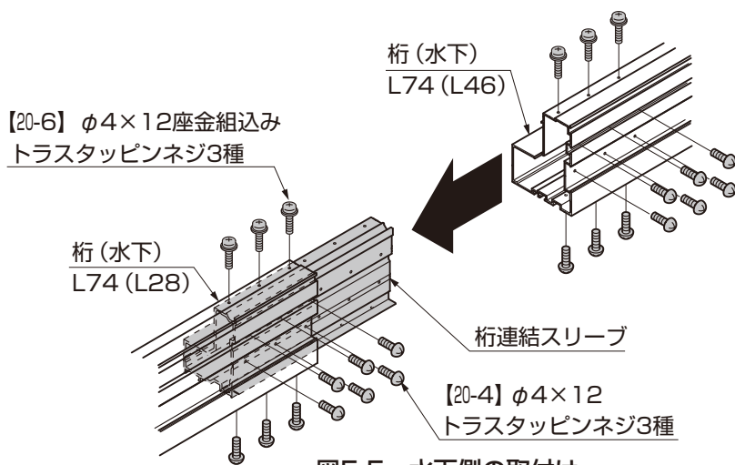
図5-5 水下側の取付け
