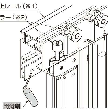
図1-16 A部詳細図
