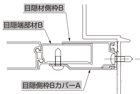
図2-7 目隠端部材B断面図
