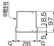
図2-50 ベース材 (目隠・機能・袖)
