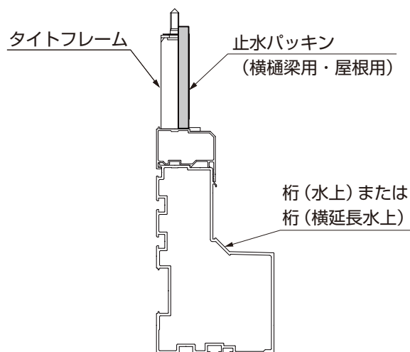
図15-5 桁（水上）の止水パッキンの貼付け位置
