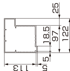
図2-52 主柱拡大図
