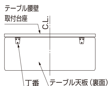
図4-1 丁番の取付け
