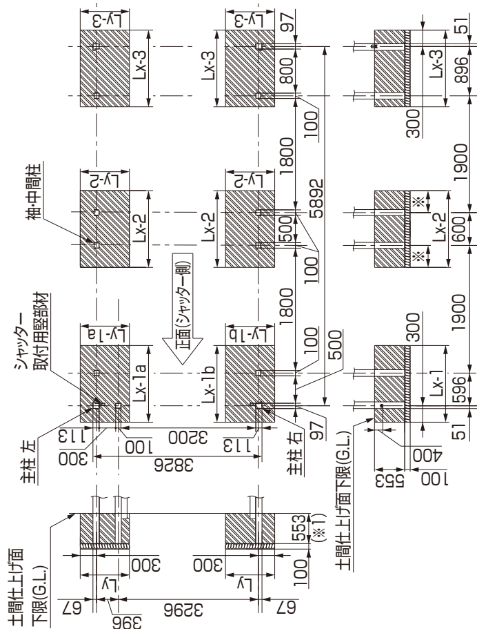
図2-91 基礎寸法 ※=[(Lx-2)-600]/2
