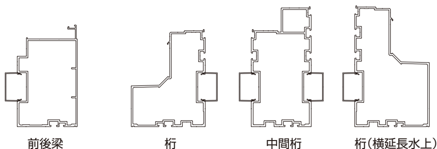
図1-2 桁配線カバーの納まり
