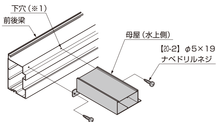
図13-3 母屋の取付け（水上側）
