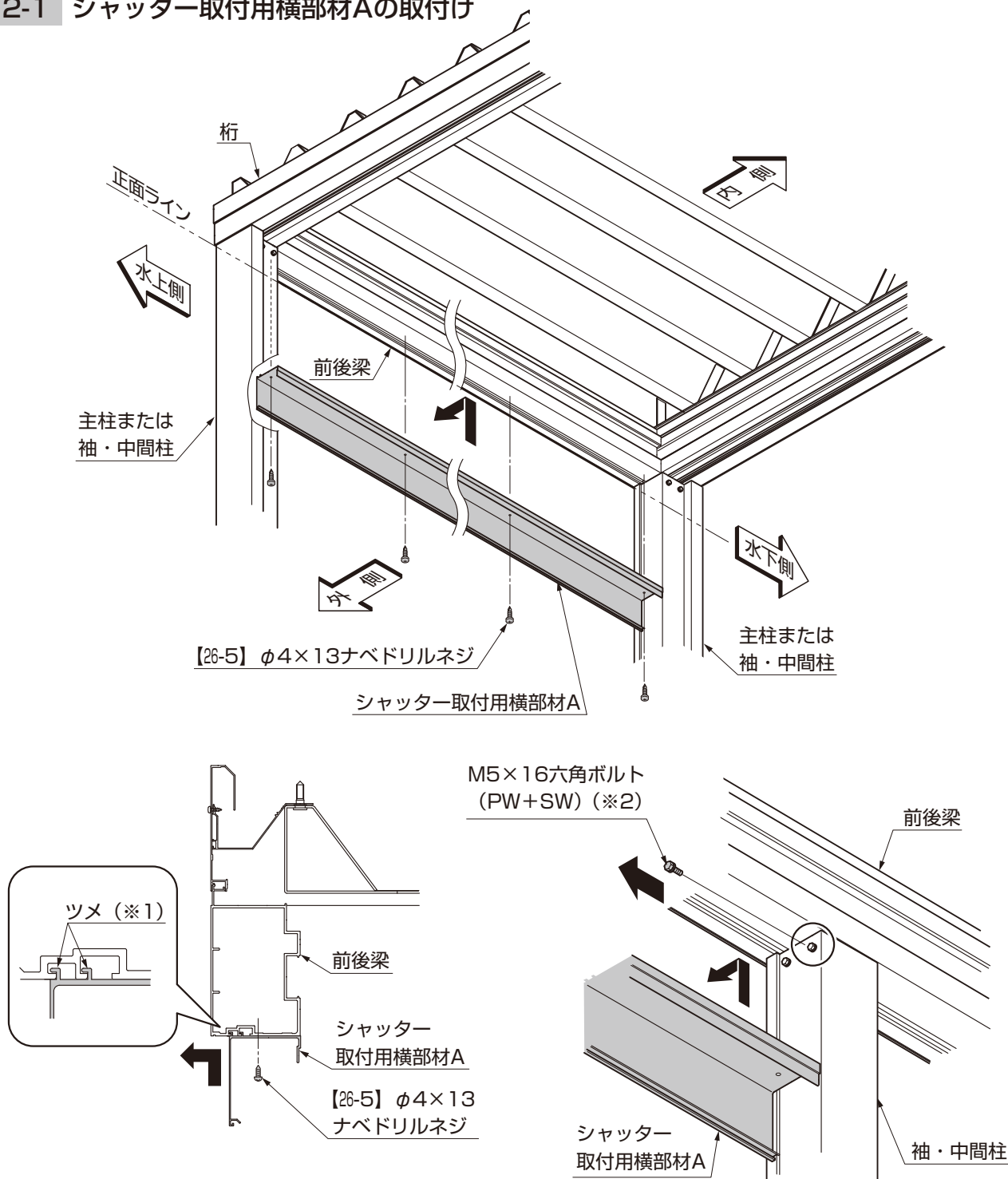
図2-1 シャッター取付用横部材Aの取付け
