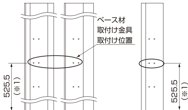
図10-5 主柱の場合
