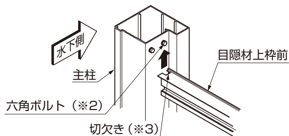
図3-2 目隠材上枠前の六角ボルトの逃げの切欠き
