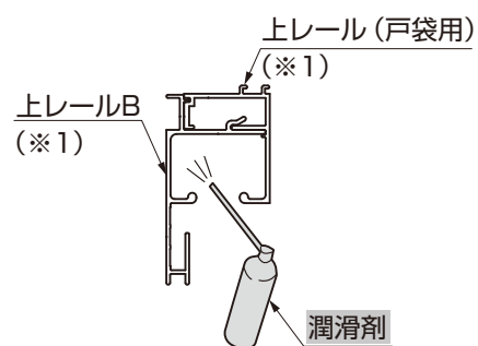
図1-17 潤滑剤の塗布
