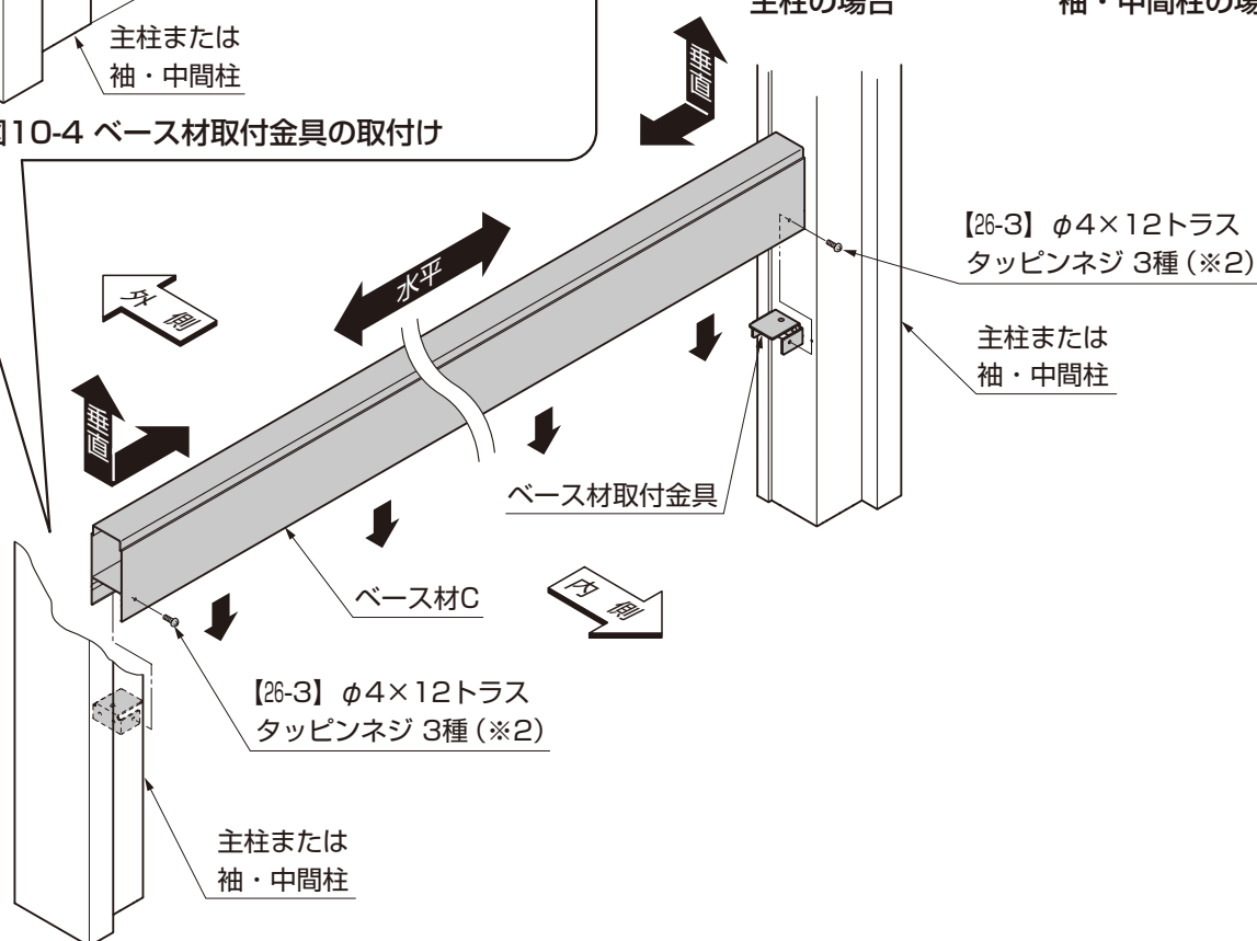
図10-5 主柱の場合
