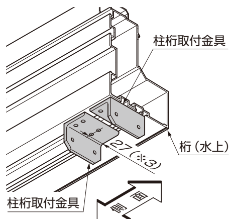
図6-4 A部詳細図 両端部の取付け
