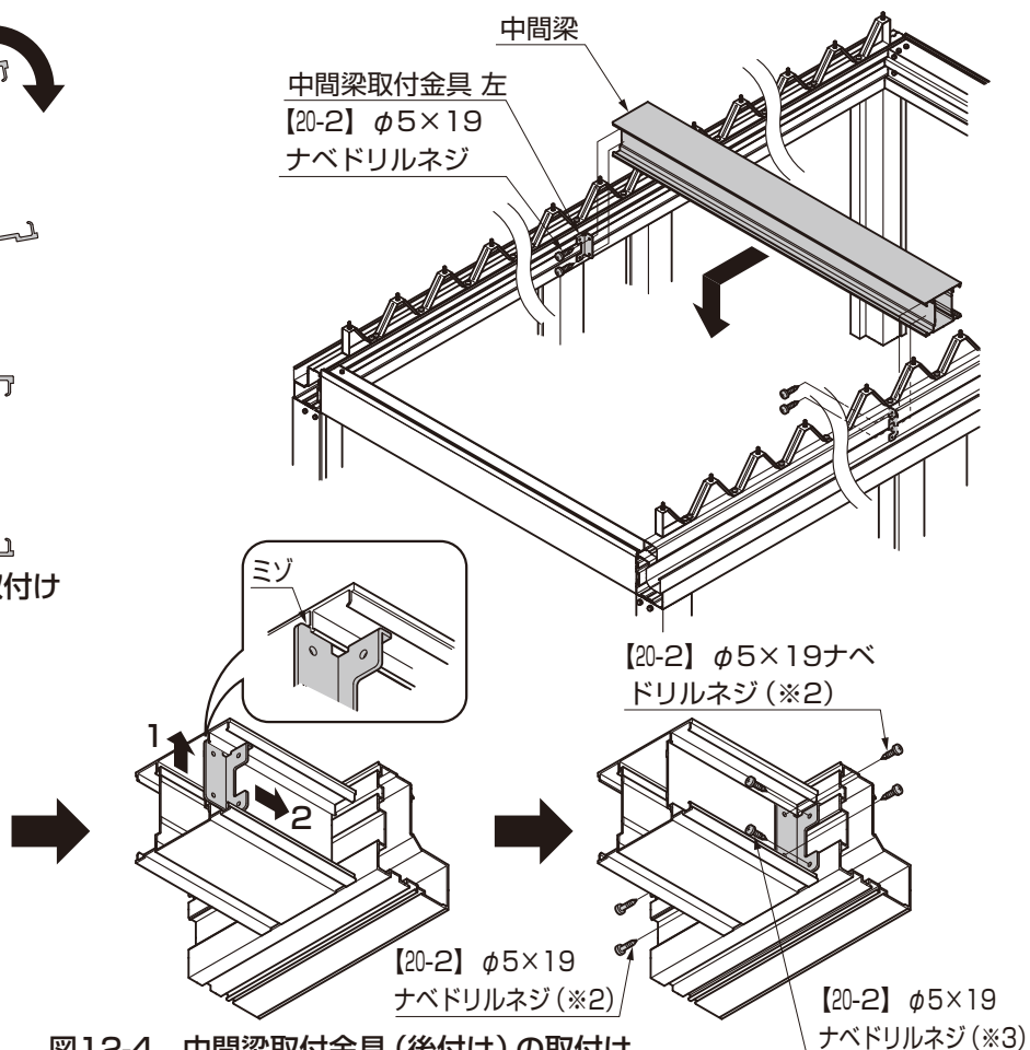
図12-4 中間梁取付金具（後付け）の取付け
