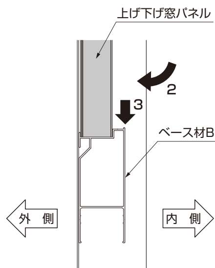
図4-2 上げ下げ窓パネルの落とし込み
