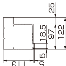
図2-25 主柱拡大図
