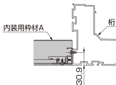
図3-5 桁との取合い
