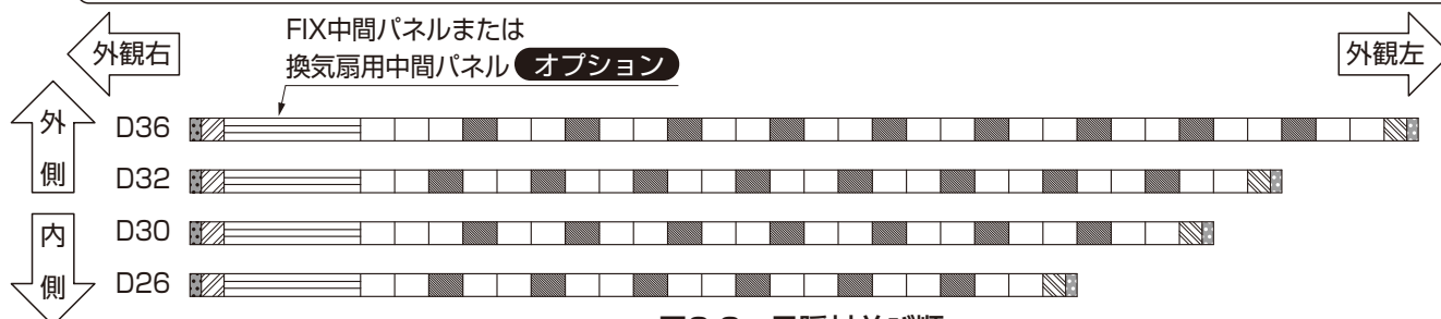
図2-2 目隠材並び順
