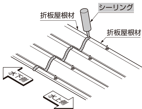
図1-7 横樋用 (縦延長・縦横延長の場合)
