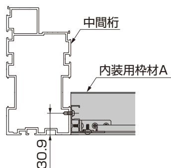
図3-4 中間桁との取合い
