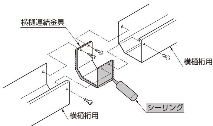
図1-7 横樋用 (縦延長・縦横延長の場合)
