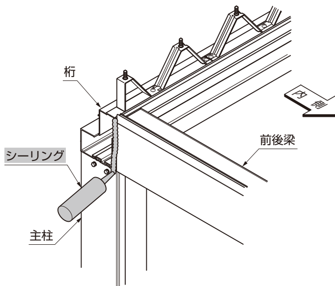
図1-2 桁・前後梁
