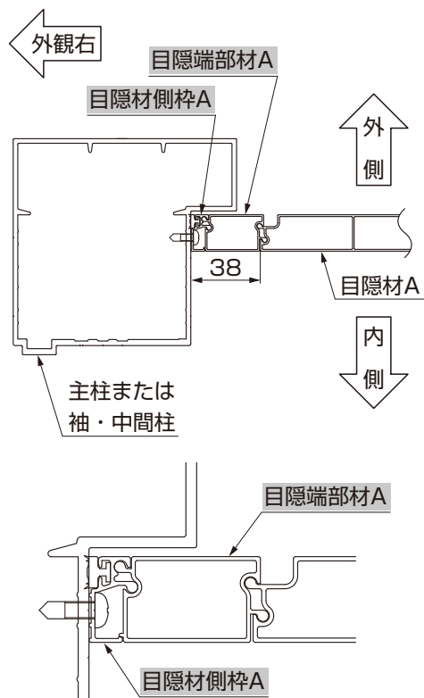
図2-3 目隠端部材A断面図
