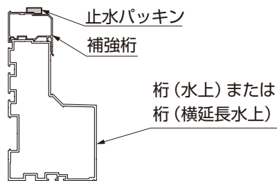
図7-3 補強桟の止水パッキンの貼付け位置
