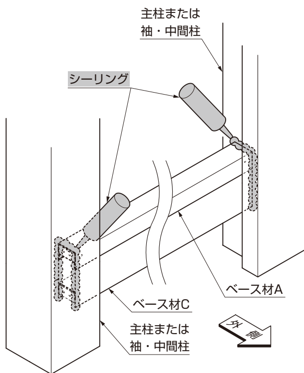
図1-5 ベース材 (折戸)
