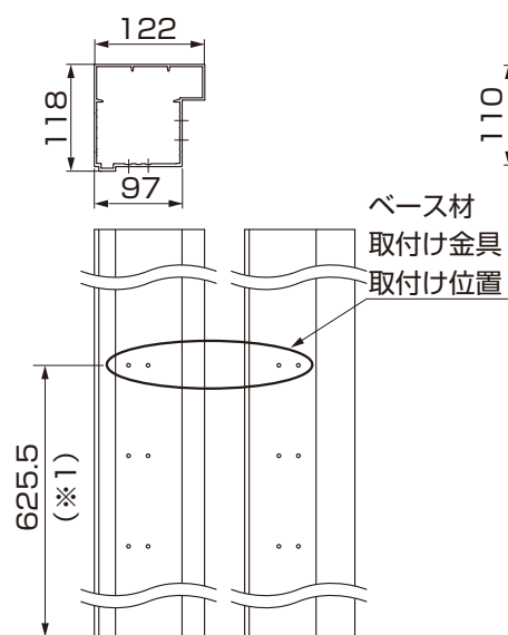
図10-13 主柱の場合
