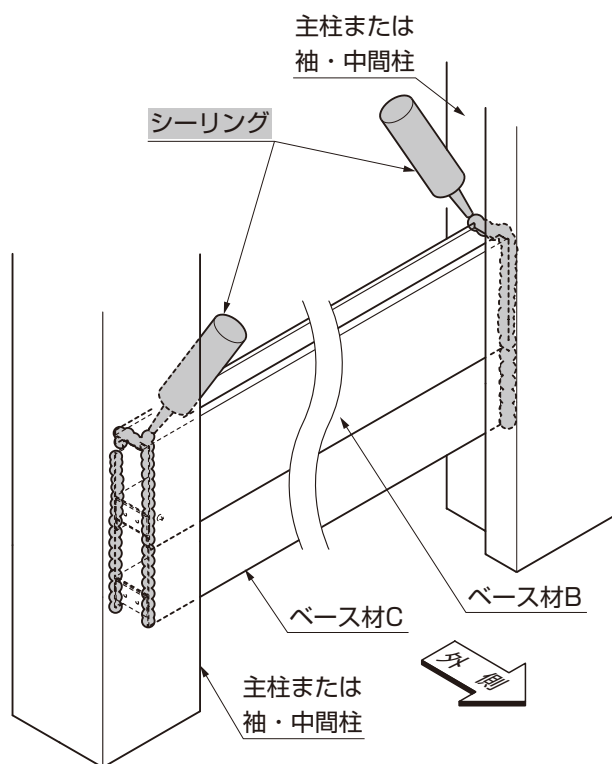
図1-4 ベース材 (目隠)
