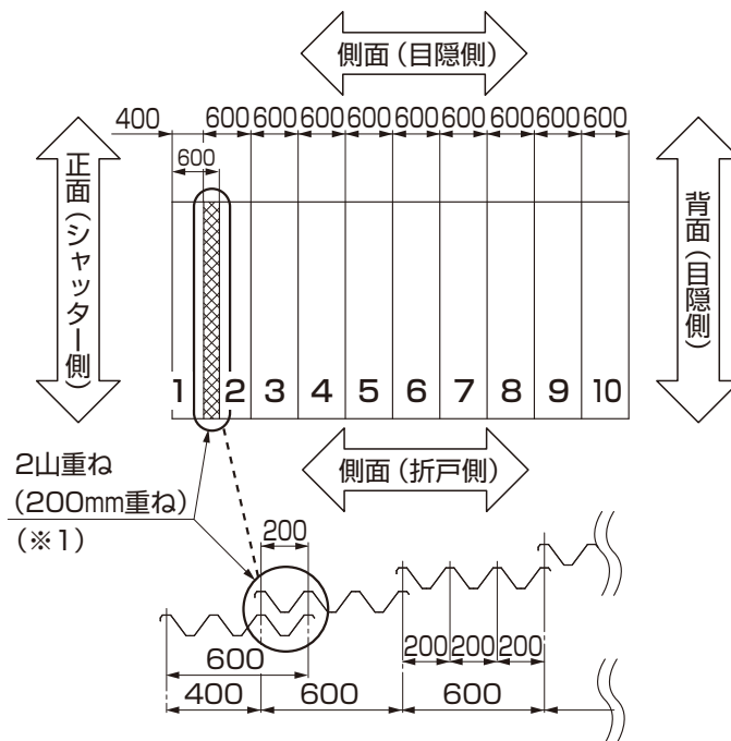
図16-2 L60の場合
