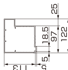
図2-43 主柱拡大図
