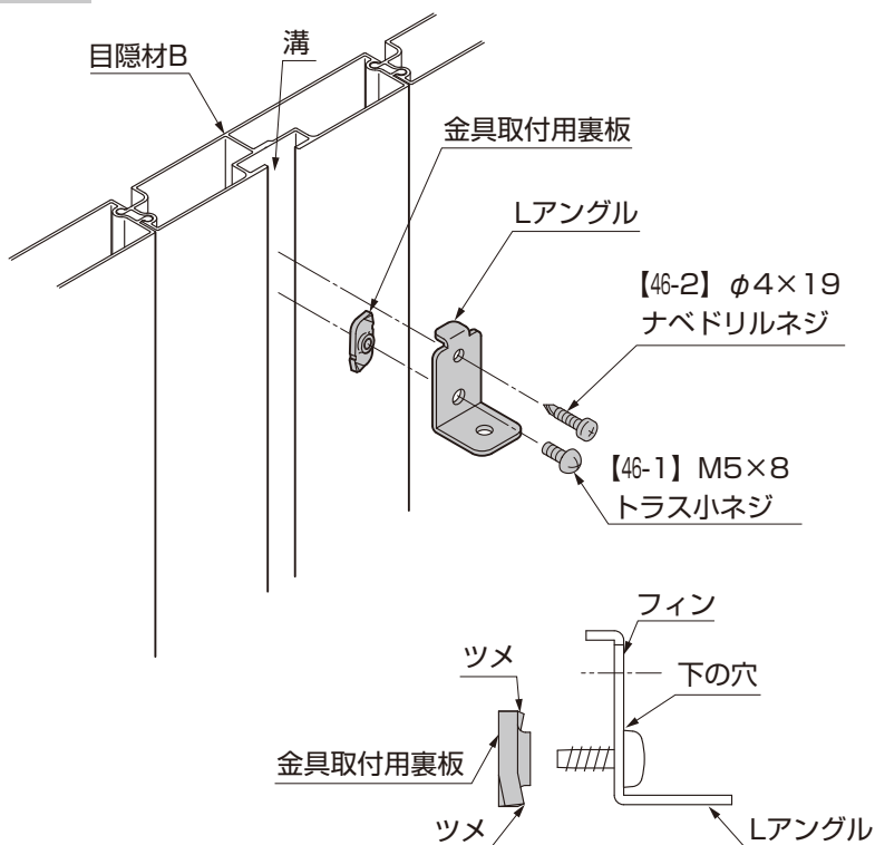
図9-1 Lアングルの取付け
