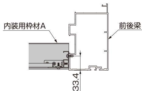
図3-5 前後梁との取合い
