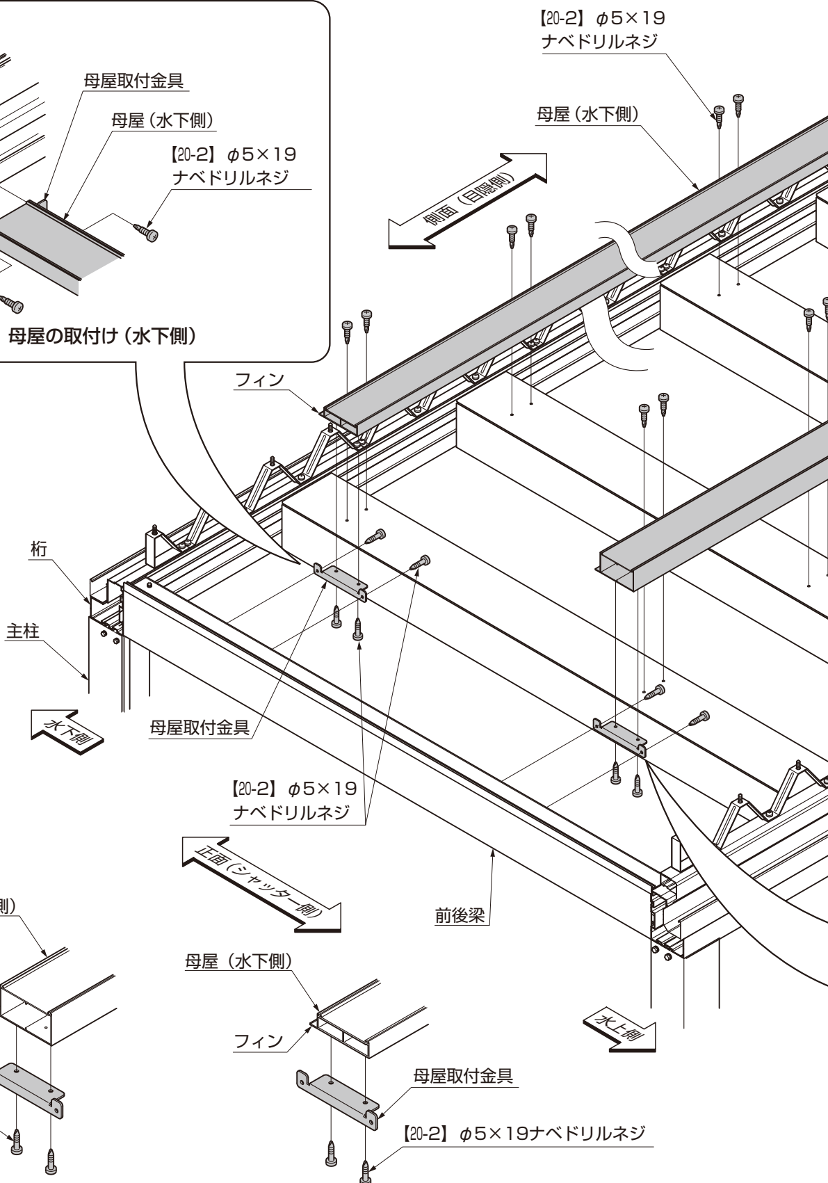
図13-1 母屋取付金具の取付け (水上側)
