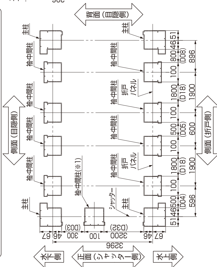
図2-90 柱の位置出し
