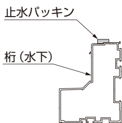
図7-2 桟（水）の止水パッキンの貼付け位置
