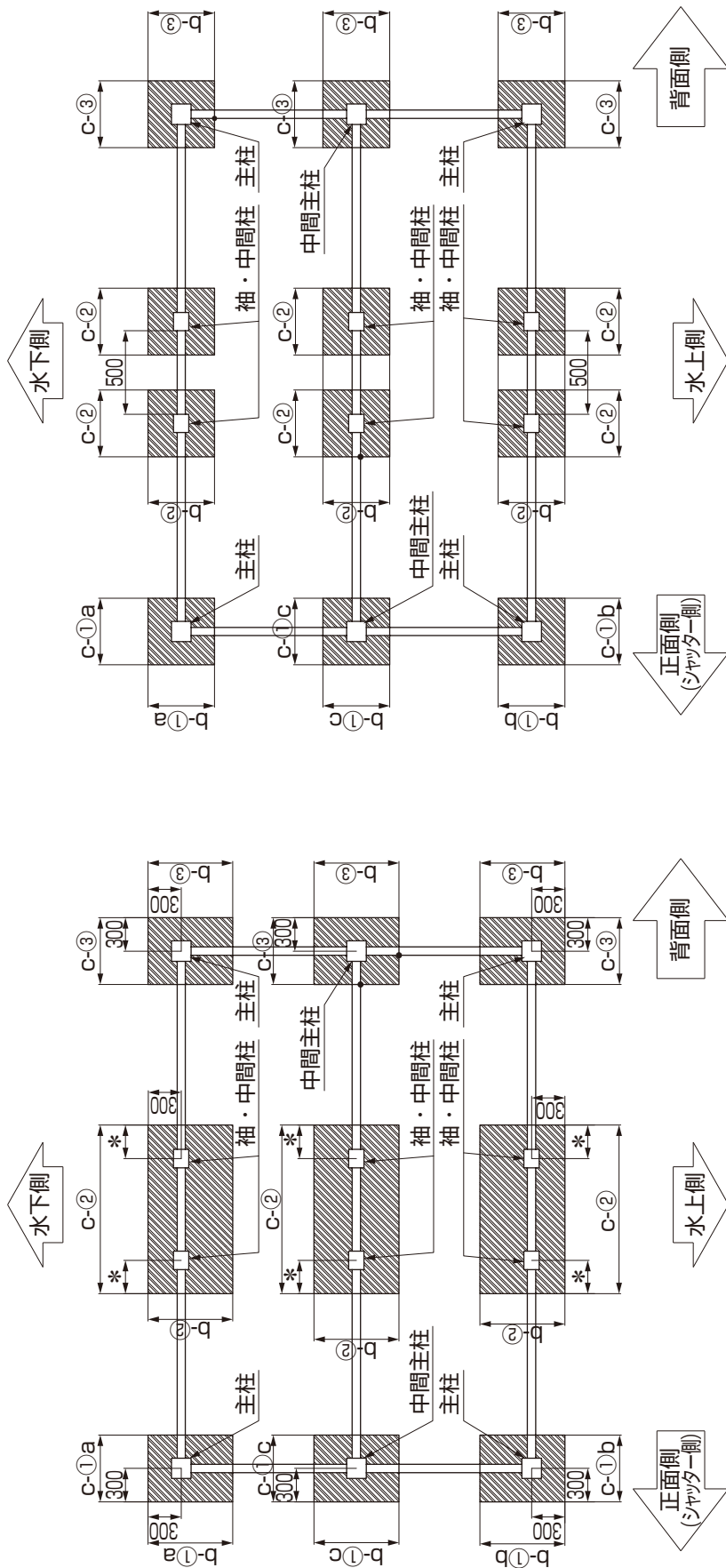
図2-47 基礎寸法 ※ =[(c-2-600)]/2
