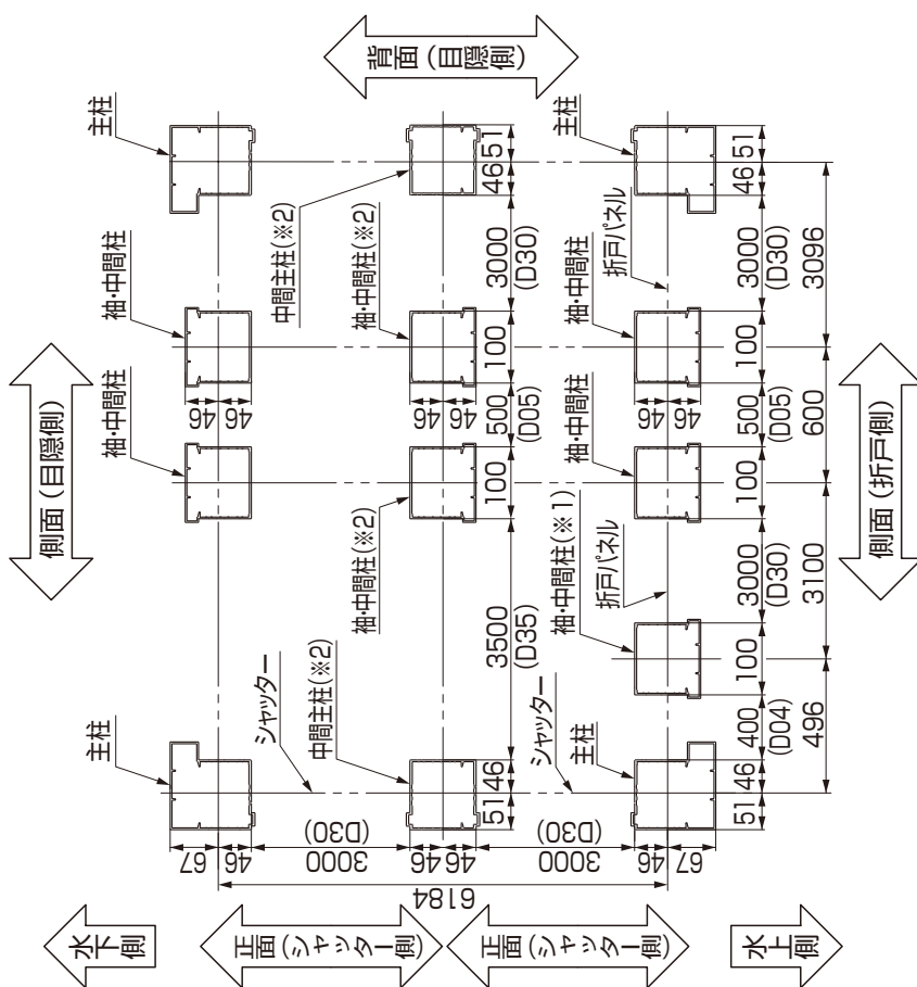
図2-56 柱の位置出し
