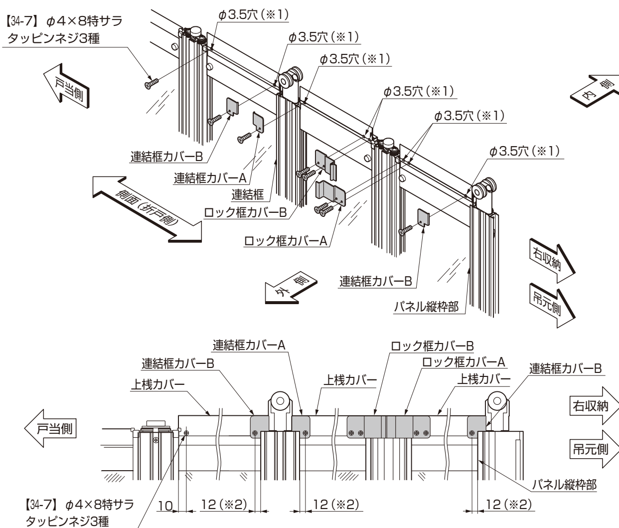
図7-2 上棧カバーと框カバーの取付け
