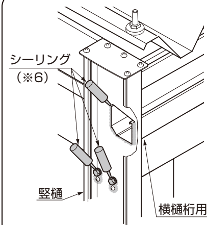
図18-18 端部のシーリング
