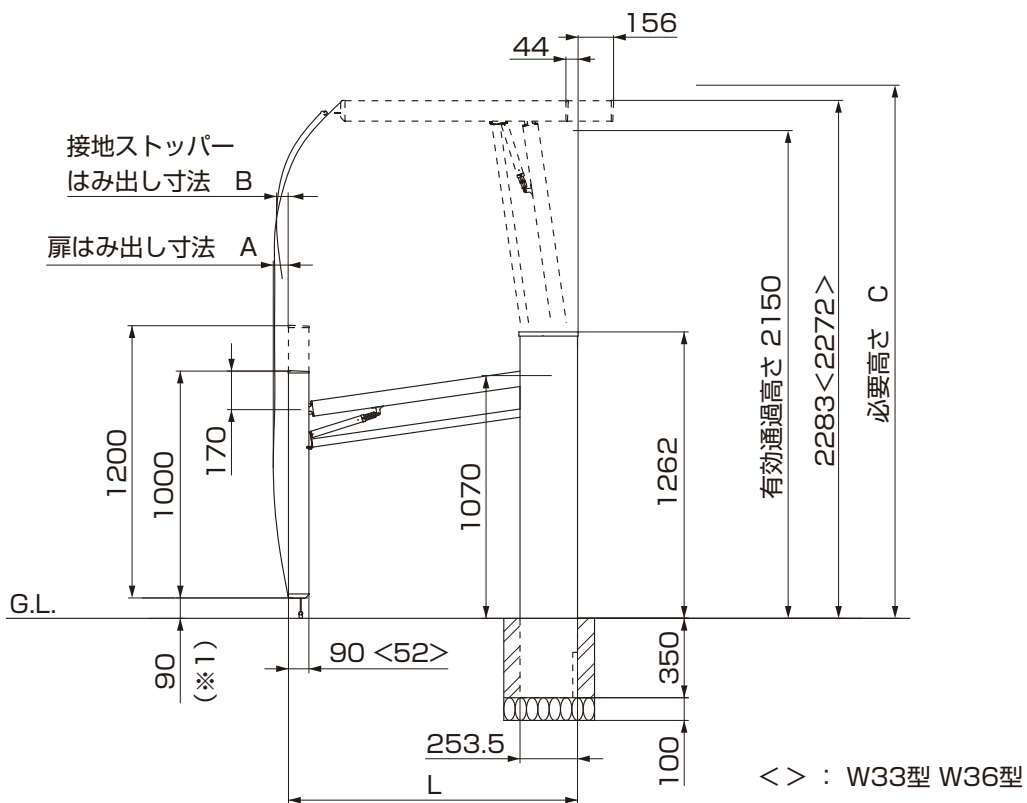
図2-12 側面図（ハイルーフの場合）
