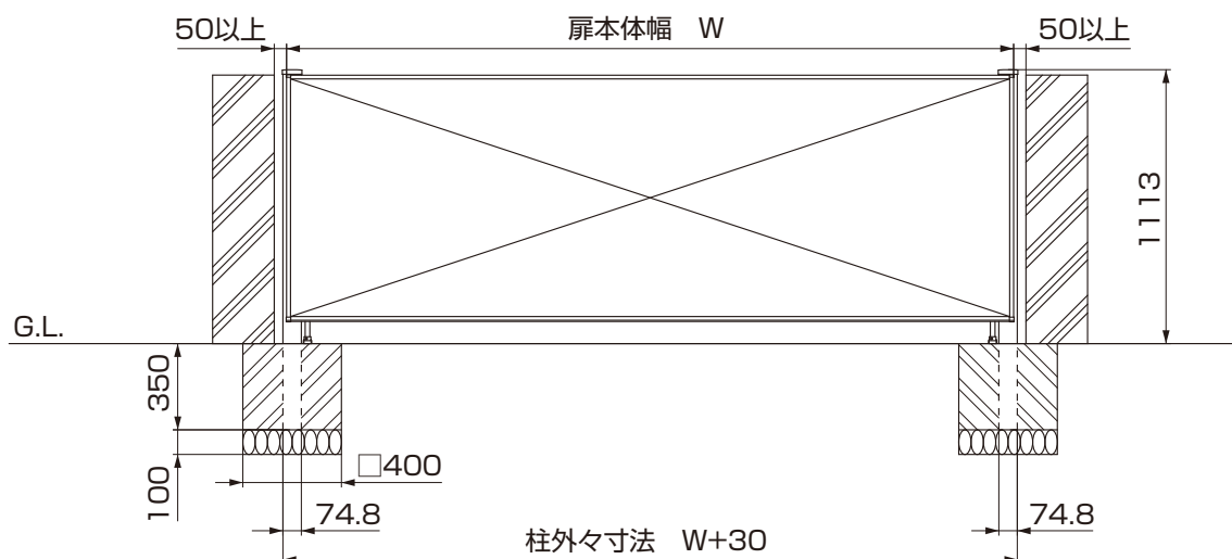
图2-10 正面图
