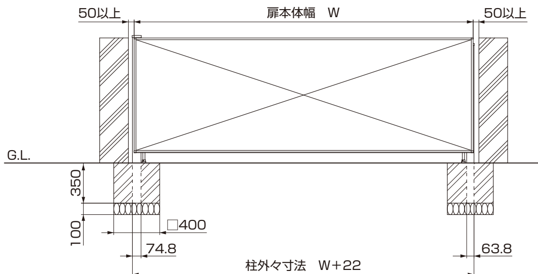
図2-6 正面図
