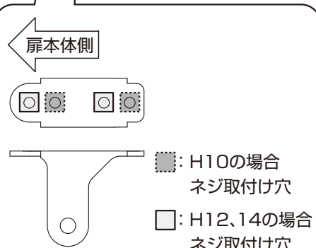
図5-1 補助スプリング取付金具詳細
