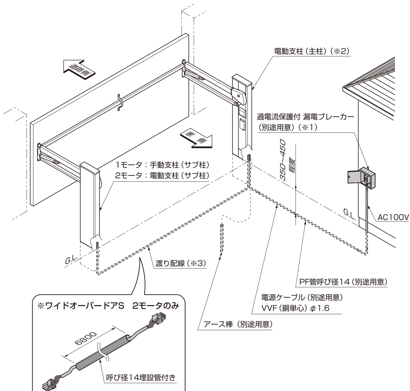
図4-1 渡り配線 (左右はありません)
