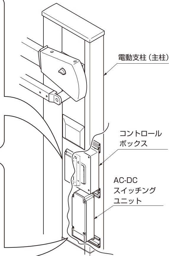
図1-1 A部詳細図
