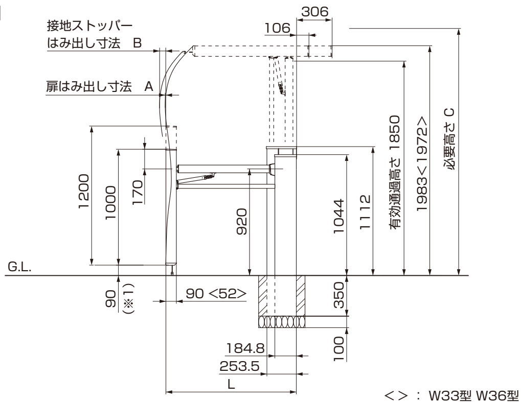
図2-7 側面図 (標準の場合)
