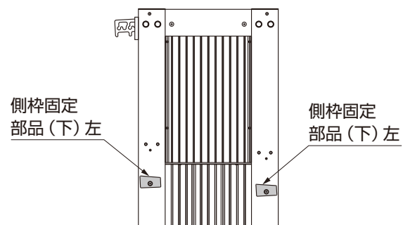
図5-2 1台用柱左
