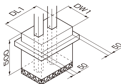
図4-3 土間コンクリート併用基礎の場合
