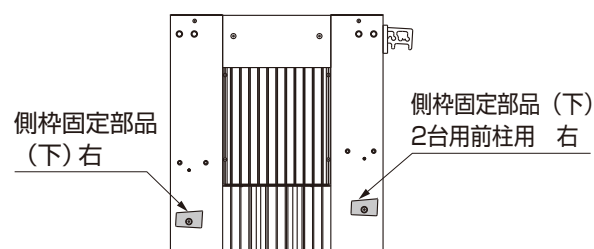
図5-3 2台用柱 右
