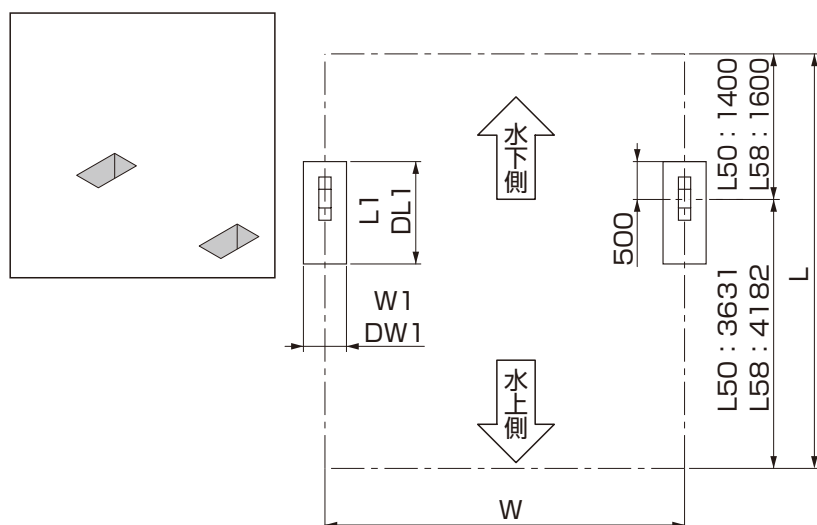
図4-1 基礎位置
