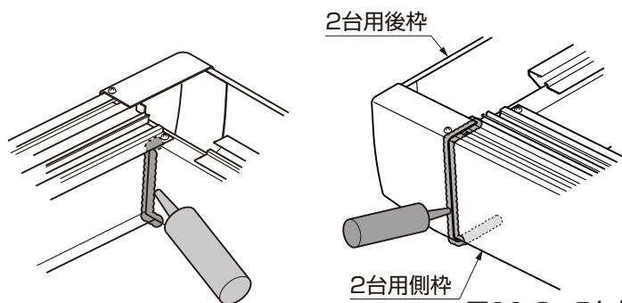
図11-2 B矢視図
