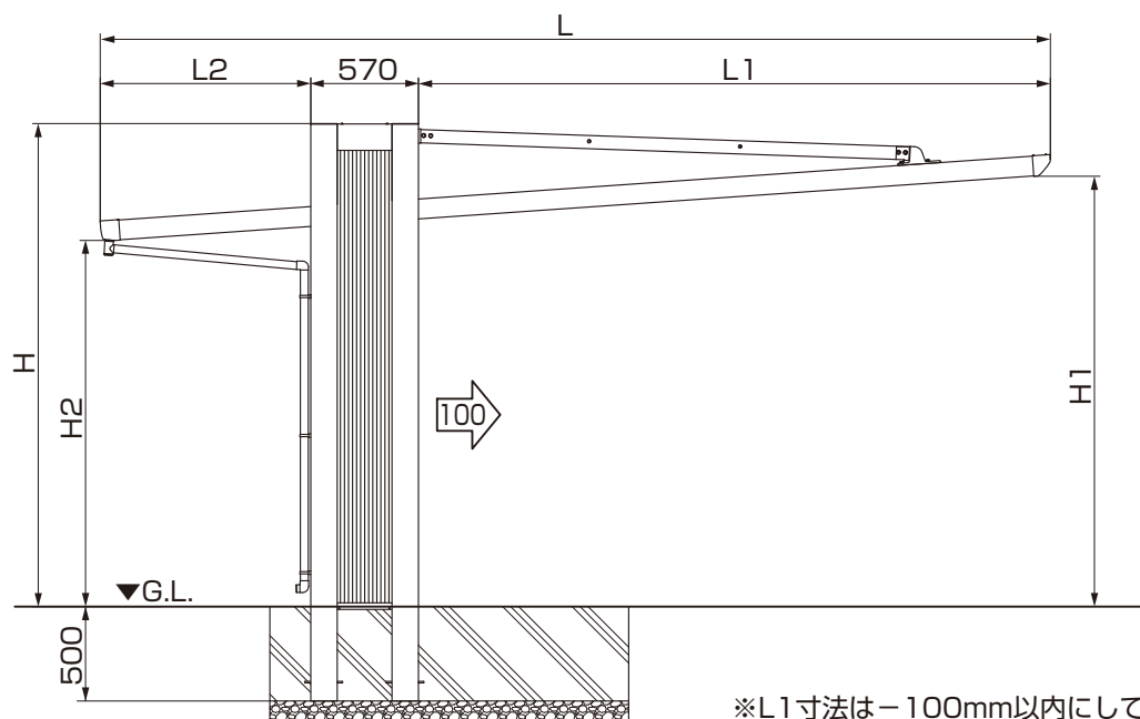
図3-1 側面図
