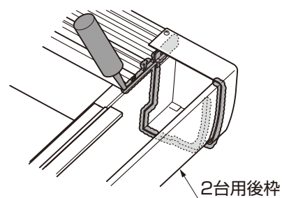
図11-3 C矢視図
