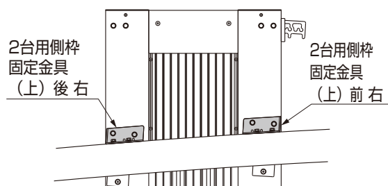
図7-2 2台用柱 右
