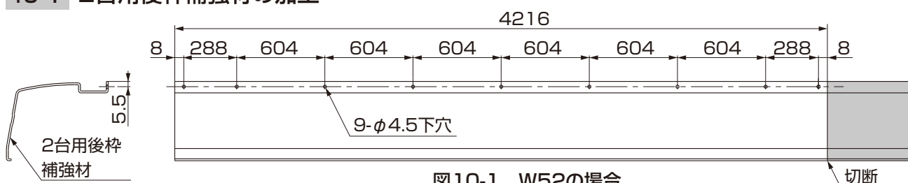
図10-1 W52の場合
