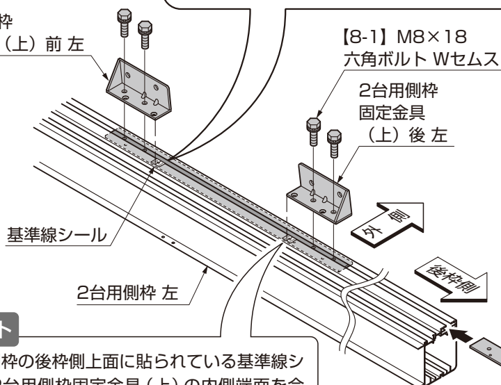
図7-1 基準線シール張付け位置
