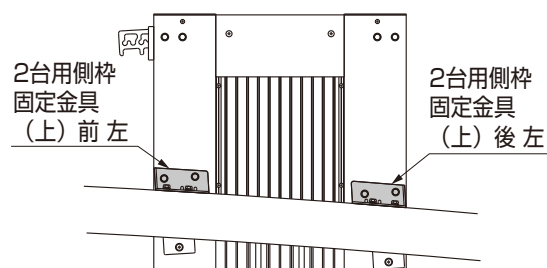
図7-3 2台用柱 左
