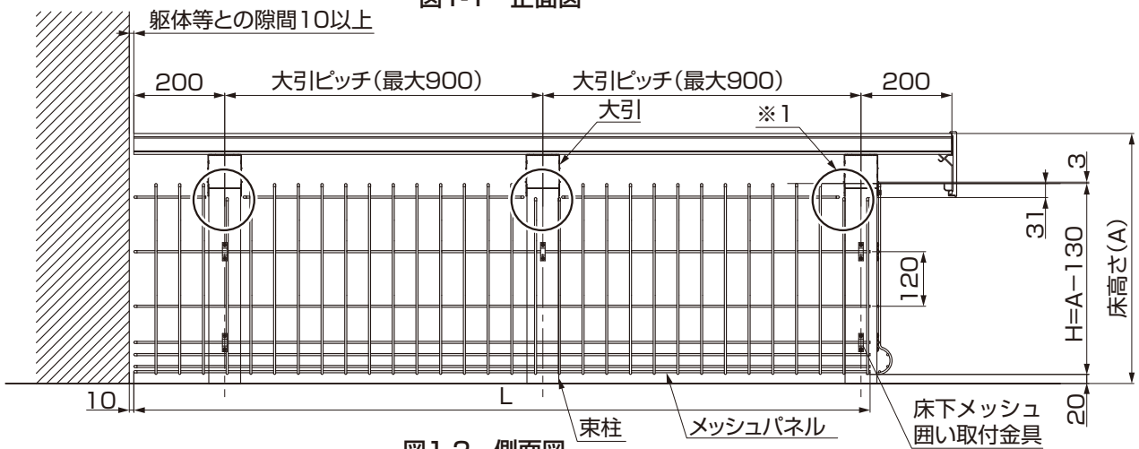
図1-2 側面図
