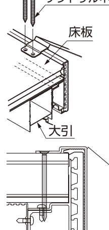
図4-10 大引で固定する場合
