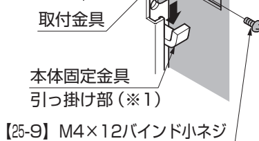
図5-2 A部詳細図
