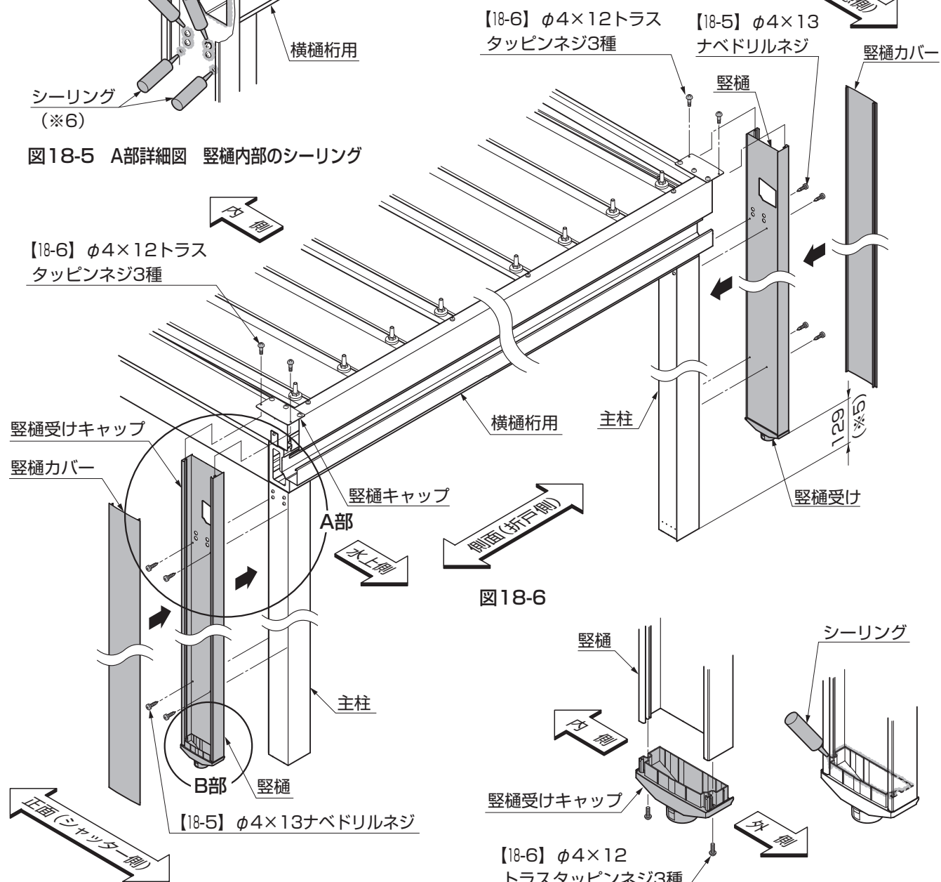
図18-7 B部詳細図 縦樋キャップの取付け
