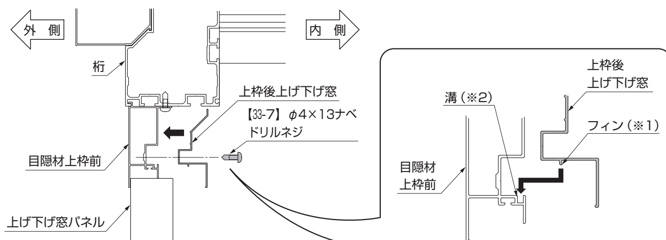
図5-1 上枠後上げ下げ窓の取付け
