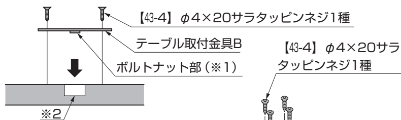
図3-1 ボルトナット部の勘合
