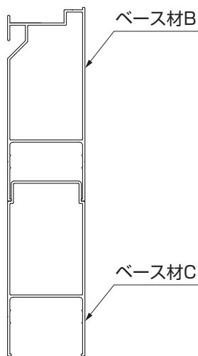
図2-34 ベース材 (目隠・機能柱・袖)
