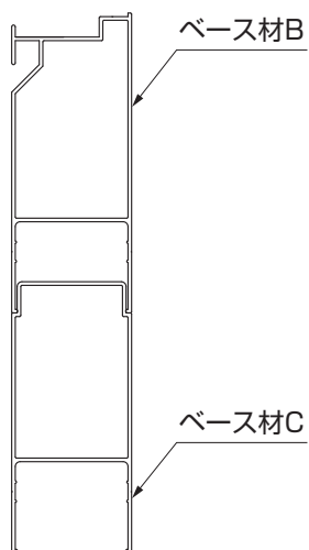
図2-24 ベース材 (目隠・機能柱・袖)
