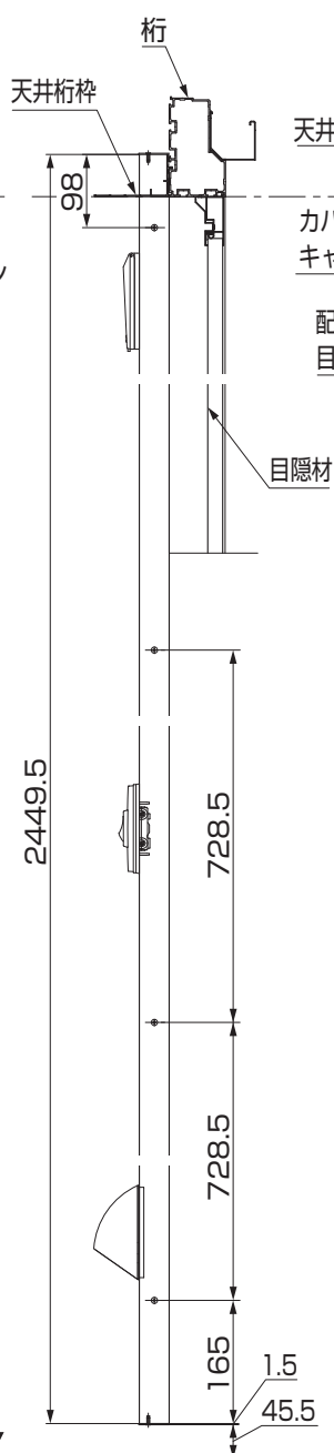
図2-4 A-A断面図 配線カバー中間柱
