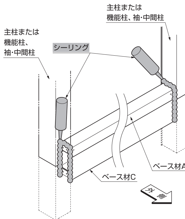
図1-4 折戸パネルベース材（折戸）
