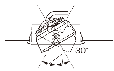
※B部：照射角度の調整
