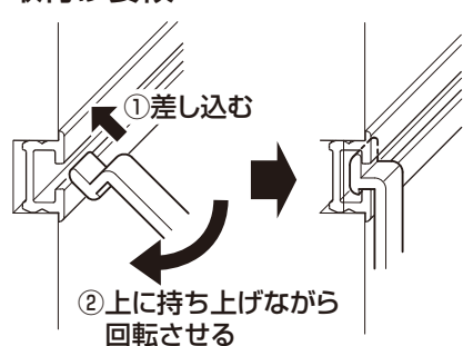
棚受け
