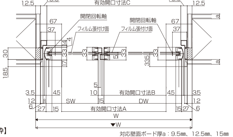
横断面図
