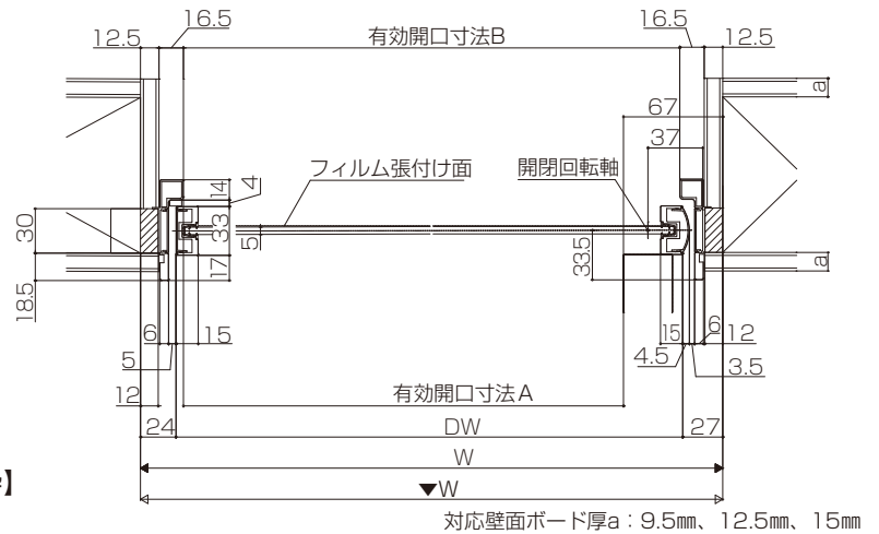
横断面図
