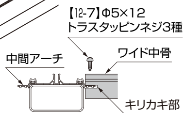
図8-3 ワイド中骨の場合
