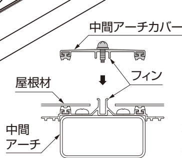
図9-3 中間アーチ断面図
