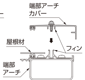
図9-4 端部アーチ断面図
