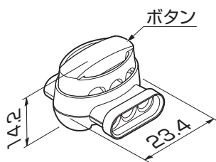
配線接続【前】
