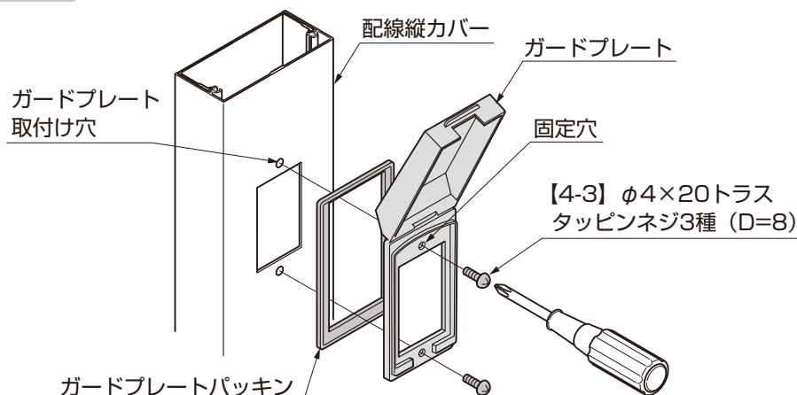
図4-7 ガードプレートの取付け
