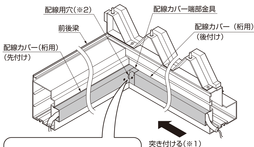
図3-2 配線カバー（桁用）入隅の納まり
