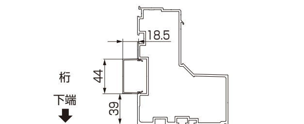
図3-1 間口断面図（標準・縦延長）
