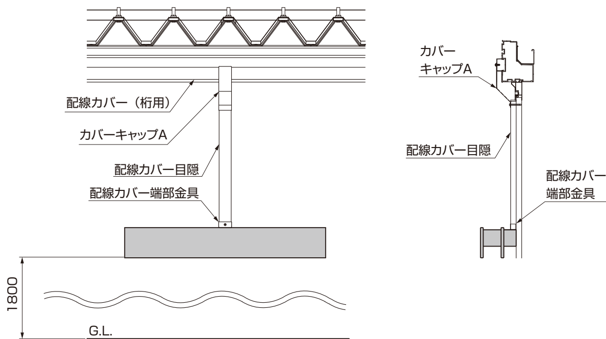
図3-7 G.L.+1800に取付けの場合
