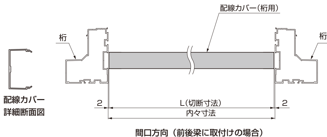
図1-3 配線カバー（桁用） 天井なしの場合の切断
