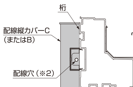
図4-5 配線縦カバーの穴加工
