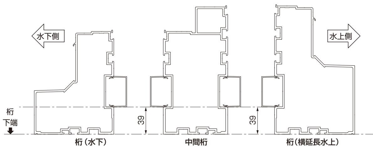
図3-4 間口断面図 (横延長・縦横延長の場合)
