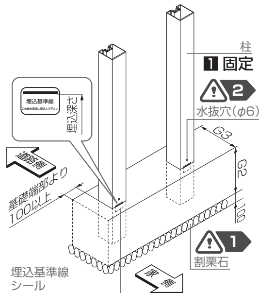
▲ 連続基礎の場合 ▲
