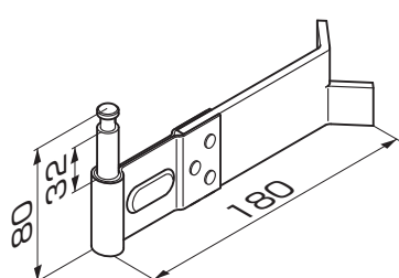
図1-2 AUS、AUW姿図
