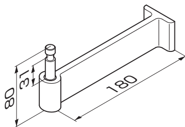
図1-3 VUS、VUW姿図
