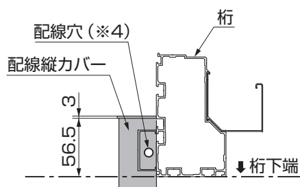
図4-3 配線縦カバーA・Dの穴加工
