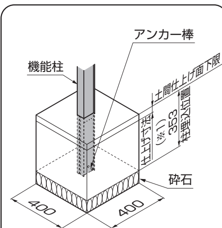
図2-7 機能柱の場合
