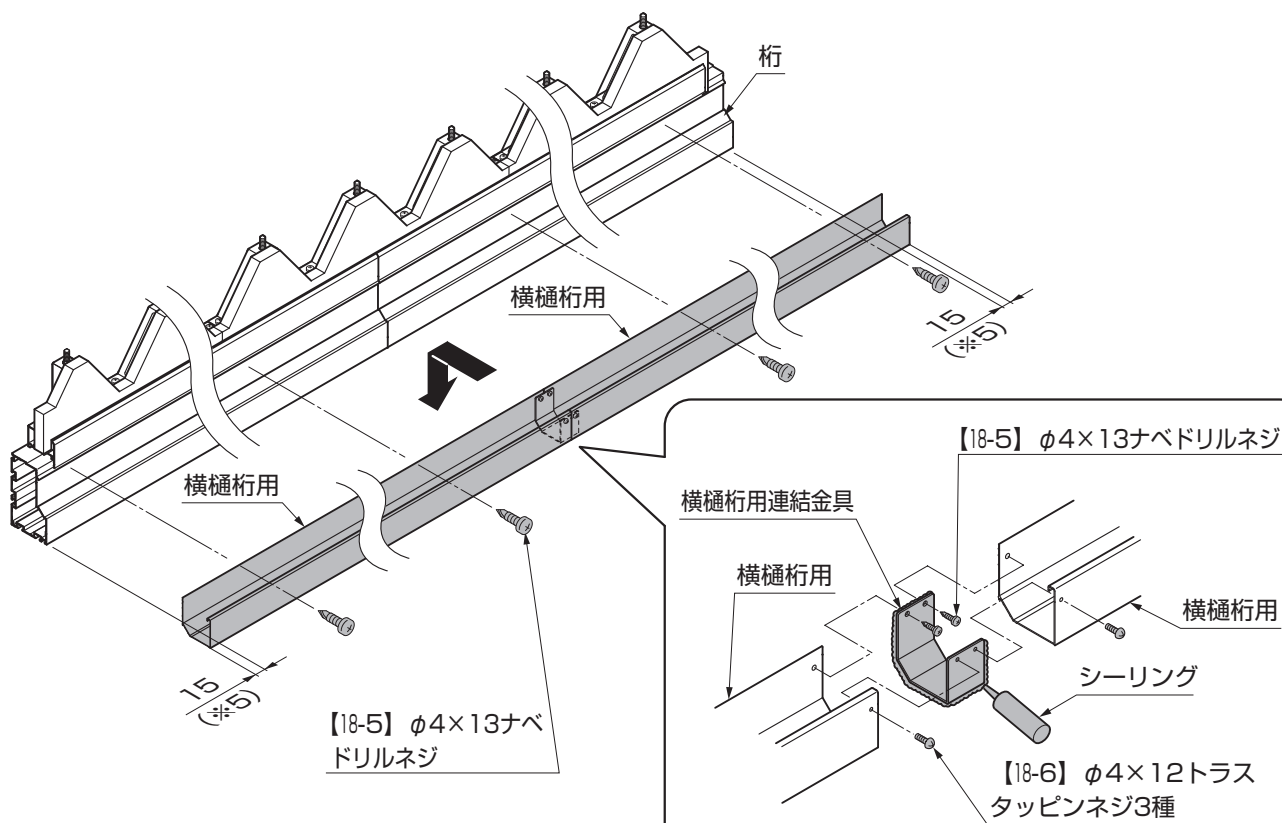
図9-3 横樋桁用の連結
