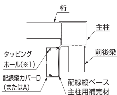
図4-1 天井なし
