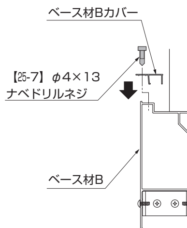
図8-3 ベース材Bカバー取付断面図
