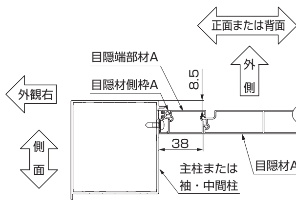
図2-5 正面・背面の場合
