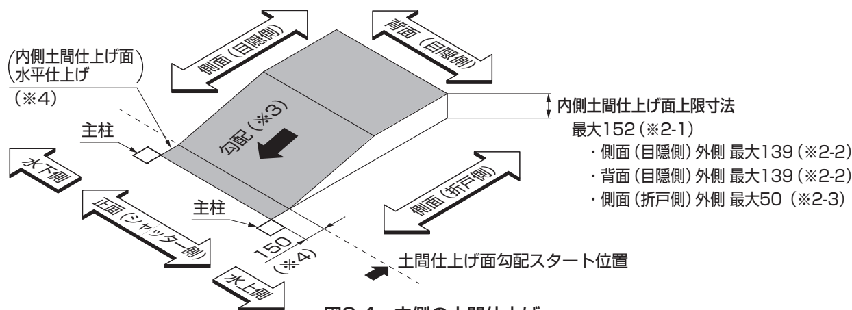
図2-4 内側の土間仕上げ
