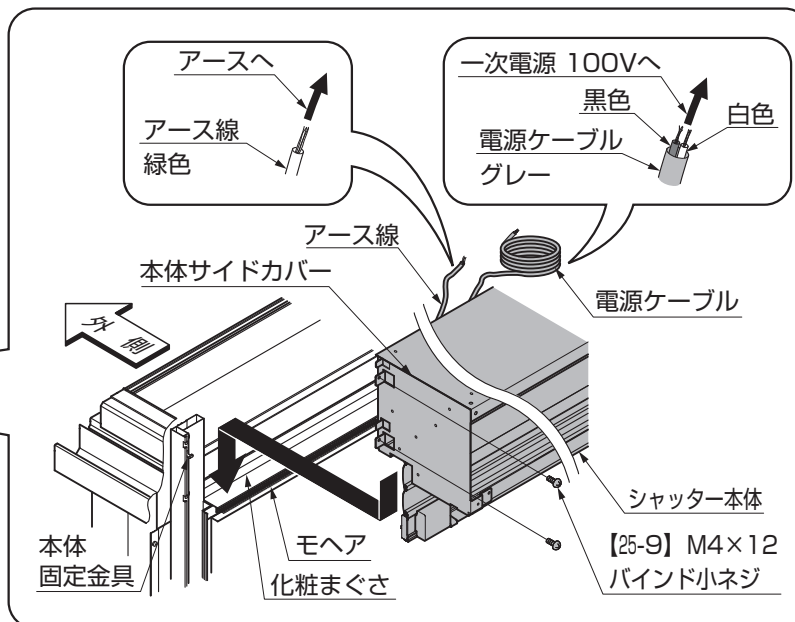
図5-1 シャッター本体の取付け
