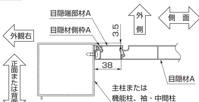
図2-4 側面の場合
