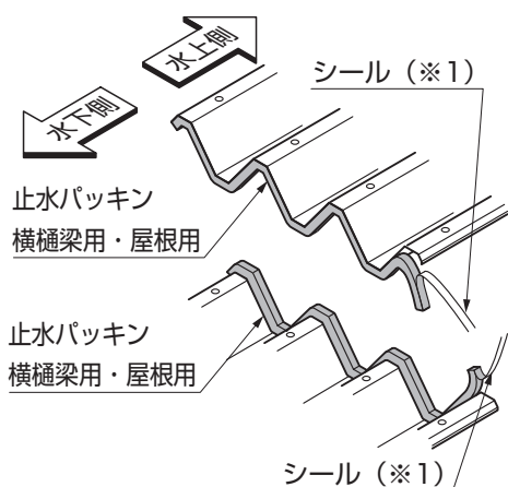
図16-14 止水パッキン 横樋梁用・屋根用の取付け (ポリカ折板屋根材の場合)
