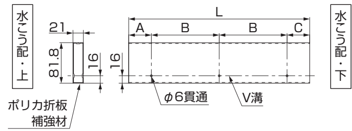
図3-3 梁3本仕様
