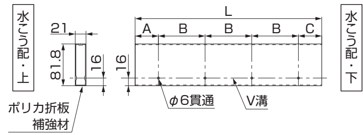
図3-4 梁4本仕様
