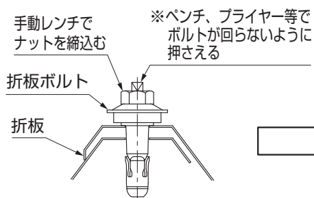
図2-3 折板ボルト取付詳細
