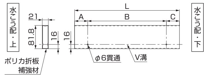
図3-2 梁2本仕様
