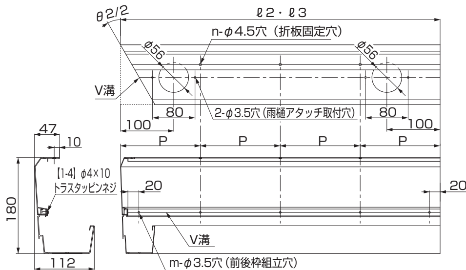
図6-5 前後枠水下
