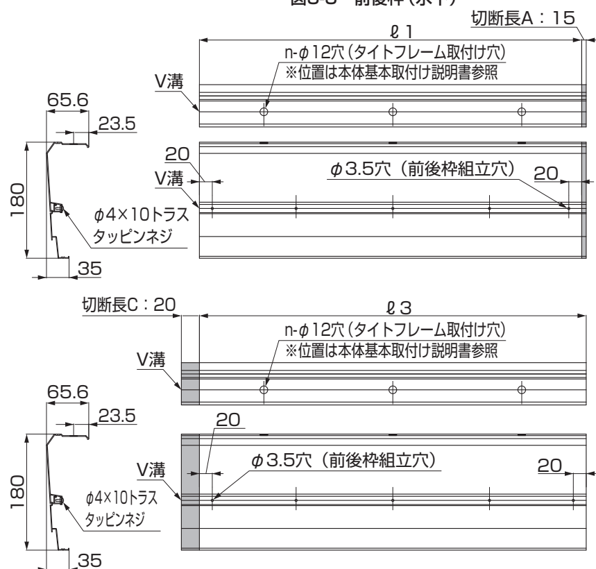
図5-6 側枠
