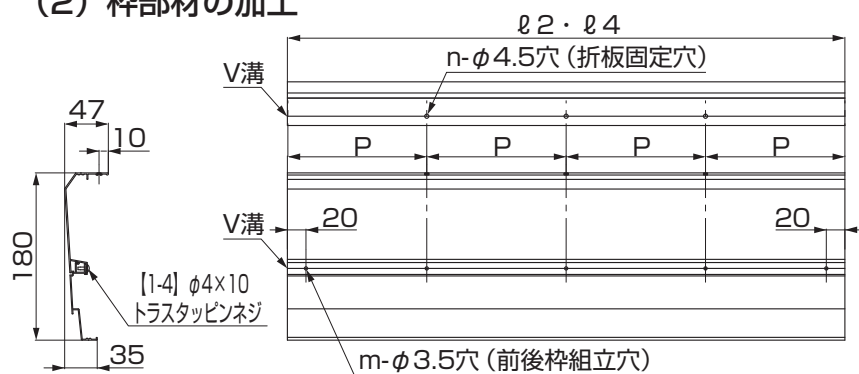
図5-4 前後枠 (水上)
