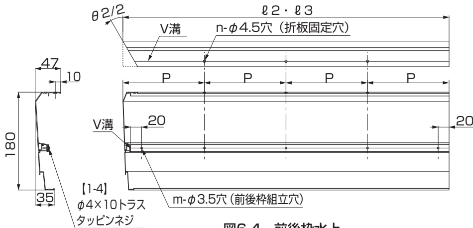
図6-4 前後枠水上
