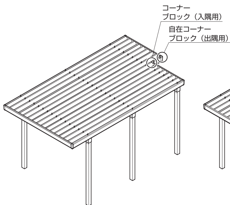
図1-1 出入隅
