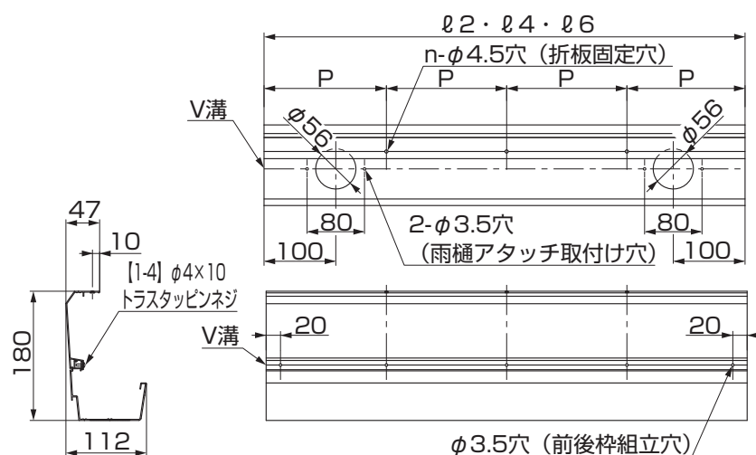
図 4-9 前後枠（水下）
