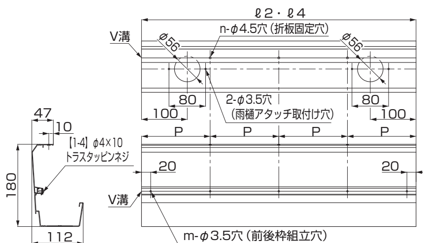
図5-5 前後枠 (水下)
