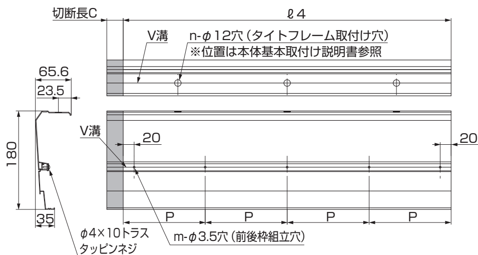
図6-6 側枠
