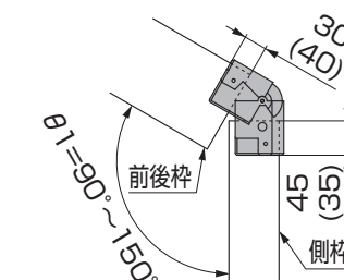
図6-11 前後枠・側枠の差込み寸法
