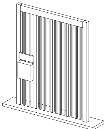
■格子タイプ
