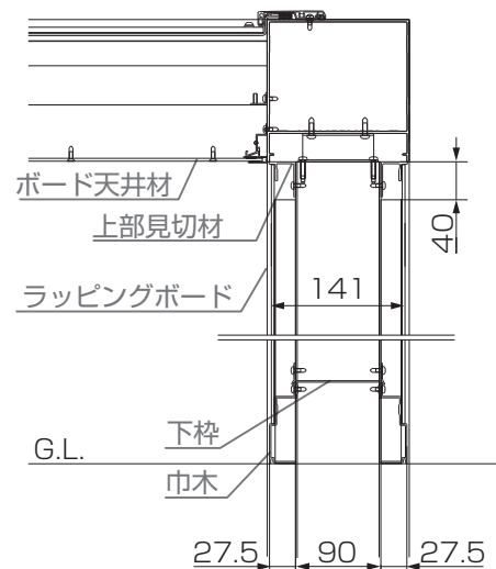
B-B'断面詳細図
