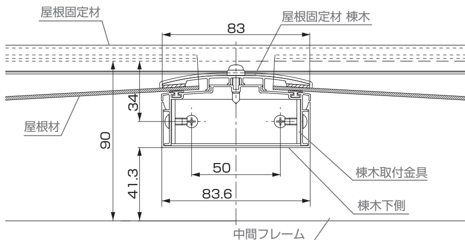
C-C' 断面詳細図
