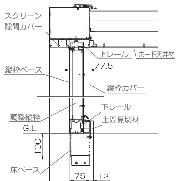
D-D'断面詳細図
