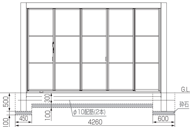
【矢視B (5スパン)】
