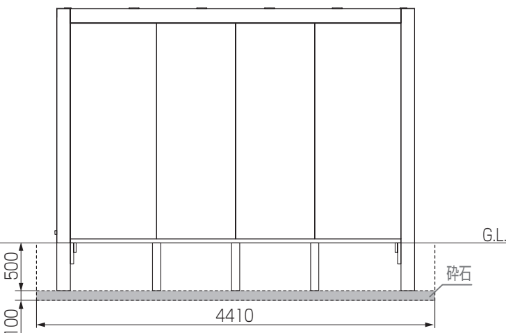
【矢視D (5スパン)】
