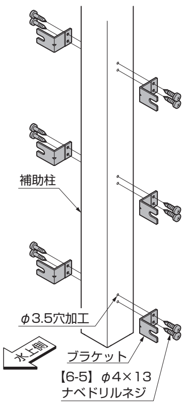
図5-1 幅方向の場合
