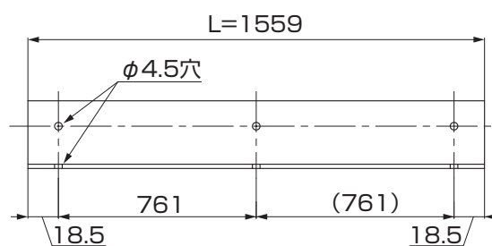
図7-2 標準2段の場合
