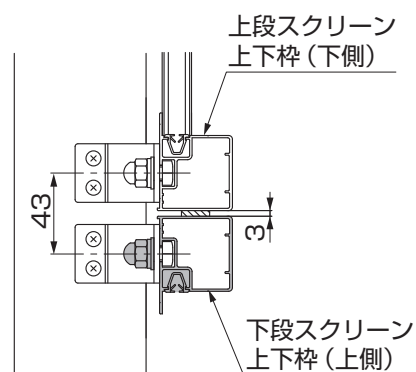
図5-10 角柱・補助柱 (上段スクリーンと接続する場合)
