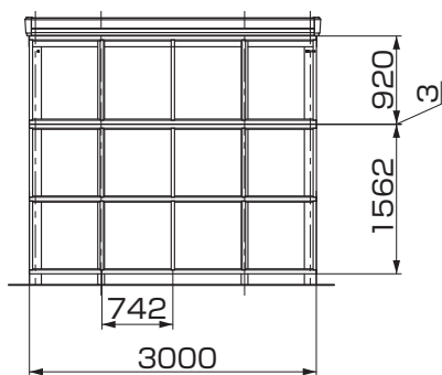
図2-13 1台用 (幅30)
