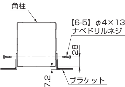
図5-5 角柱（長さ方向）
