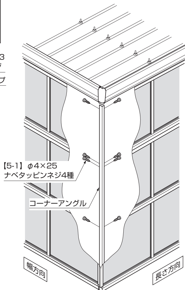
図1-3 コーナー部接続の場合
