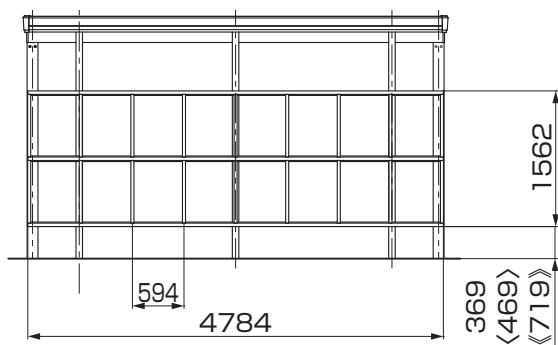
図2-7 2台用 (幅48)
