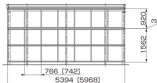
図2-16 2台用 (幅55・60)
