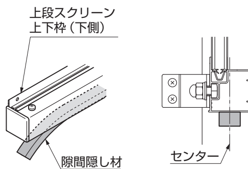
図5-8 上段スクリーンと接続する場合
