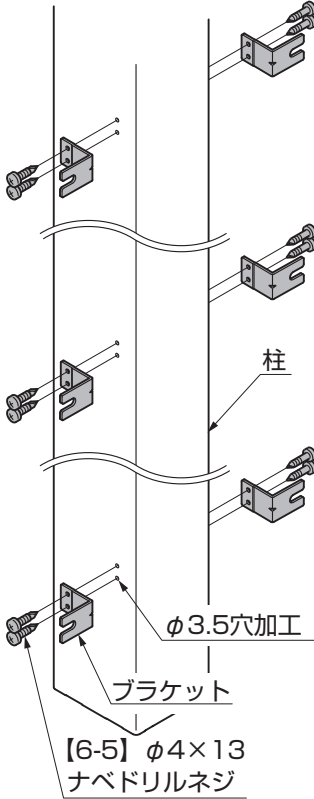
図5-2 長さ方向の場合
