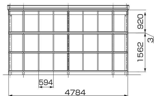
図2-15 2台用 (幅48)
