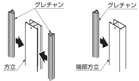
図6-1 グレチャンの取付け
