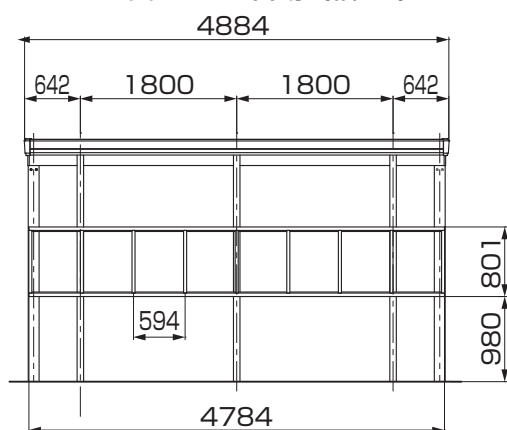
図2-3 2台用 (幅48)
