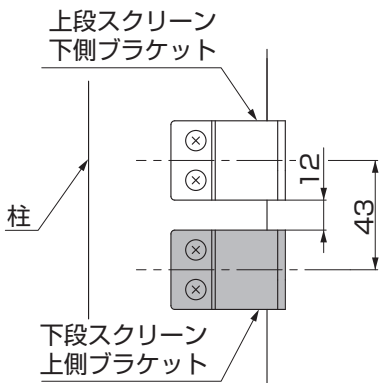
図5-6 上段スクリーンと 接続する場合
