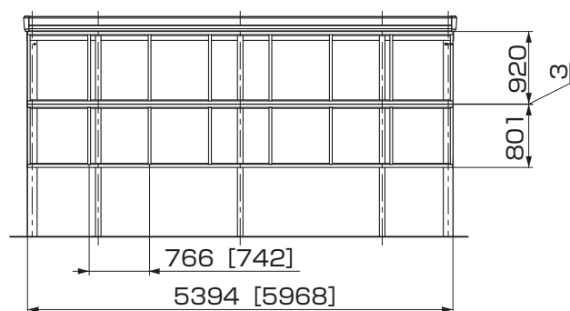
図2-12 2台用 (幅55・60)
