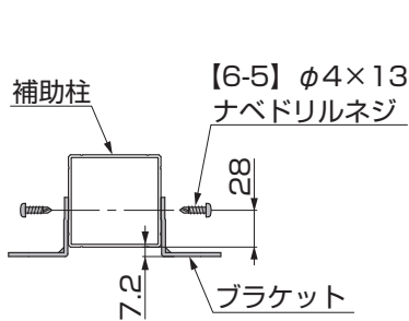
図5-4 補助柱（幅方向）
