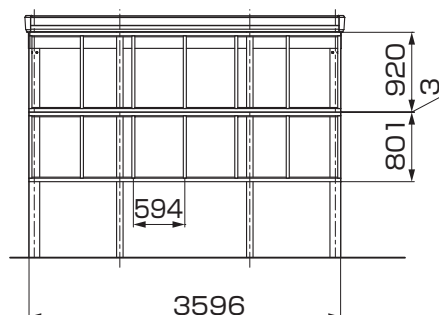
図2-10 1台用 (幅36)
