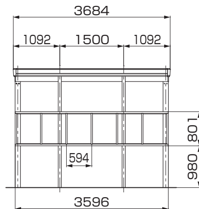
図2-2 1台用 (幅36)
