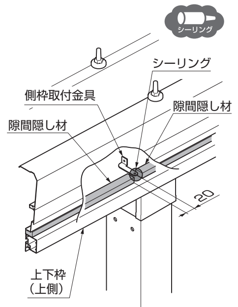
図4-8 側枠取付金具位置の 隙間隠し材の取付け
