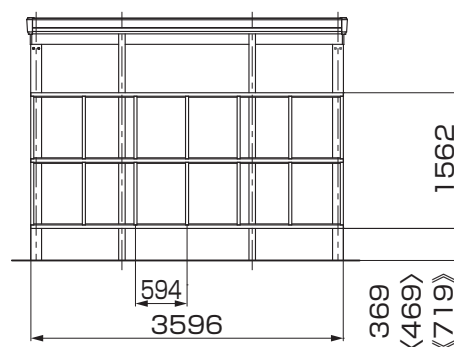
図2-6 1台用 (幅36)
