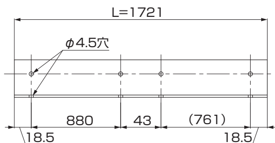
上側 図7-3 上段+標準1段の場合 下側
