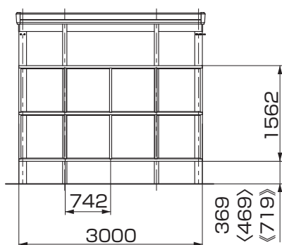
図2-5 1台用 (幅30)
