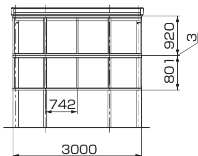
図2-9 1台用 (幅30)
