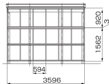
図2-14 1台用 (幅36)
