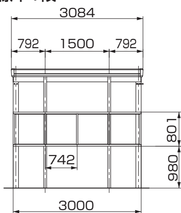
図2-1 1台用 (幅30)
