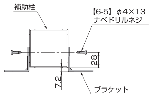
図4-6 補助柱用ブラケット取り付け位置
