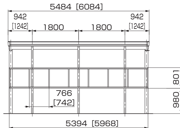
図2-4 2台用 (幅55・60)
