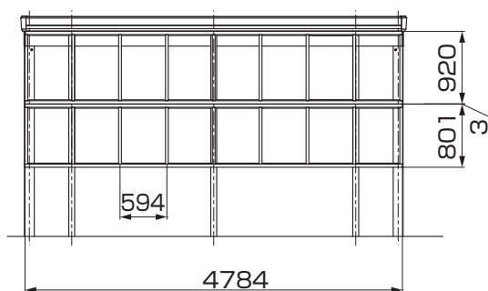
図2-11 2台用 (幅48)
