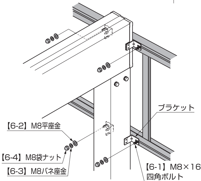
図4-13 上下枠の取付け
