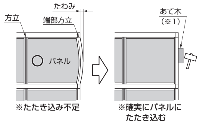
図6-3 パネルのたたき込み
