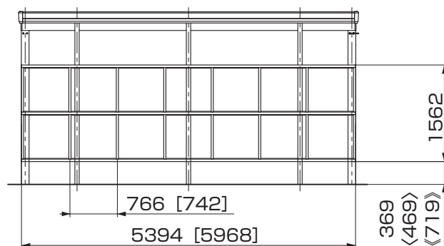
図2-8 2台用 (幅55・60)
